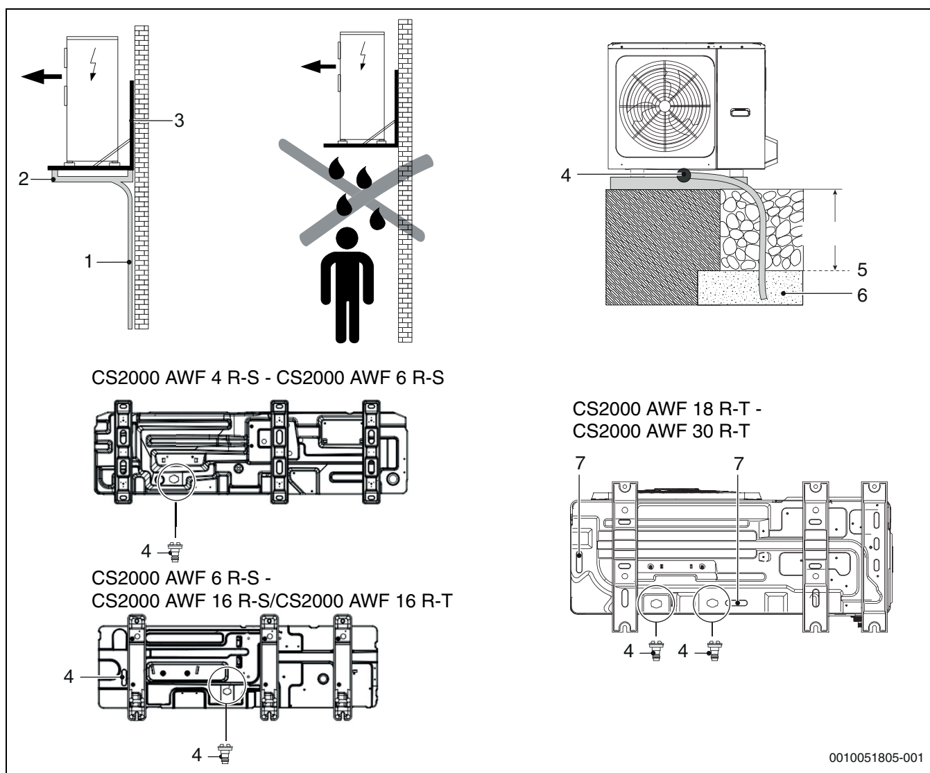
Afb. 49 Condensafvoer
