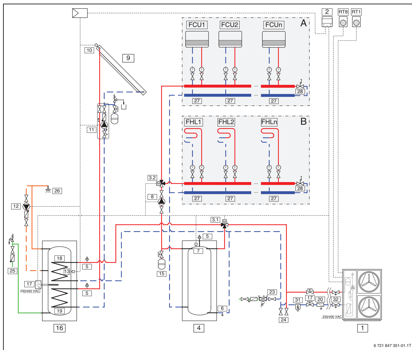
Afb. 21 Buitenunit met één of meerdere cv-groepen, elektrische back-up verwarming, boiler en zonnesysteem (CS2000AWF 18 -30 R-T)
