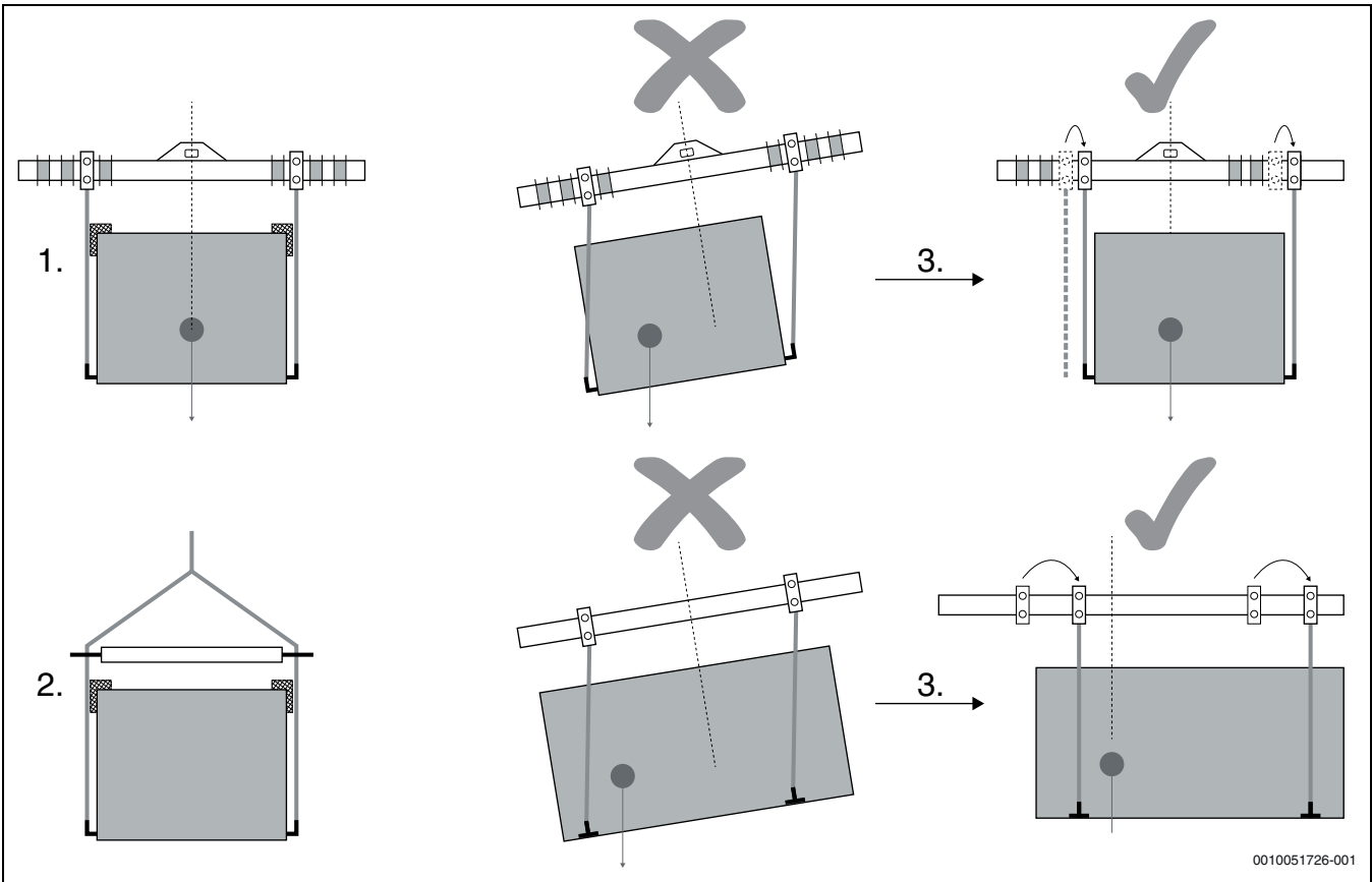
Afb. 29 Hijsen
