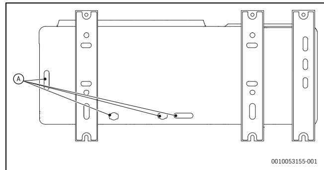
Afb. 47 Afvoeropeningen
