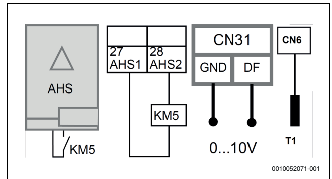
Afb. 92 Extra cv-toestel
