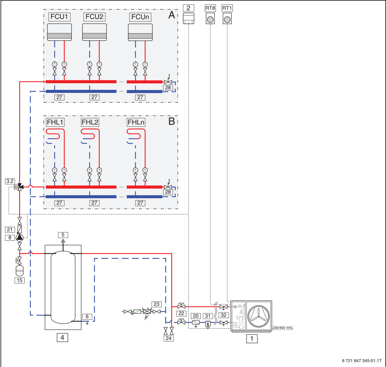
Afb. 17 Buitenunit met één of meerdere cv-groepen, vloerverwarming en ventilatorconvector (CS2000AWF 4-6 R-S, CS2000AWF 8-10 R-S, CS2000AWF 12-16 R-S/T)
