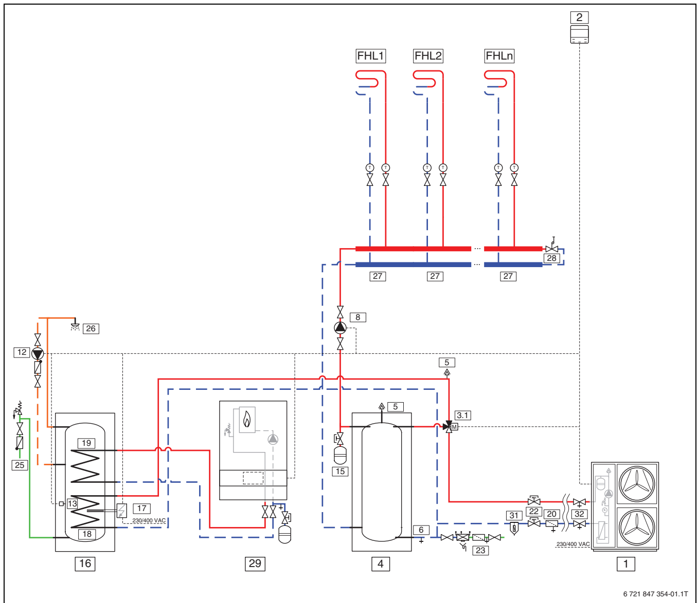
Afb. 24 Buitenunit met één of meerdere cv-groepen, externe bijverwarming en boiler (CS2000AWF 18 -30 R-T)
