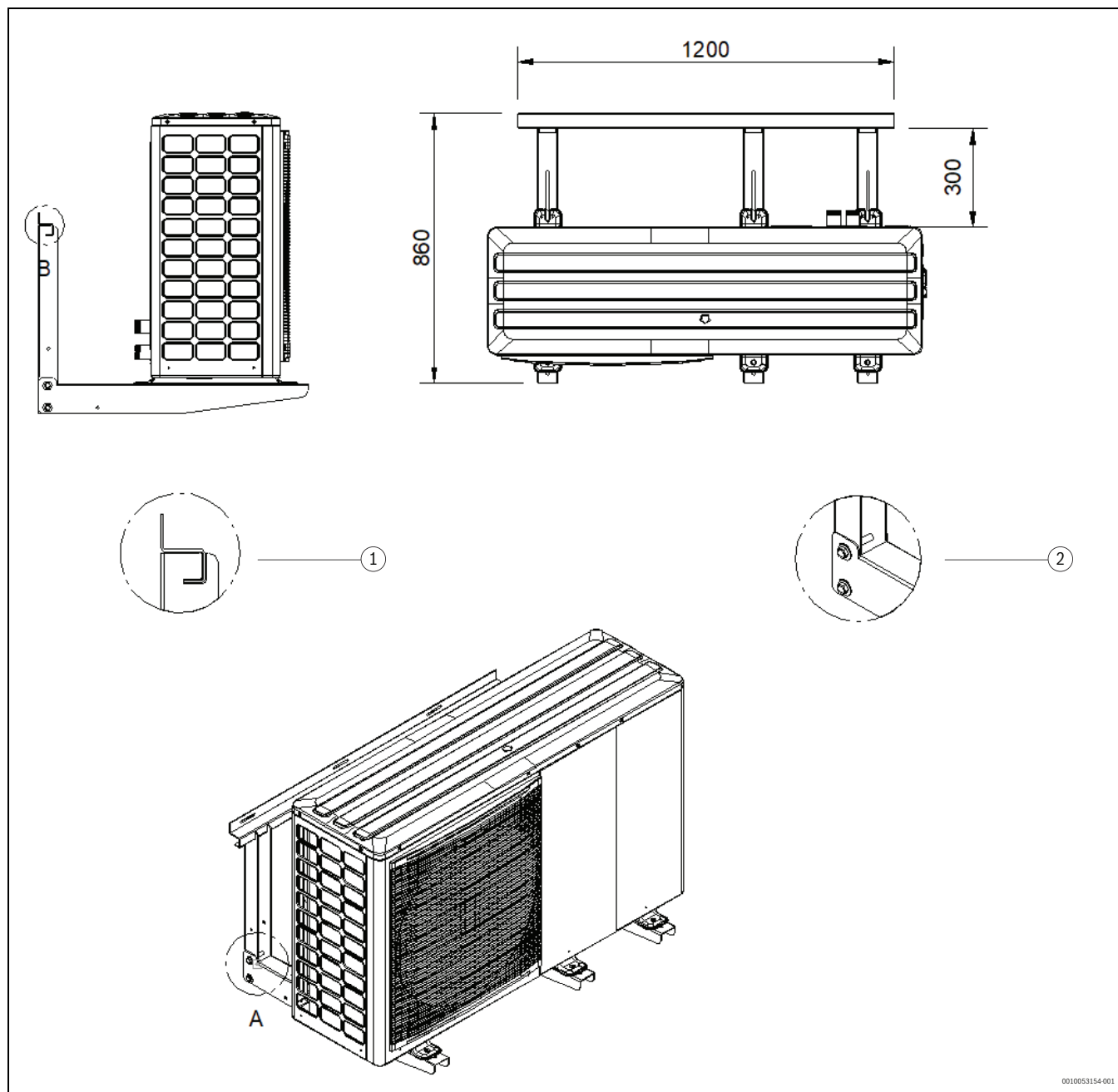
Afb. 44 Wandmontage
