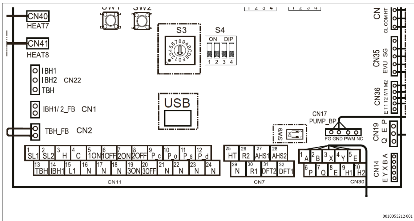
Afb. 73 Klemmenblok aansluiten
