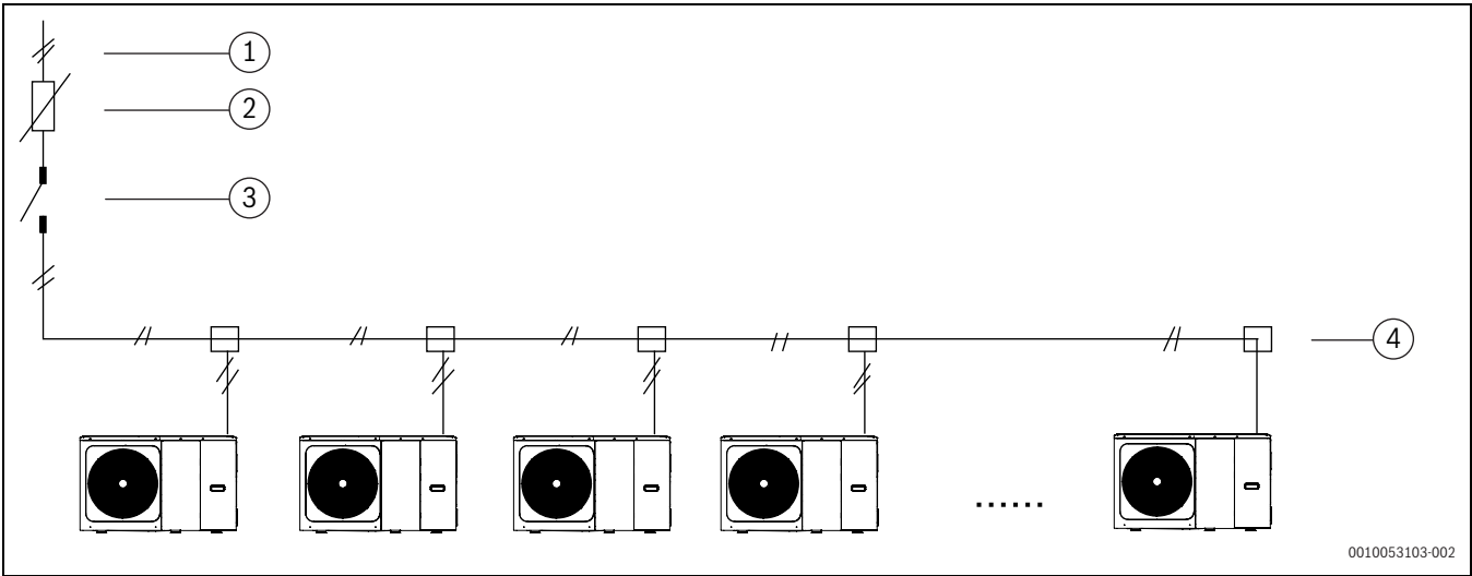
Afb. 71 Elektrisch circuit
