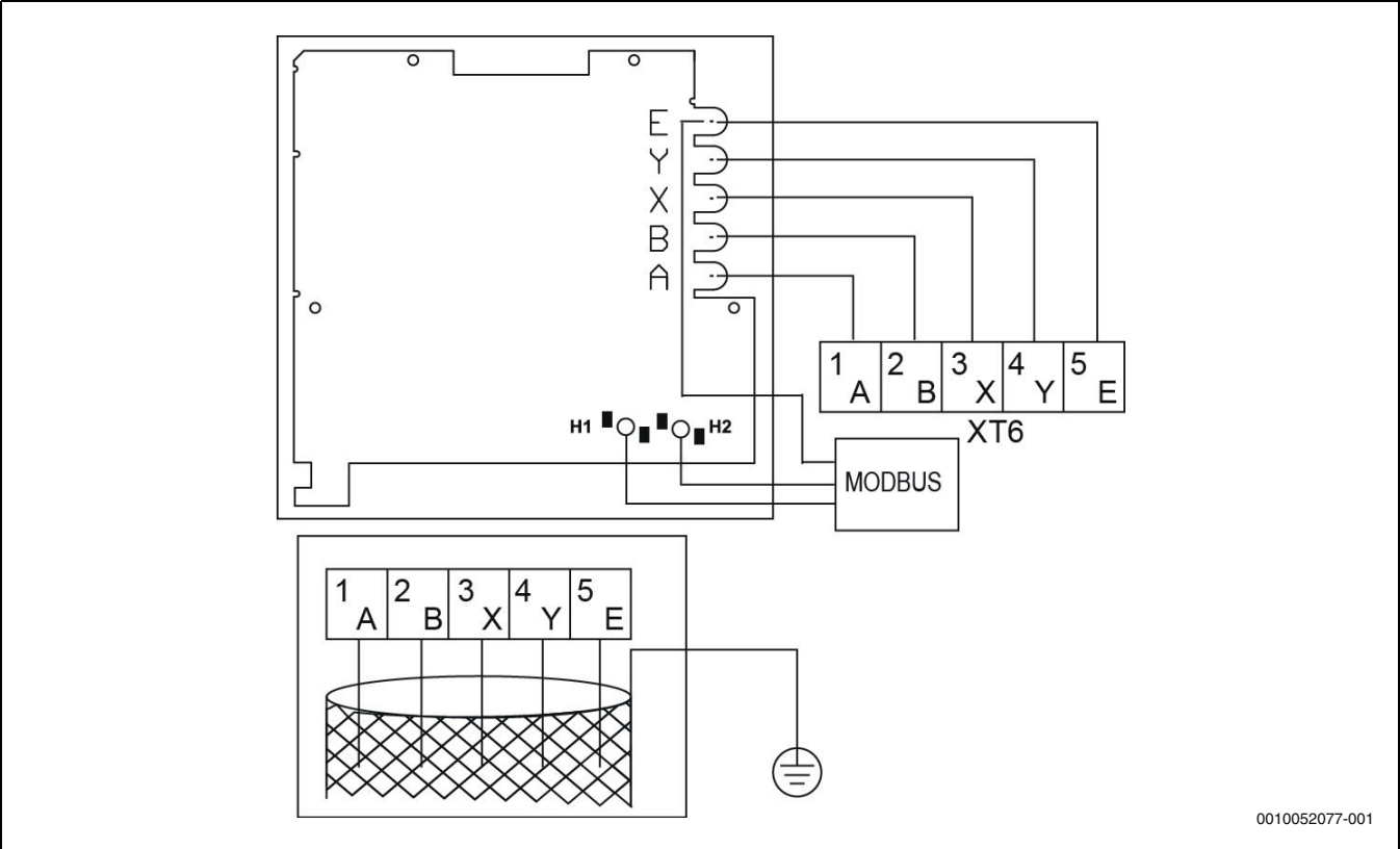
Afb. 94 Bedieningsunit
