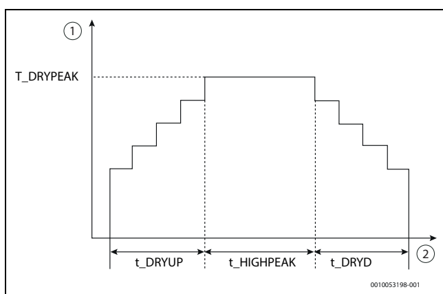
Afb. 143 Diagram droogcyclus
