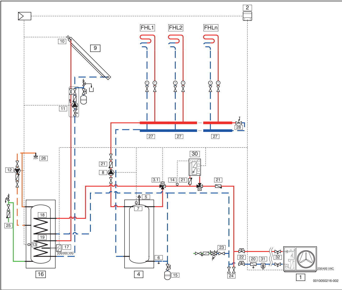
Afb. 15 Buitenunit met één of meerdere cv-groepen, elektrische back-up verwarming, boiler en zonnestelsysteem (CS2000AWF 4-6 R-S, CS2000AWF 8-10 R-S, CS2000AWF 12-16 R-S/T)
