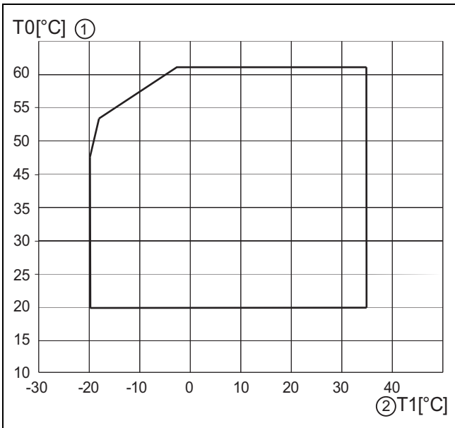
Afb. 20 Buitenunit zonder bijverwarming
