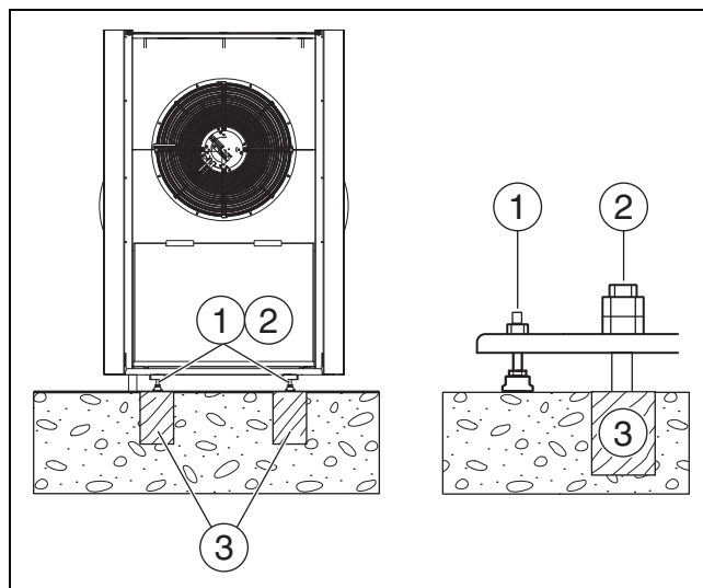
Afb. 11 Bevestigen van de warmtepomp
