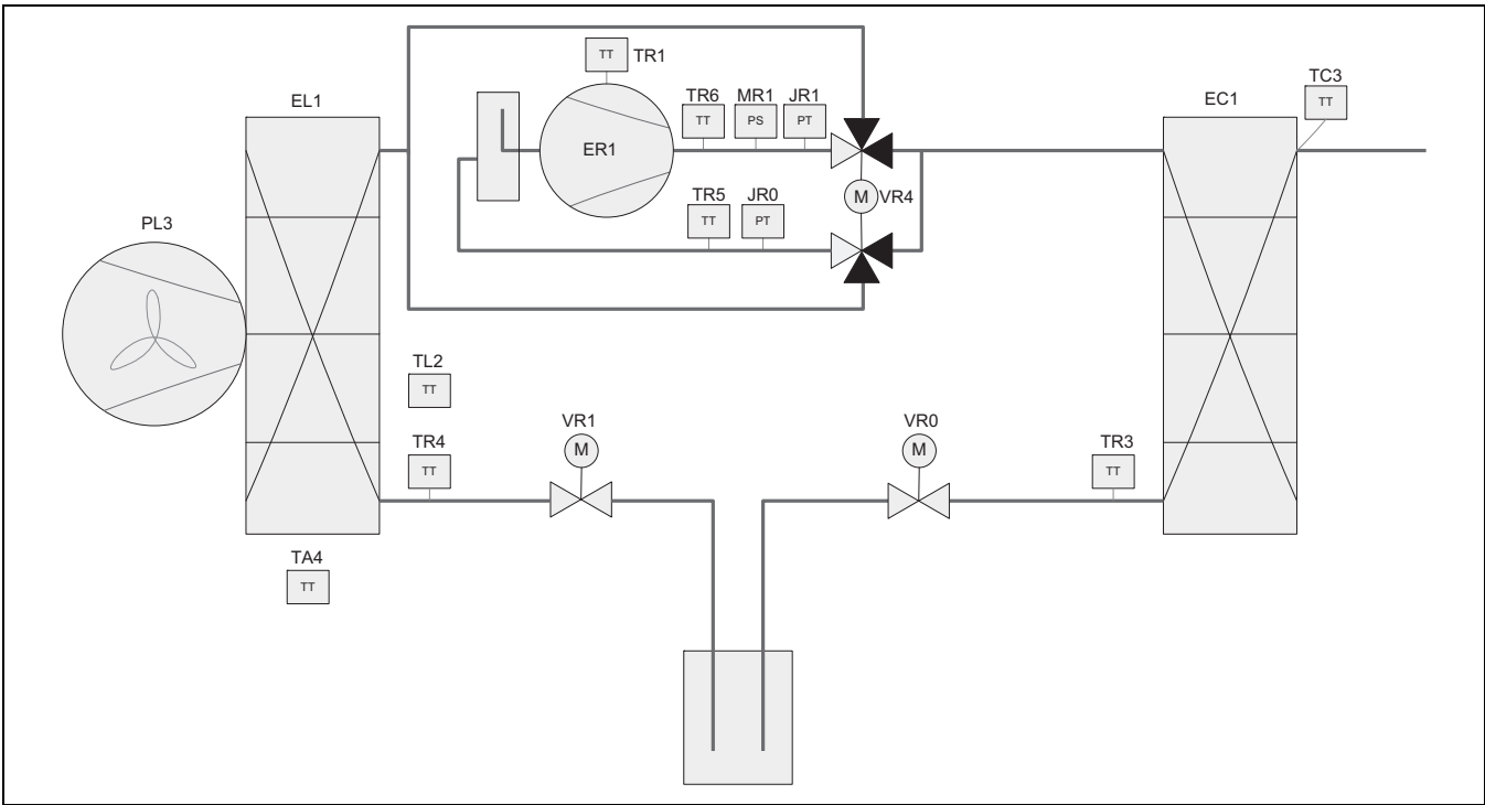
Afb. 21 Koudemiddelcircuit
