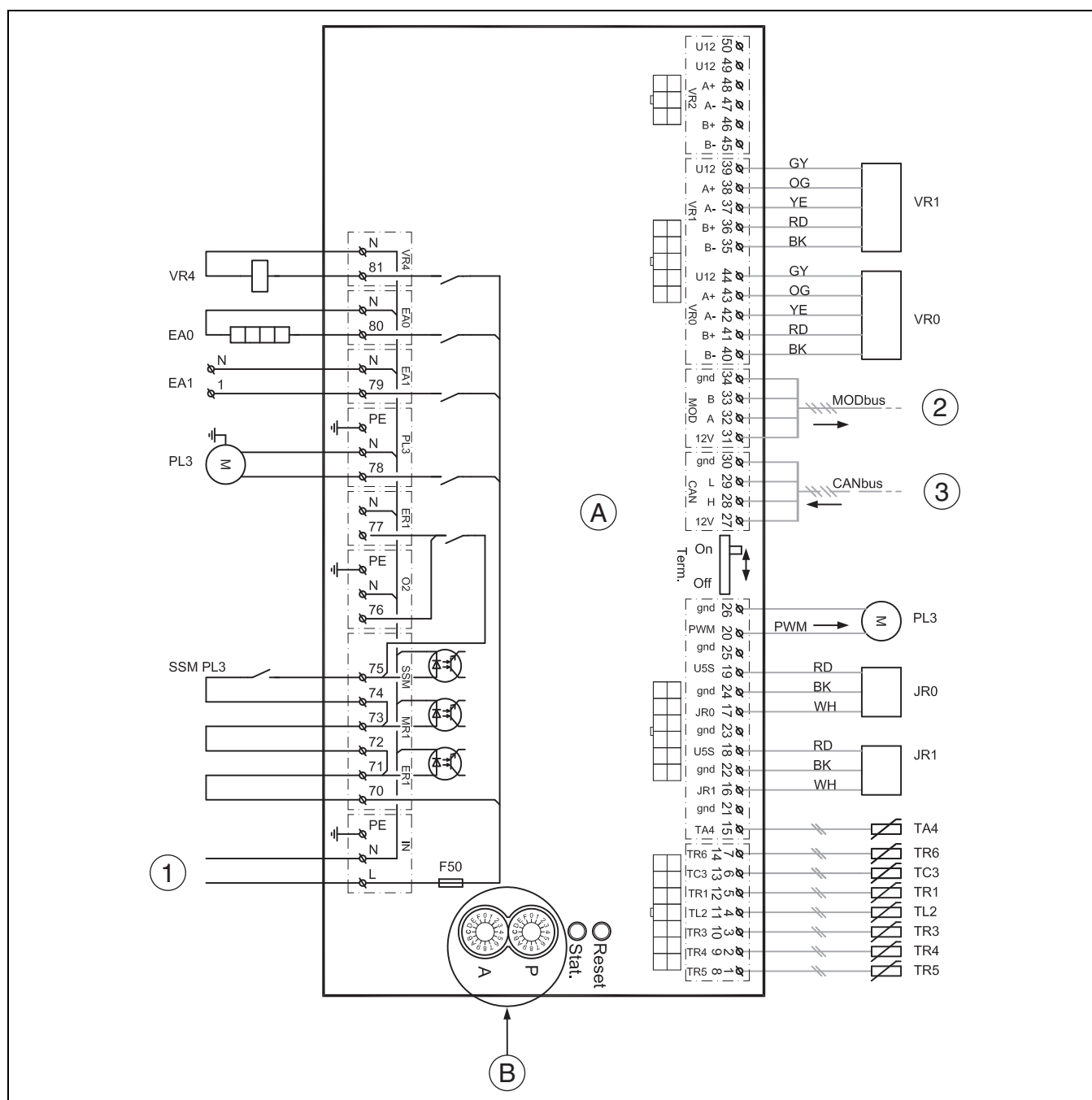
Afb. 22 Elektrische schema voor I/O-module
