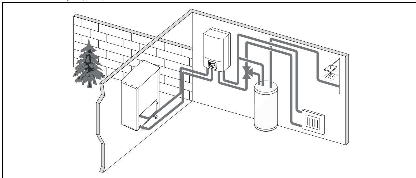
Fig. 3 Pompe à chaleur Compress 7000 AW, unité intérieure AWE avec chauffage d'appoint électrique et ballon d'eau chaude sanitaire externe
