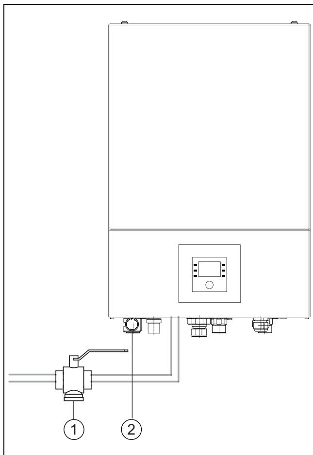
Afb. 6 Binneneenheid AWE
