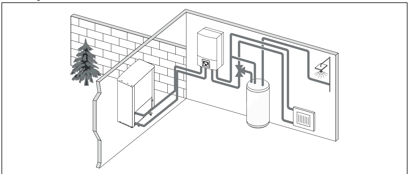
Afb. 3 Warmtepomp Compress 7000 AW, binneneenheid AWE met elektrische bijverwarming en externe warmwaterboiler
