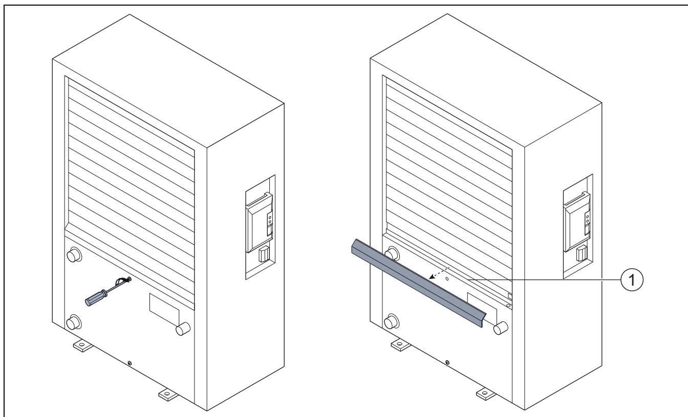
Afb. 8 Condensbak van de warmtepomp
