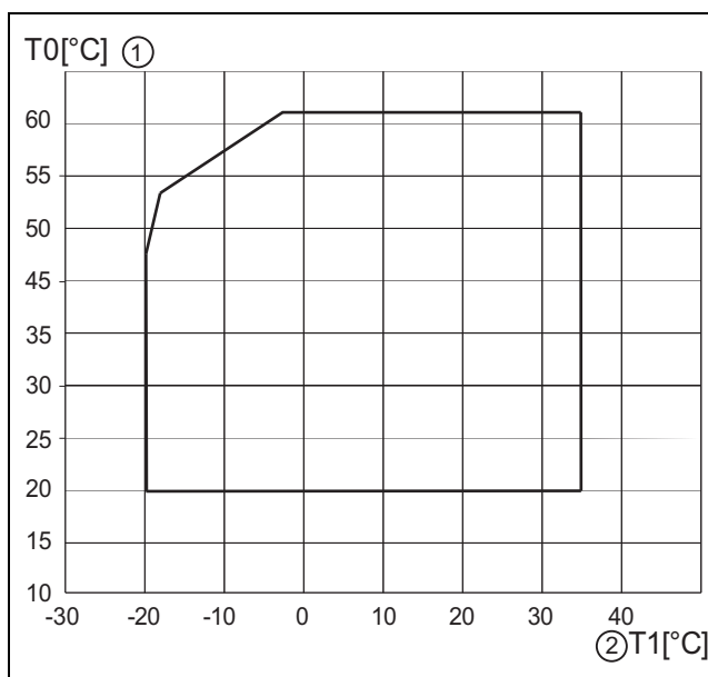
Afb. 1 Warmtepomp zonder bijverwarming
