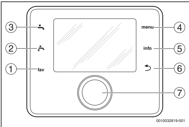
Afb. 4 Bedieningselementen
