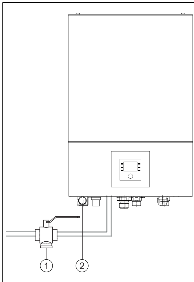
Afb. 6 Binneneenheid AWB
