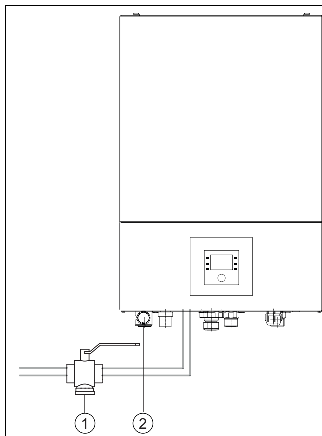
Fig. 6 Unité intérieure AWB
