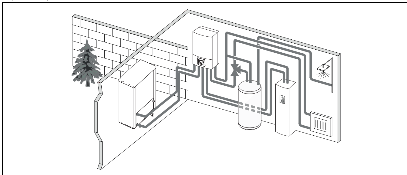
Fig. 3 Pompe à chaleur Compress 6000 AW, unité intérieure AWB sans chauffage d'appoint électrique, ballon d'eau chaude sanitaire externe et chauffage d'appoint externe
