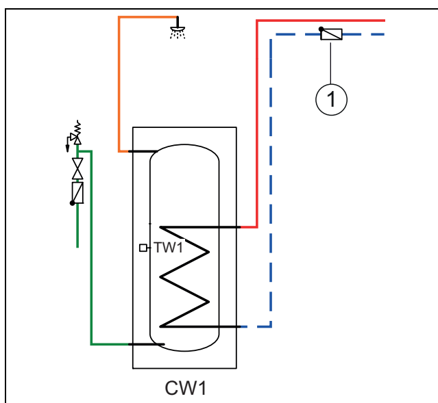
Fig. 22 Ballon d'eau chaude sanitaire
