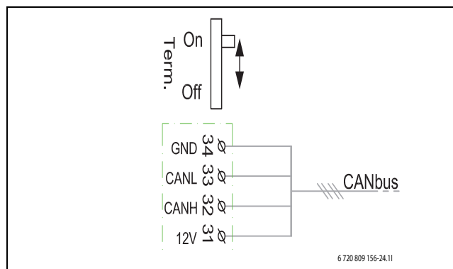
Fig. 8 Terminaison CAN-BUS
