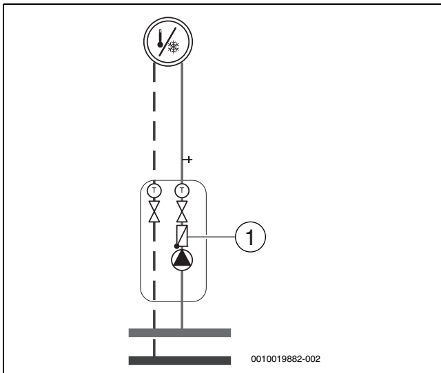
Fig. 30 Circuit de chauffage
