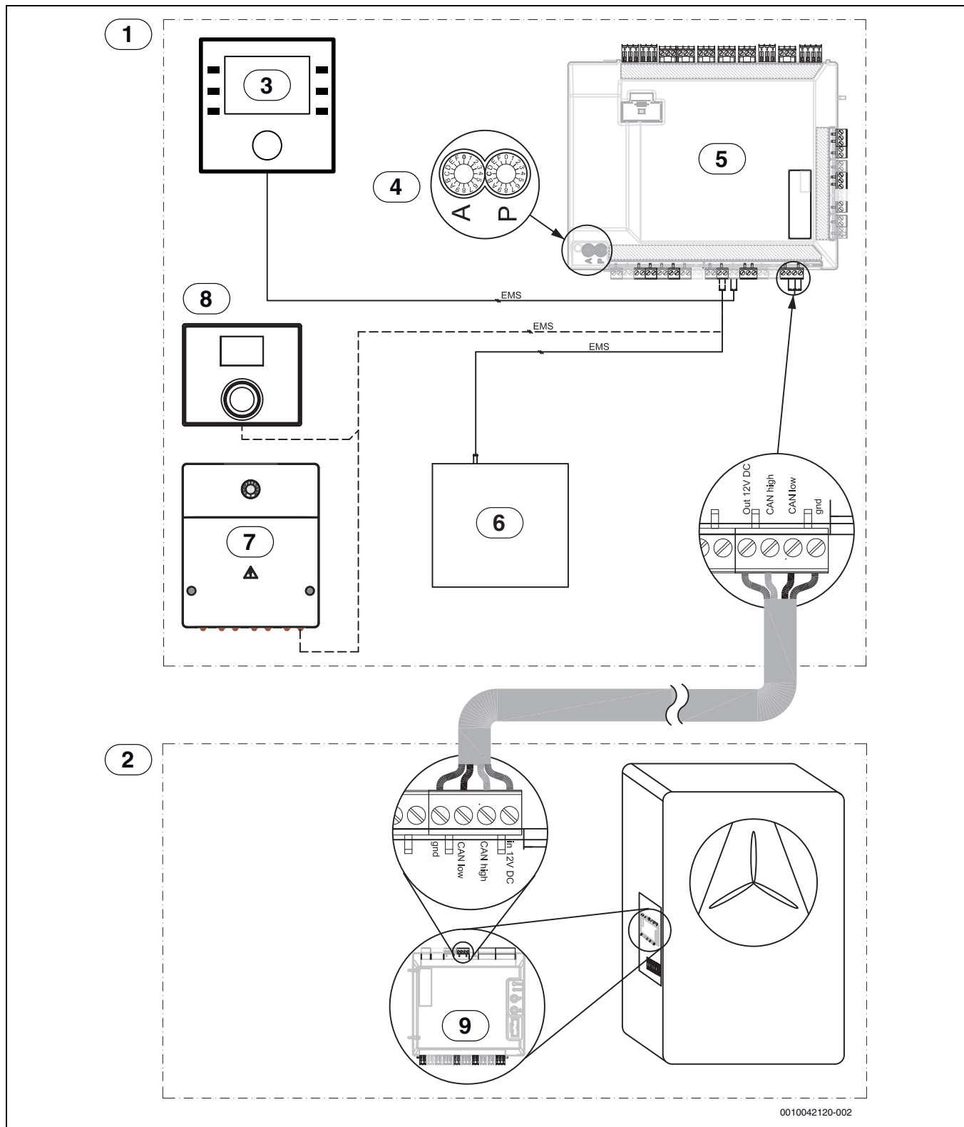
Fig. 32 CAN-BUS/EMS-BUS pour unité intérieure avec chauffage d'appoint électrique – aperçu
