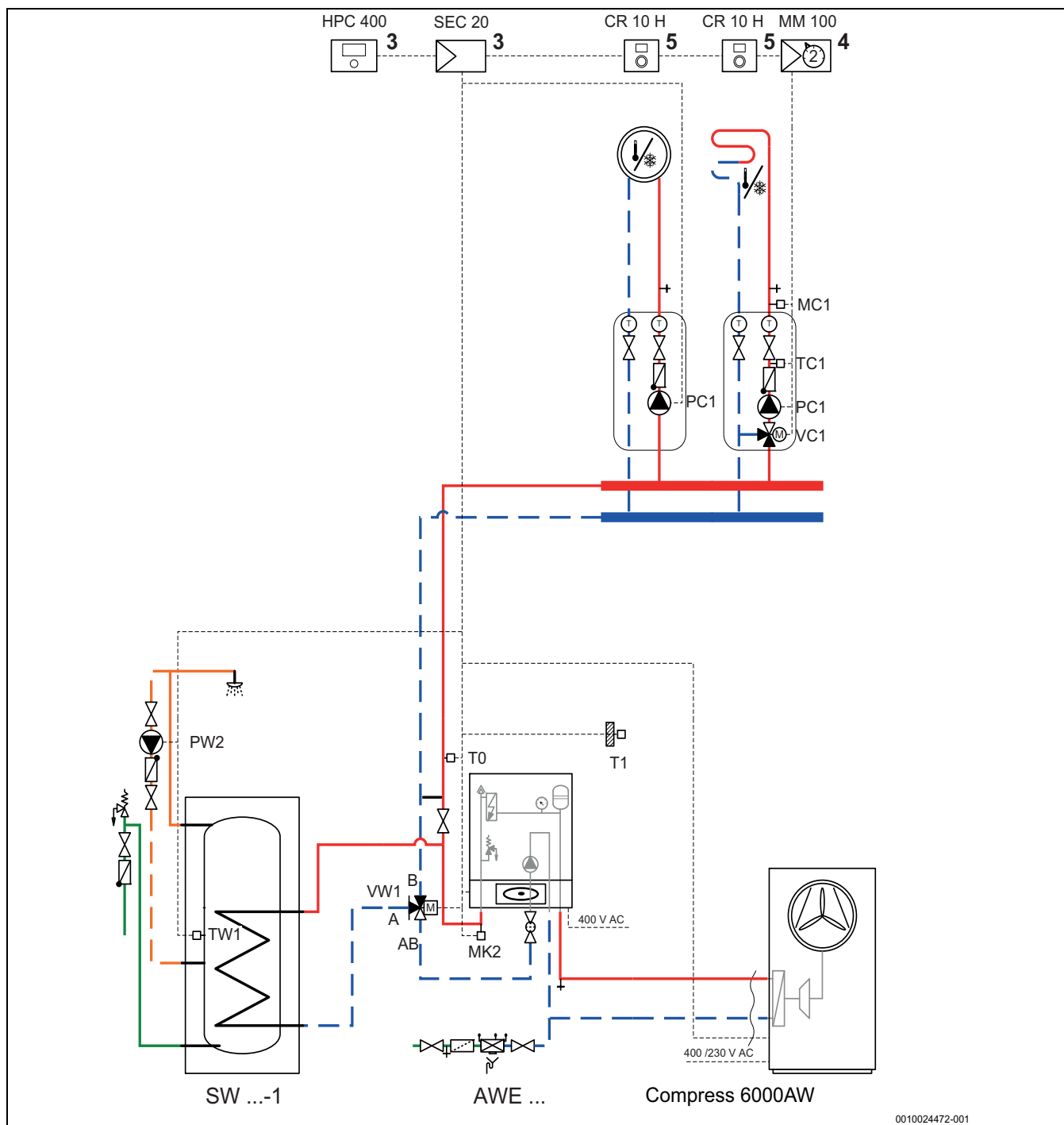
Fig. 31 Chauffage d'appoint électrique avec préparateur d'eau chaude sanitaire
