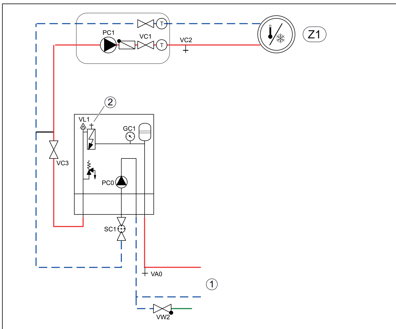
Fig. 19 Unité intérieure avec chauffage d'appoint électrique intégré et système de chauffage
