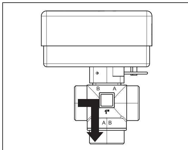
Fig. 25 Contact ouvert, raccordement B ouvert
