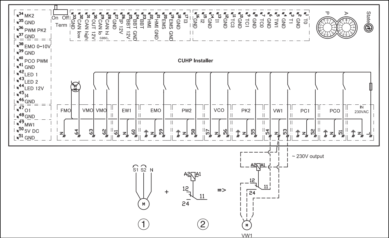
Fig. 36 Alternative d'installation de la vanne sélective
