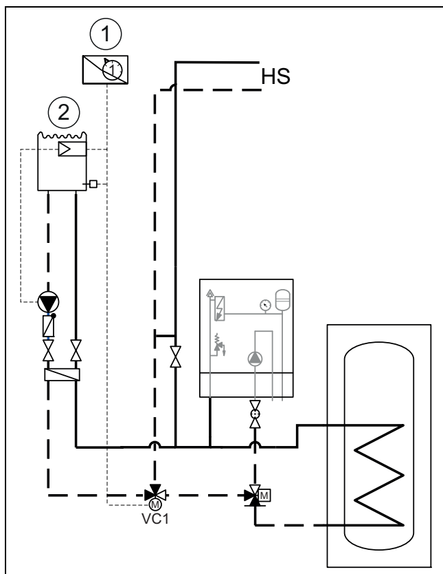
Fig. 27 Exemple d'installation de piscine
