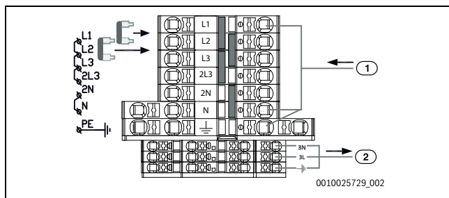
Fig. 12 Exécution alternative
