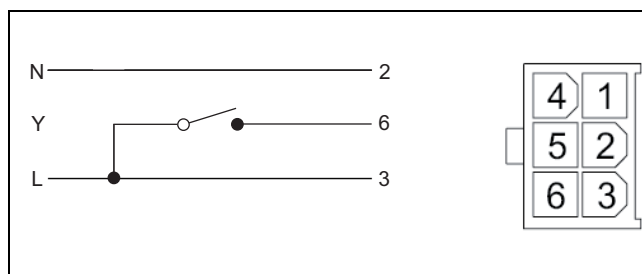
Fig. 26 Connecteur Molex
