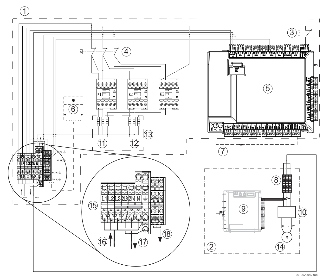
Fig. 33 Pompe à chaleur monphasée avec chauffage d'appoint électrique intégré (courant triphasé)
