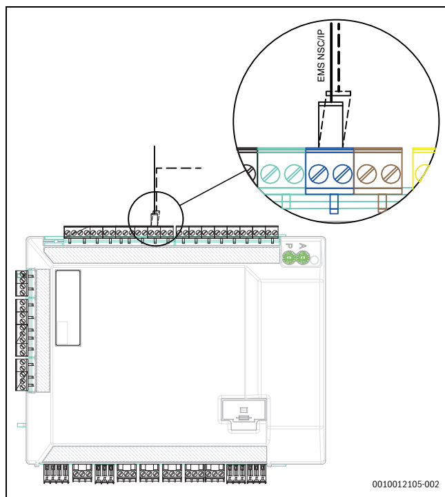
Fig. 21 Raccordement EMS sur le module d'installation
