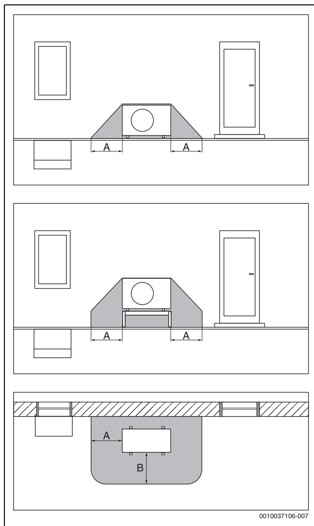
Afb. 1 Veiligheidszone vloermontage
