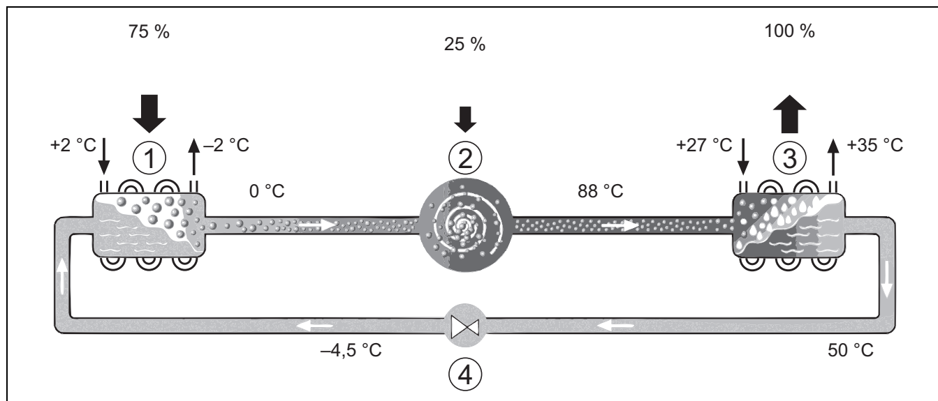
Afb. 6 Weringsprincipe van het koelmiddelcircuit in de warmtepomp
