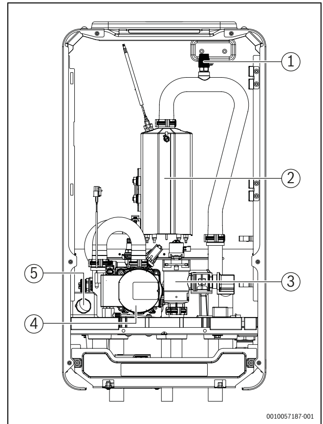
Afb. 5 Componenten
