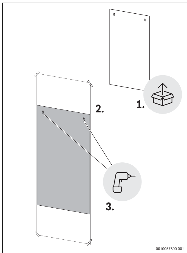
Afb. 9 Boorsjabloon
