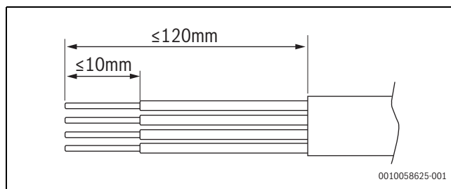
Afb. 49 Strippen CAN-BUS
