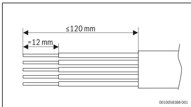
Afb. 38 Striplengte ader voedingsaansluiting
