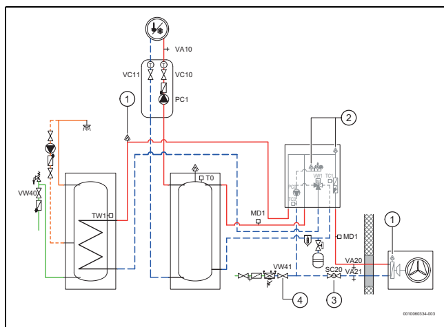
Afb. 37 Binneneenheid, buiteneenheid, boiler en een verwarmingssysteem
