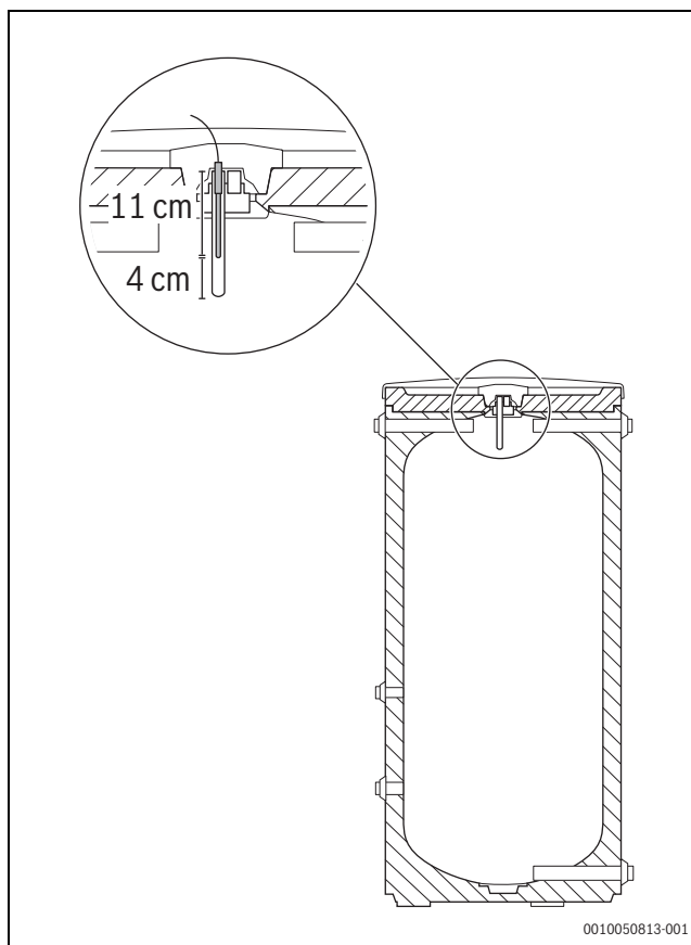
Afb. 52 Aanvoertemperatuursensor T0 plaatsen
