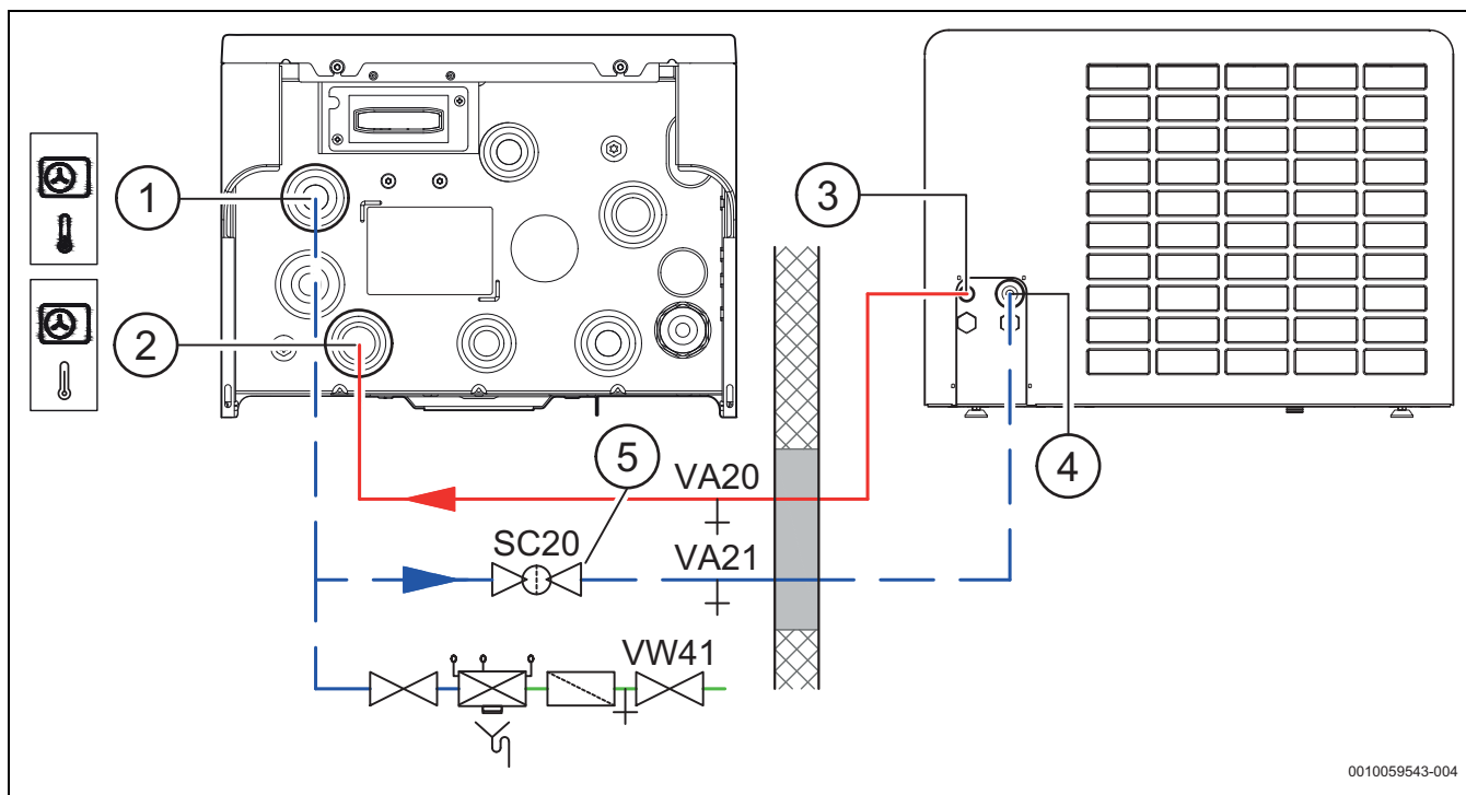
Afb. 23 Aansluiten van de binneneenheid op de buiteneenheid
