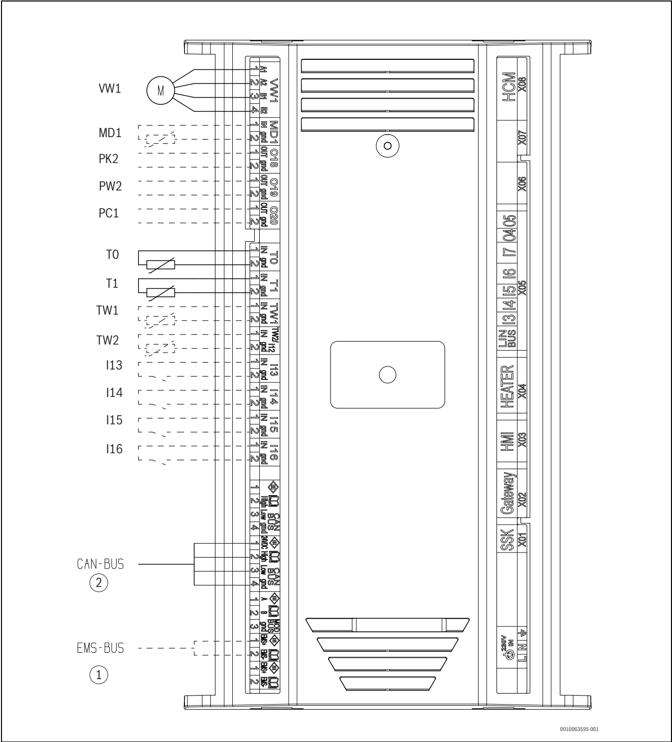
Afb. 46 Aansluitingen XCU-THH
