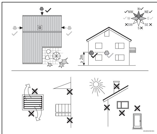
Afb. 51 Positie van de buitentemperatuursensor
