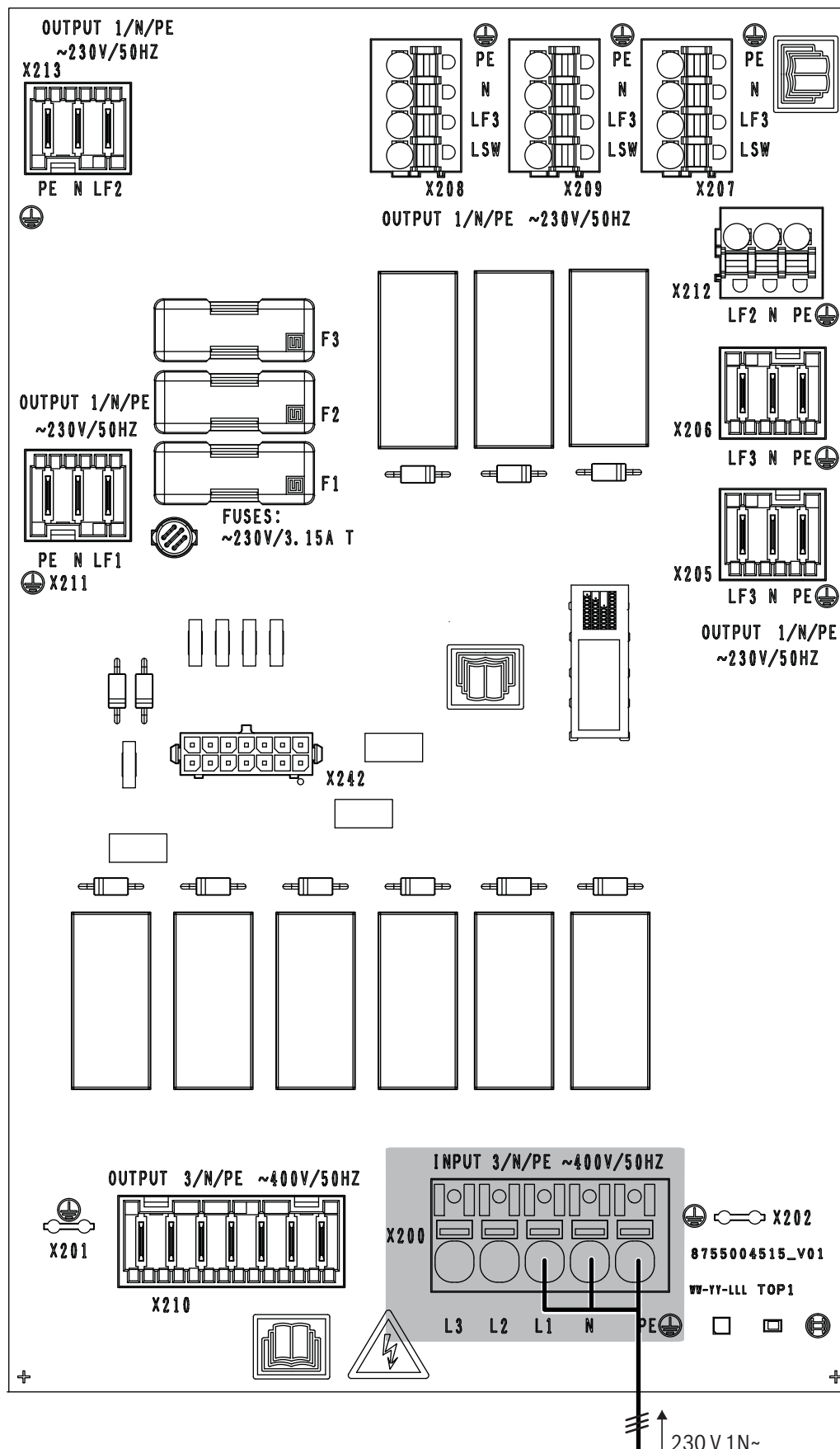
Afb. 45 230 V aansluiting voor binneneenheid
