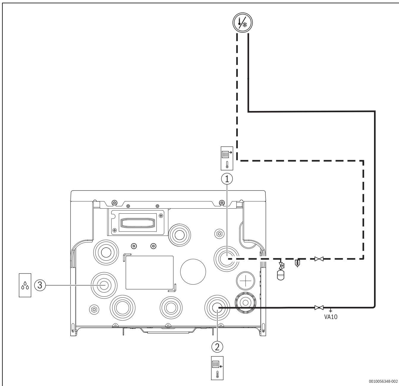
Afb. 22 Aansluiting van de binneneenheid op het verwarmingssysteem
