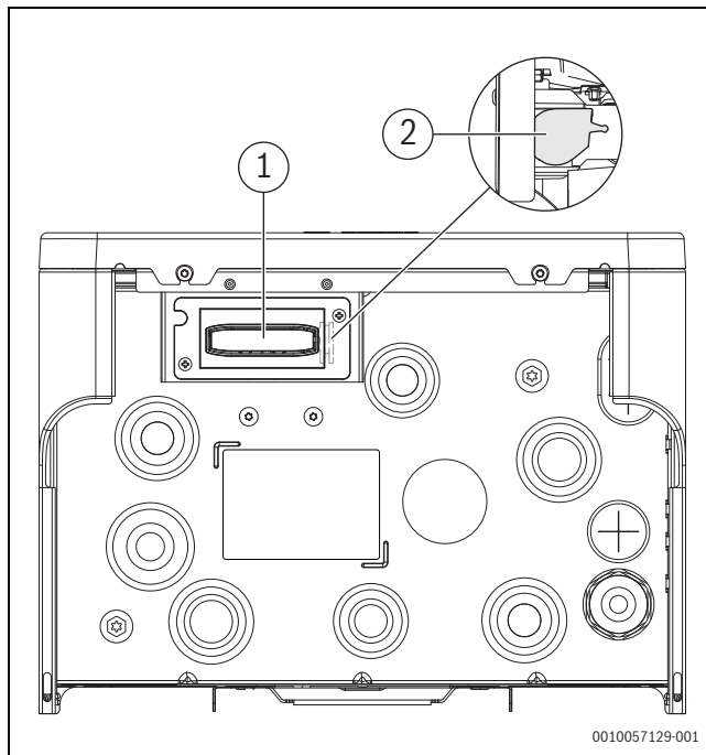
Afb. 14 Connect-Key plaatsen
