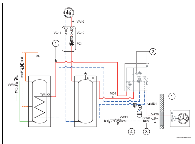
Afb. 35 Binneneenheid, buiteneenheid, boiler en een verwarmingssysteem
