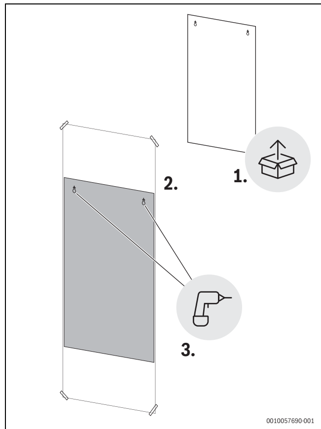
Afb. 9 Boorsjabloon
