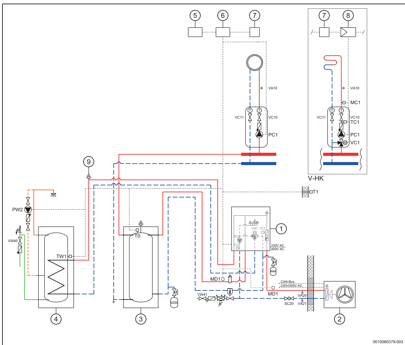
Afb. 56 Buiteneenheid, binneneenheid, buffervat en boiler
