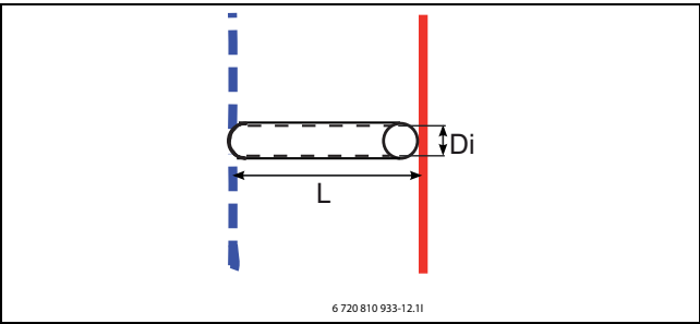
Afb. 27 Gedetailleerd overzicht van bypass
