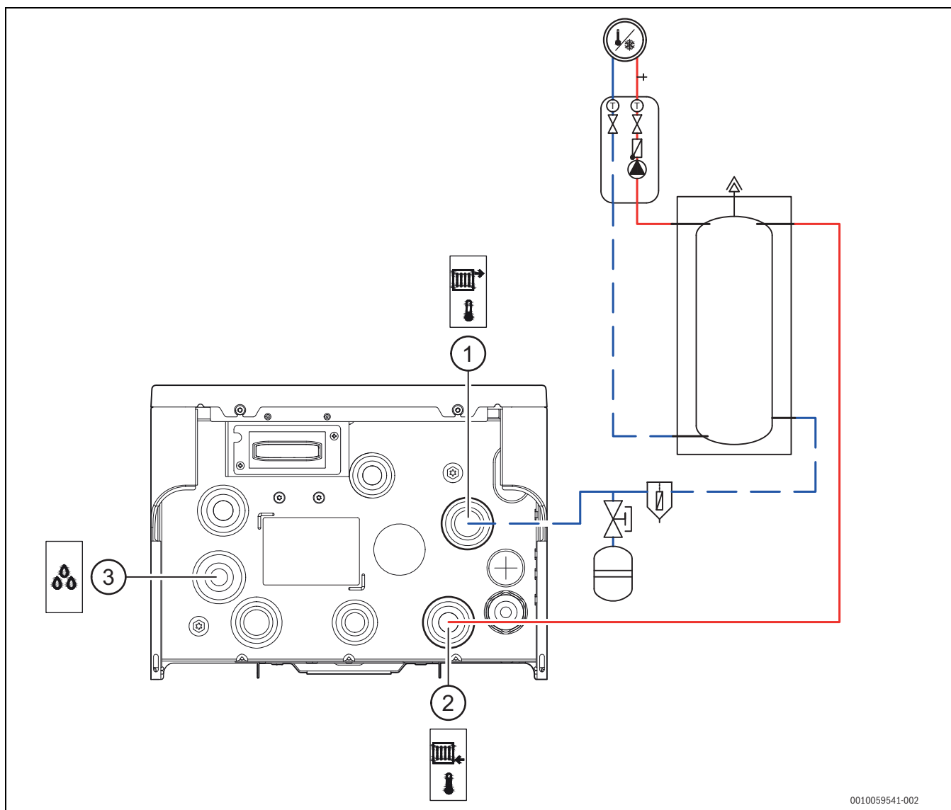
Afb. 26 Aansluiting van de binneneenheid op het verwarmingssysteem
