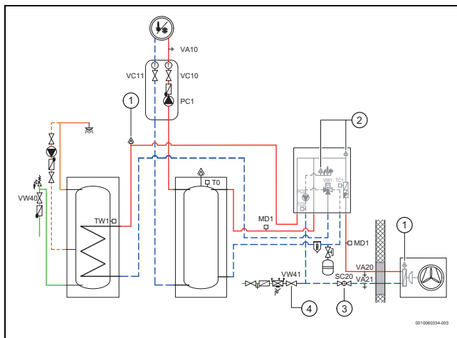
Afb. 30 Binneneenheid, buiteneenheid, boiler en een verwarmingssysteem
