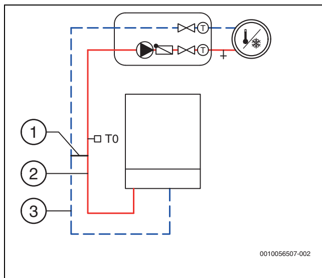
Afb. 36 Cv-circuit met bypass
