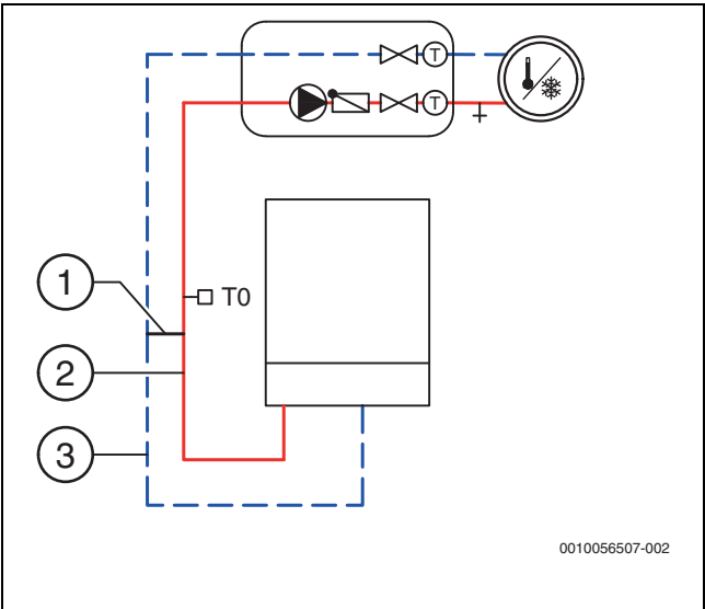
Afb. 29 Cv-circuit met bypass
