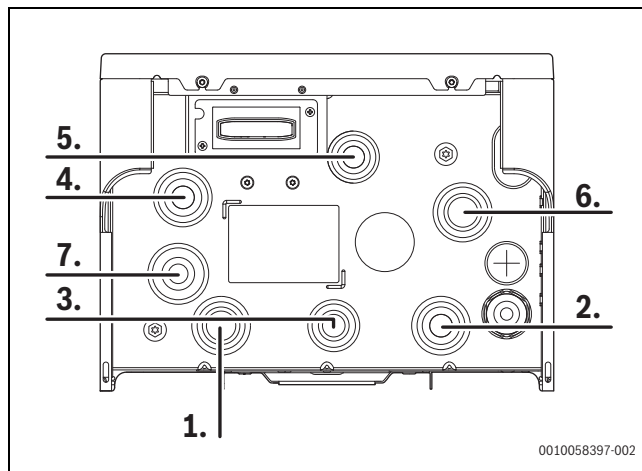
Afb. 17 Aanbevolen volgorde voor de leidingaansluitingen
