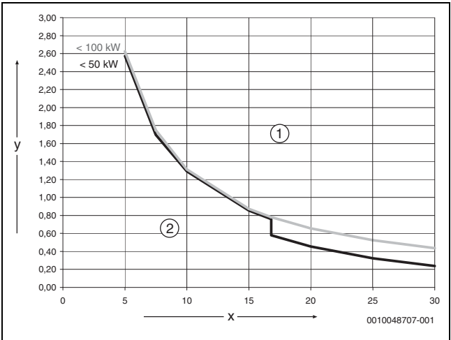
Afb. 8 Warmteproducenten < 50 kW-100 kW
