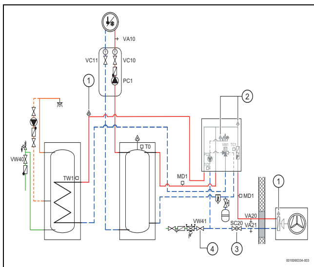
Afb. 23 Binneneenheid, buiteneenheid, boiler en een verwarmingssysteem
