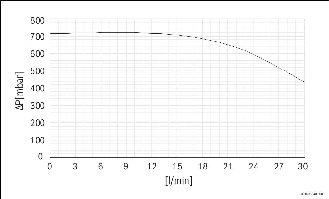
Afb. 57 Prestatieoverzicht voor PC0
