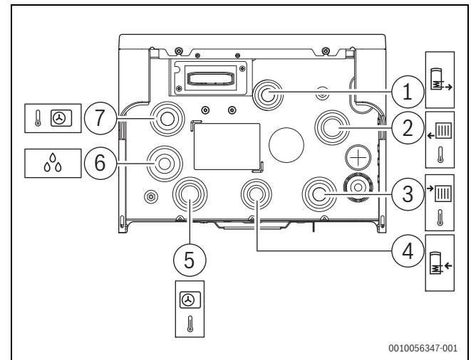
Afb. 6 Leidingaansluitingen
