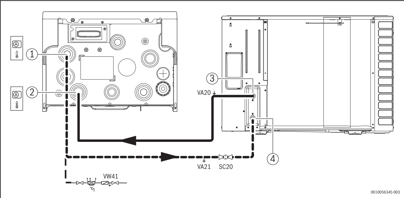
Afb. 21 Aansluiten van de binneneenheid op de buiteneenheid
