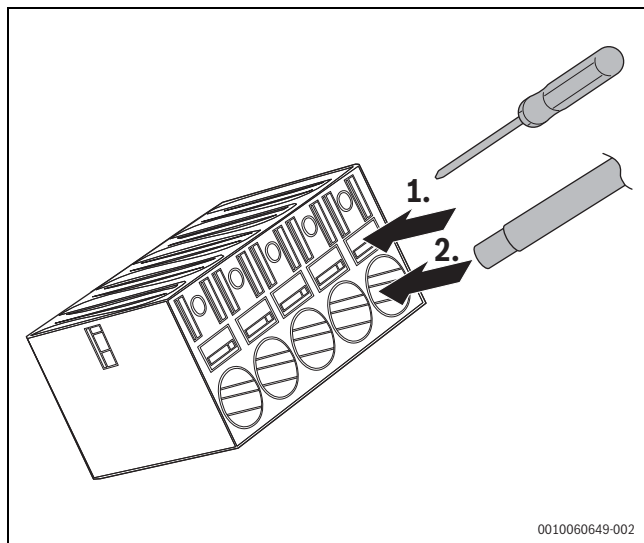
Afb. 42 Kabelinstallatie
