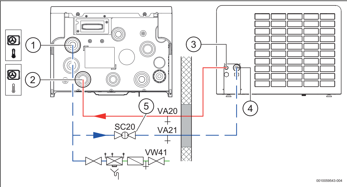
Afb. 25 Aansluiten van de binneneenheid op de buiteneenheid
