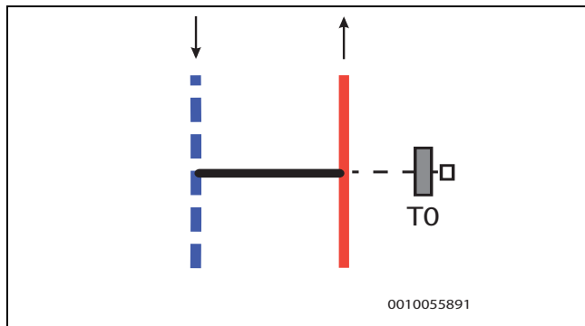
Afb. 26 Bypass, in rechte uitvoering
