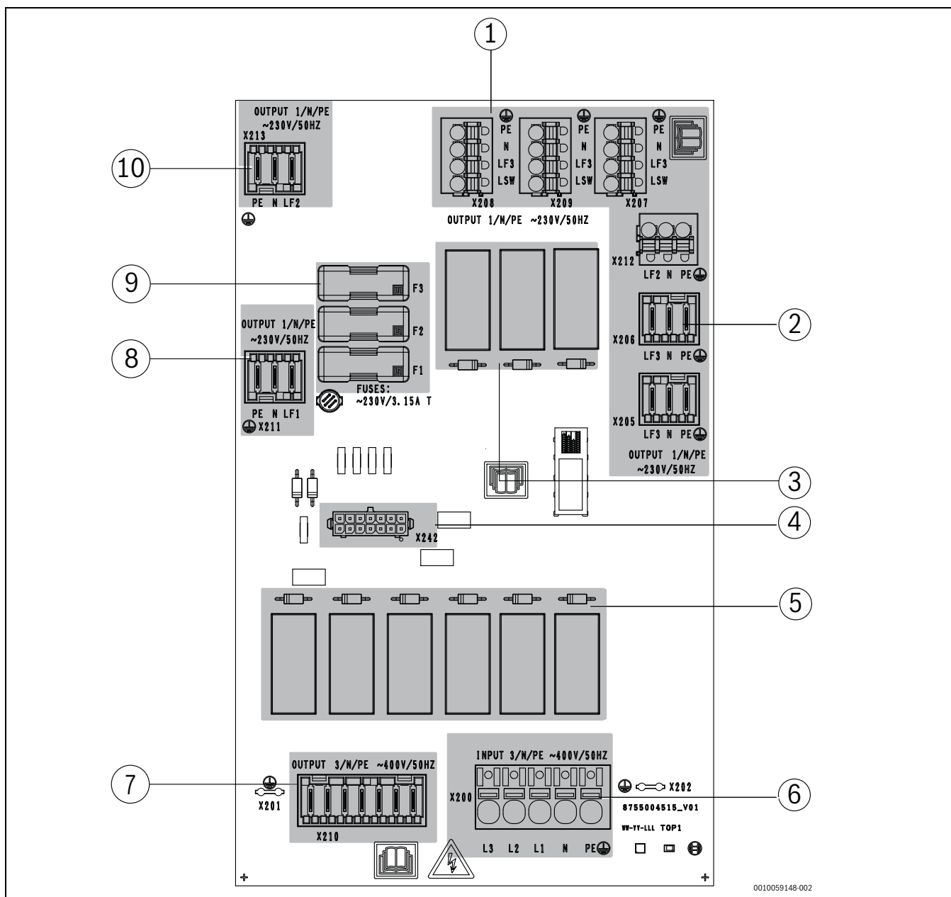
Afb. 41 Aansluitingen op de XCU-SEH
