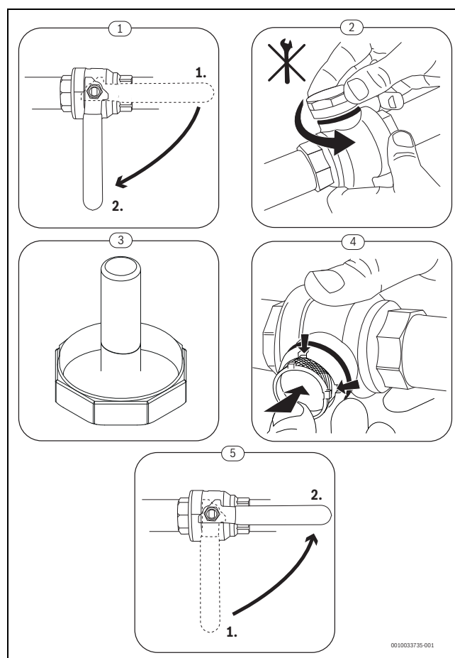
Afb. 54 Deeltjesfilter reinigen
