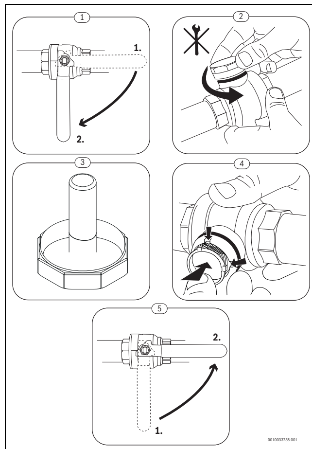
Afb. 52 Deeltjesfilter reinigen
