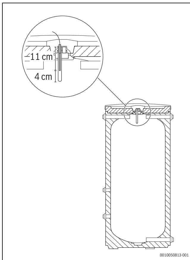
Fig. 52 Mise en place de la sonde de température de départ T0
