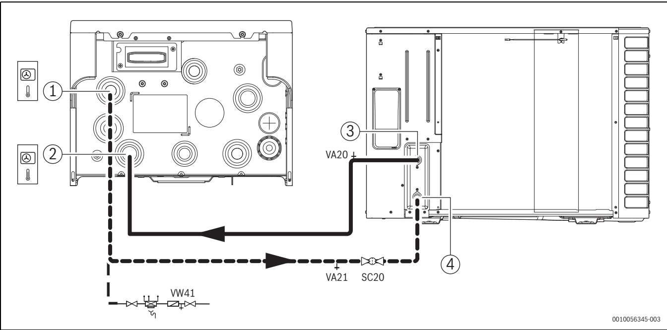
Fig. 21 Raccordement de l'unité intérieure à l'unité extérieure
