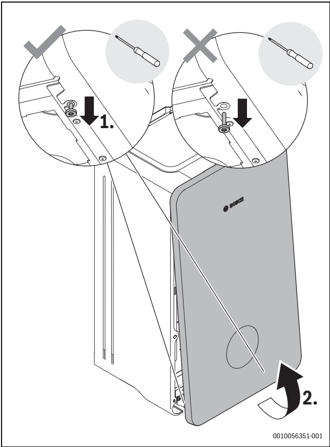
Fig. 11 Retirer le cache avant
