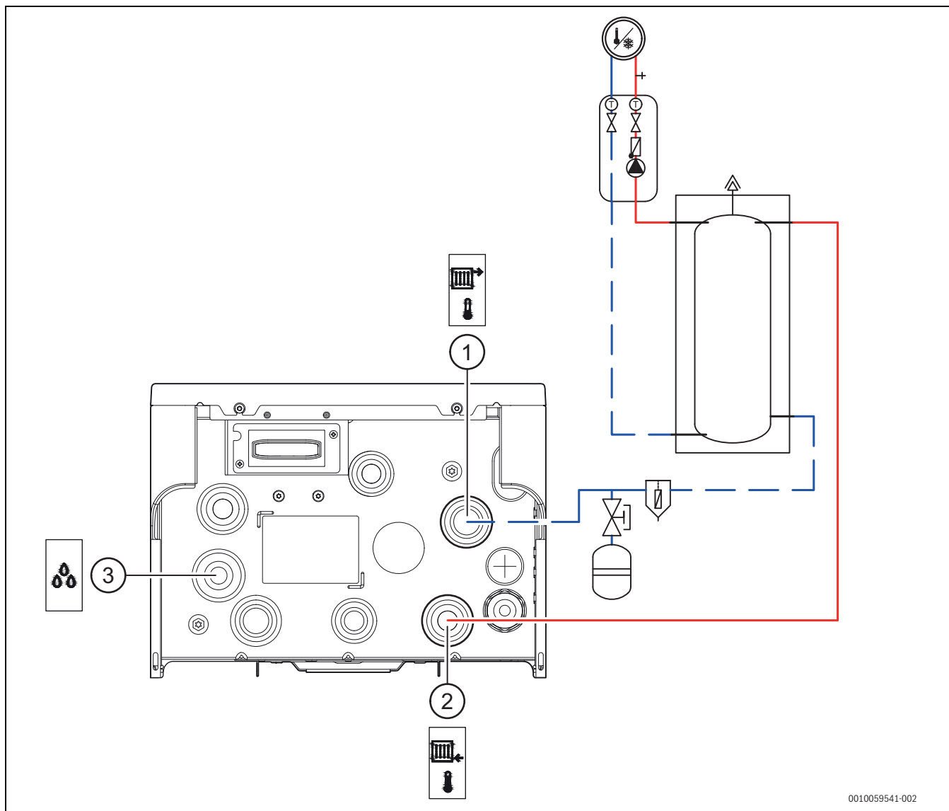
Fig. 26 Raccordement de l'unité intérieure au système de chauffage
