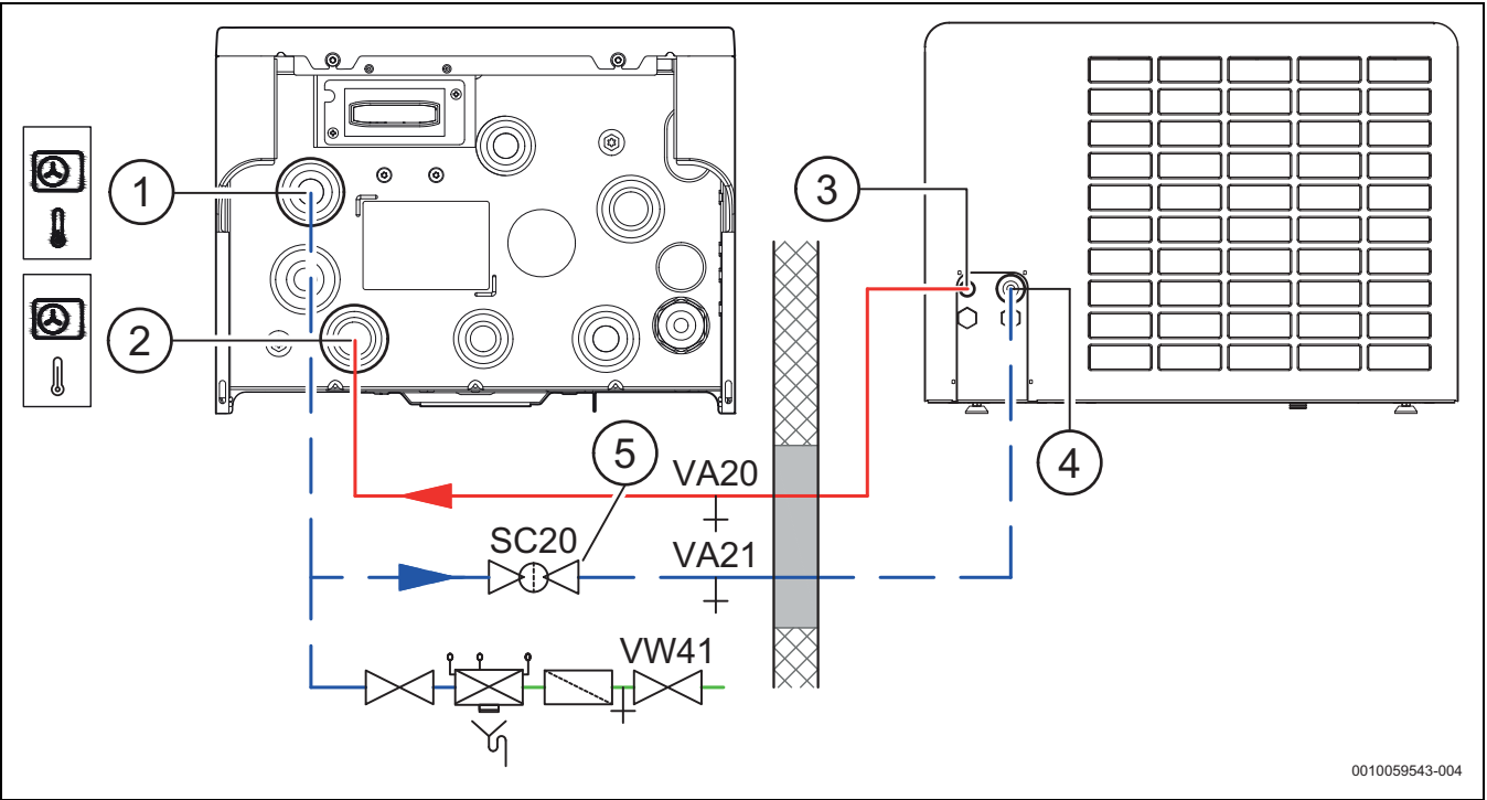
Fig. 25 Raccordement de l'unité intérieure à l'unité extérieure
