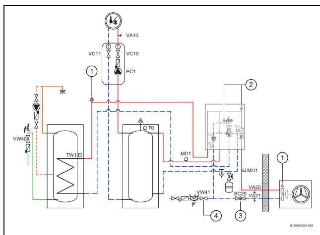
Fig. 30 Unité intérieure, unité extérieure, préparateur d'eau chaude sanitaire et un seul système de chauffage
