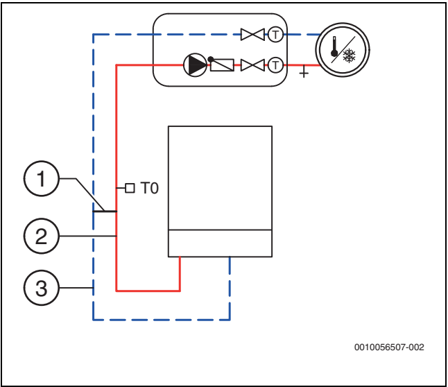
Fig. 29 Circuit de chauffage avec by-pass
