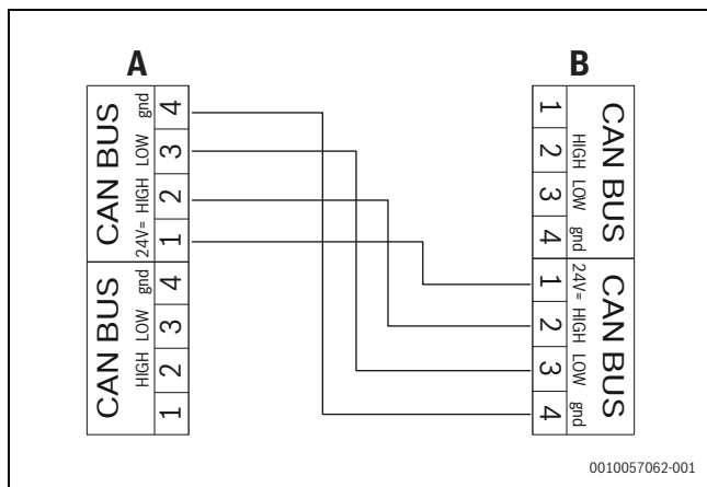
Fig. 47 BUS CAN, unité extérieure - unité intérieure
