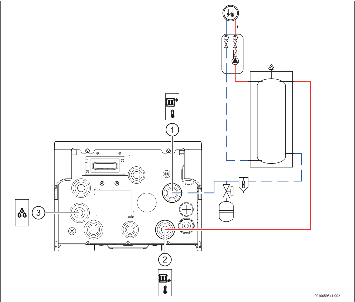
Fig. 33 Raccordement de l'unité intérieure au système de chauffage
