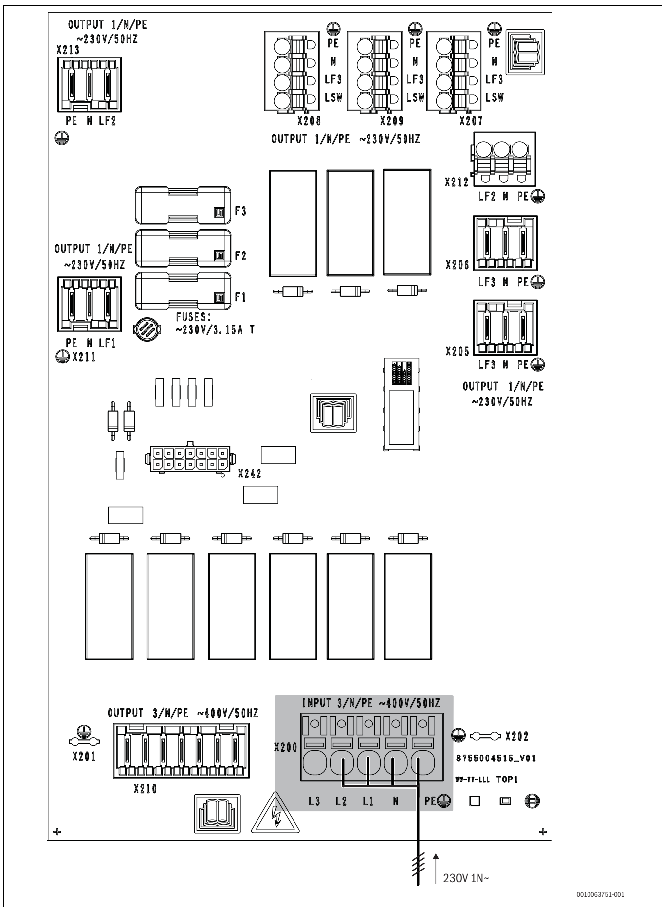
Fig. 44 Raccordement 230 V pour l'unité intérieure
