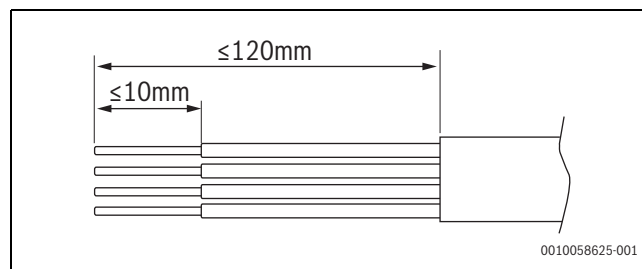
Fig. 49 Dénudage CAN-BUS
