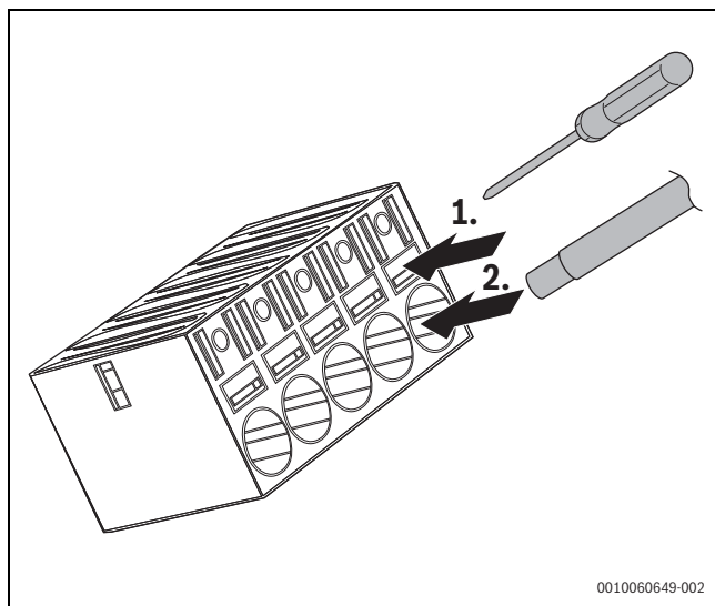
Fig. 42 Installation des câbles
