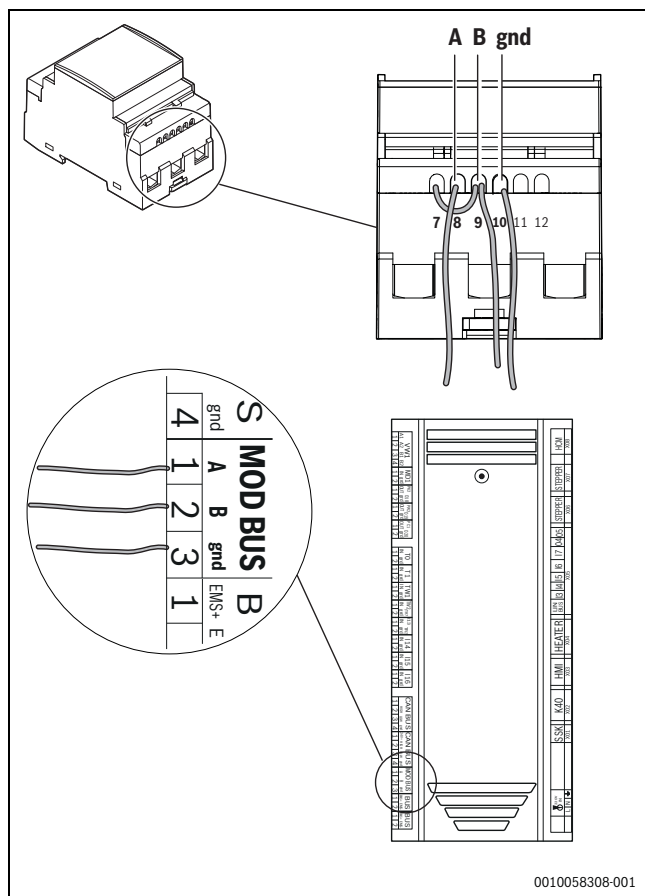
Fig. 15 Raccordement du compteur électrique Power Meter 5000 à l'unité intérieure
