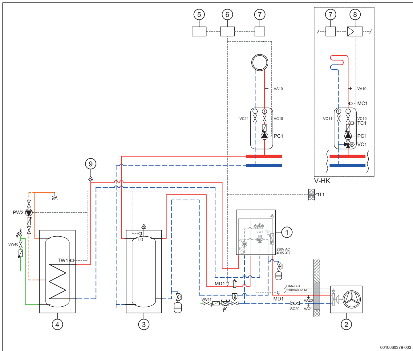
Fig. 56 Unité extérieure, unité intérieure, ballon tampon et ballon d'eau chaude sanitaire
