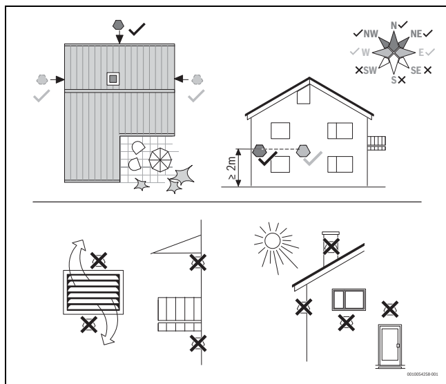
Fig. 51 Position de la sonde de température extérieure
