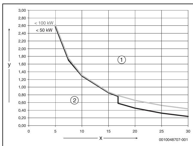
Fig. 8 Générateurs de chaleur &lt; 50 kW–100 kW
