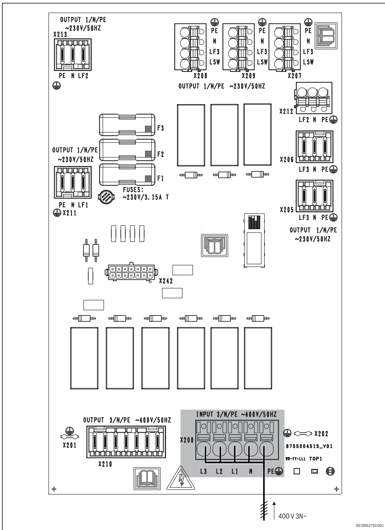
Fig. 43 Raccordement 400 V pour l'unité intérieure
