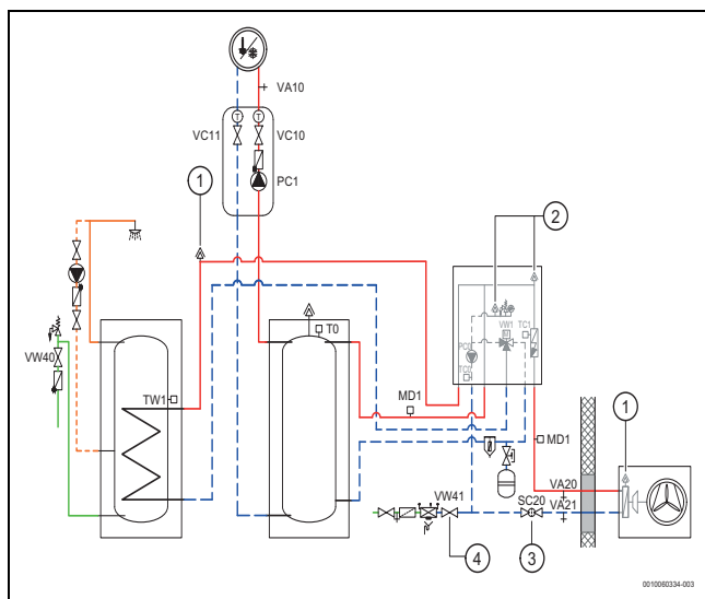
Fig. 23 Unité intérieure, unité extérieure, préparateur d'eau chaude sanitaire et un seul système de chauffage
