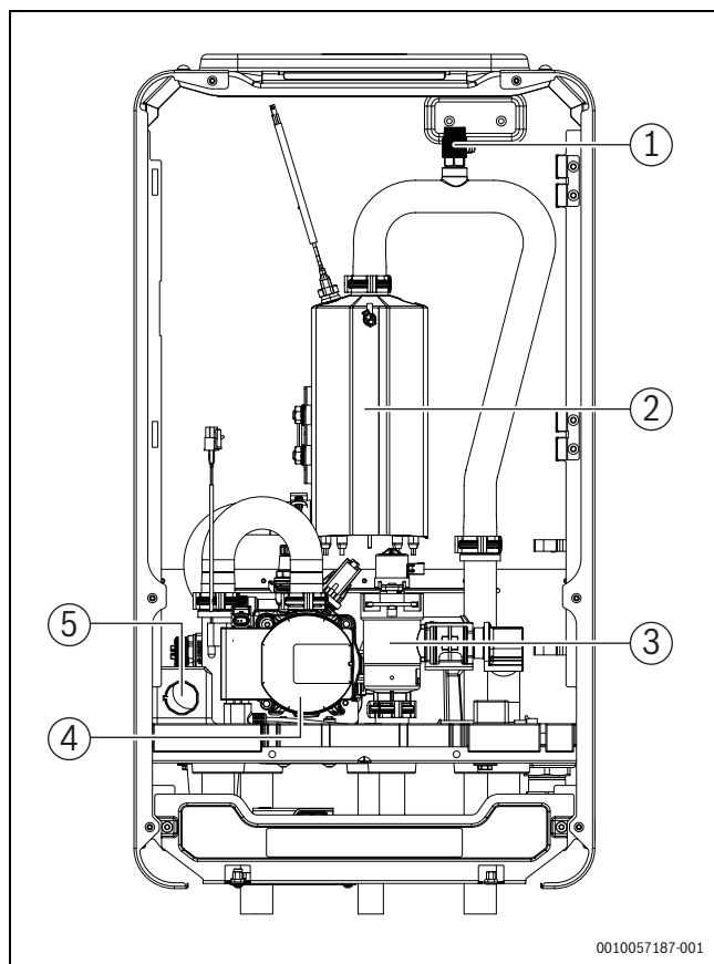
Fig. 5 Composants
