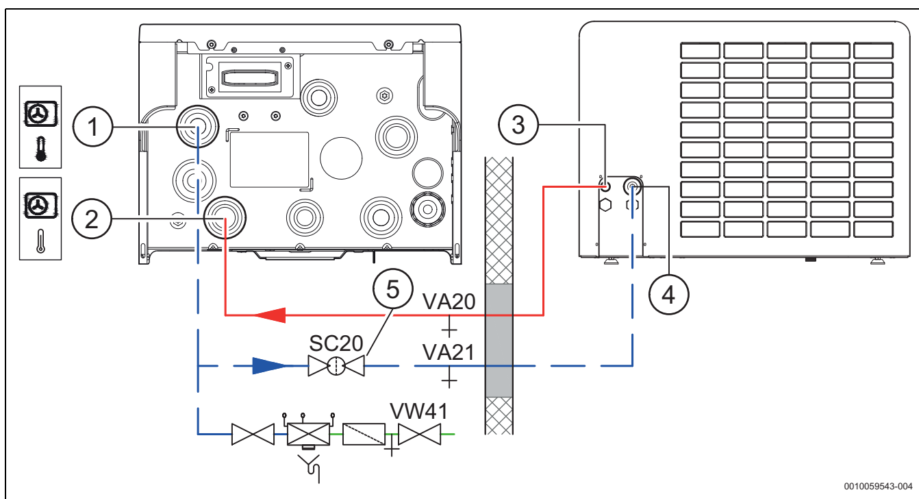
Fig. 32 Raccordement de l'unité intérieure à l'unité extérieure
