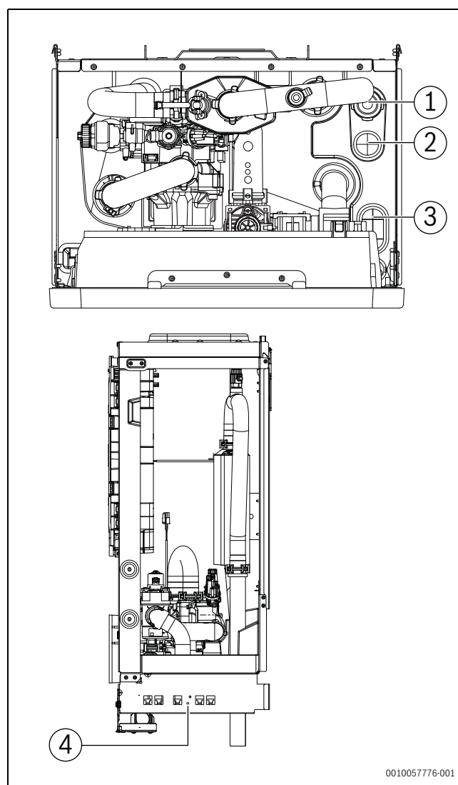
Fig. 39 Presse-étoupe et gaines vers l'unité intérieure (alimentation principale, accessoires et basse tension)
