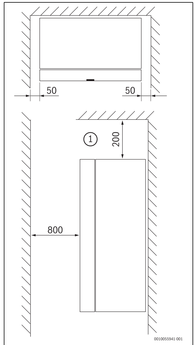
Fig. 4 Dégagements minimaux avec les pièces ou murs voisins (mm)
