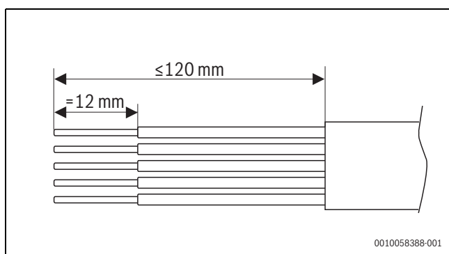
Fig. 38 Raccordement à l'alimentation secteur avec dénudage des fils
