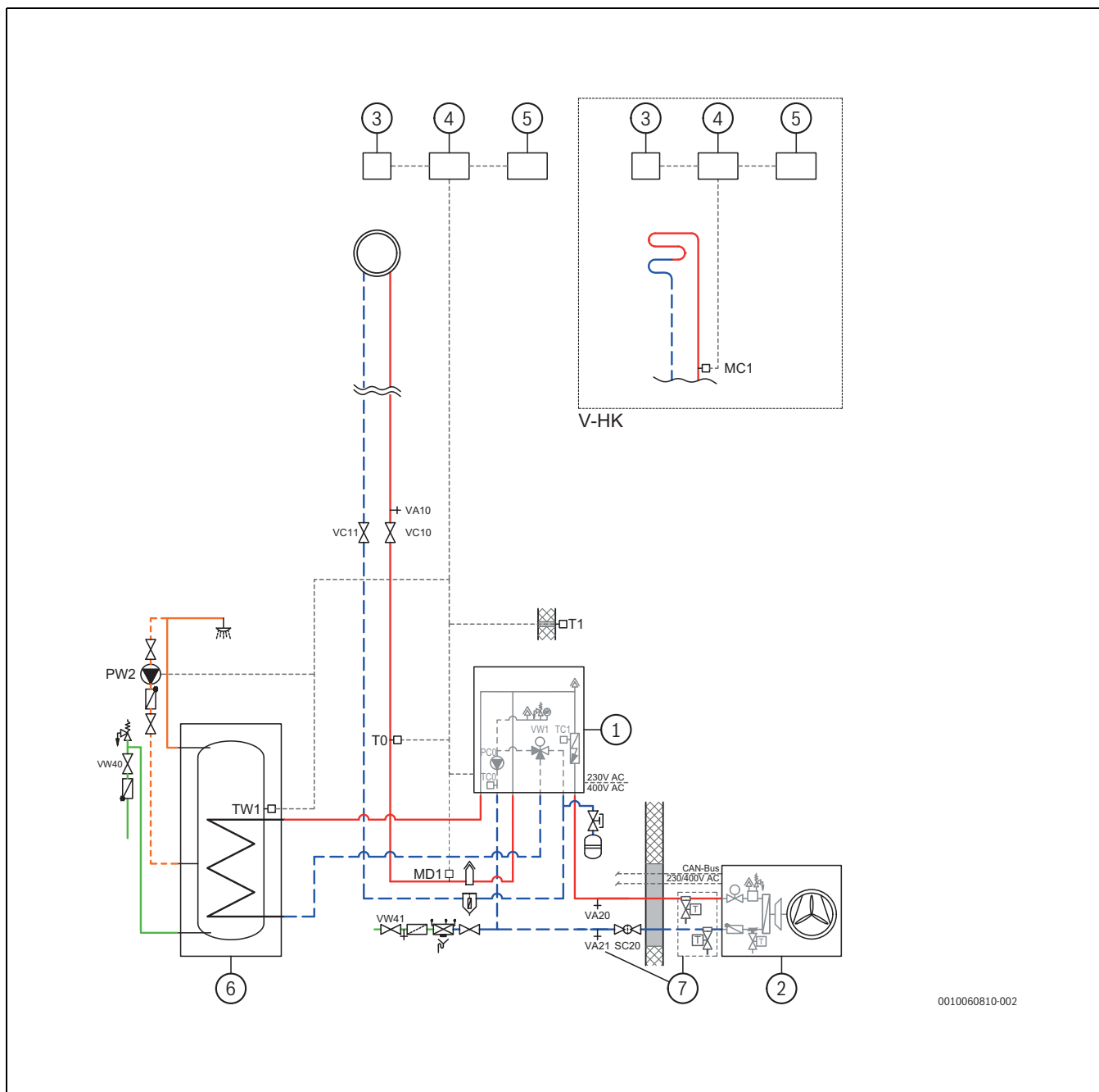
Fig. 55 Unité extérieure, unité intérieure et ballon d'eau chaude sanitaire
