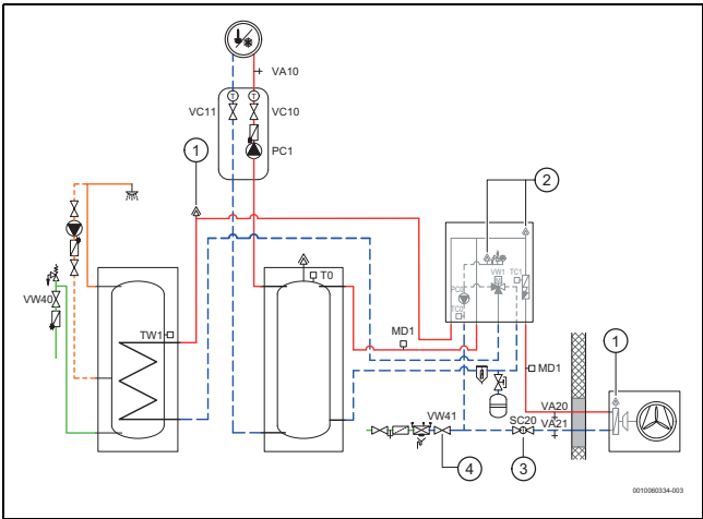
Fig. 37 Unité intérieure, unité extérieure, préparateur d'eau chaude sanitaire et un seul système de chauffage
