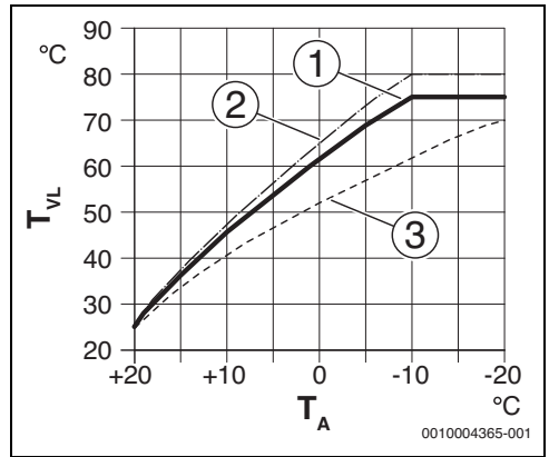
Fig. 12 Réglage de la courbe de chauffage pour radiateurs Pente ascendante au-dessus de la température de référence T_{AL} et température extérieure minimale T_{A,min}
