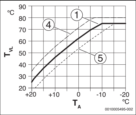
Fig. 13 Réglage de la courbe de chauffage pour radiateurs Décalage parallèle par la température ambiante souhaitée
