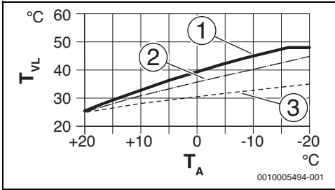
Fig. 10 Réglage de la courbe de chauffage pour chauffage par le sol Pente ascendante au-dessus de la température de référence T_{AL} et température extérieure minimale T_{A,min}
