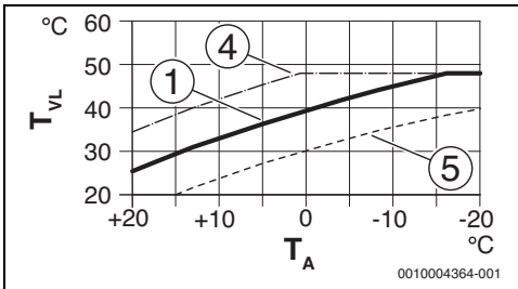
Fig. 11 Réglage de la courbe de chauffage pour chauffage par le sol Décalage parallèle par la température ambiante souhaitée
