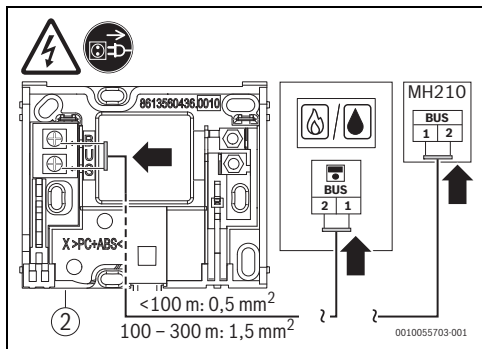
Fig. 6 Raccordement du module de commande
