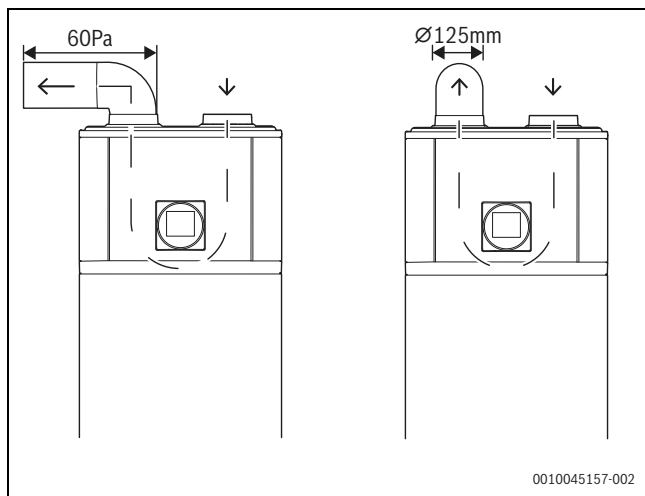
Afb. 13 Speciaal luchtkanaal
