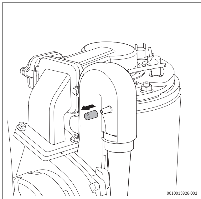
Afb. 51 Meetnippel op de menginrichting
