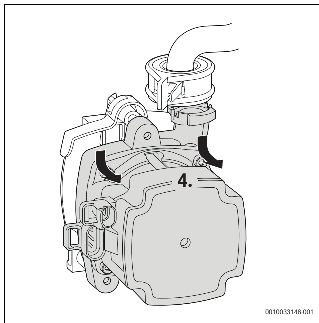
Afb. 55 Cv-pomp afnemen
