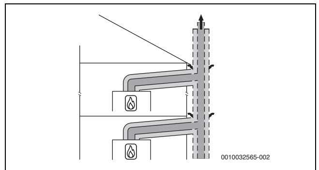
Afb. 24 Collectief systeemconform C (12)3x met concentrisch luchttoevoer/rookgasafvoersysteem in opstellingsruimte
