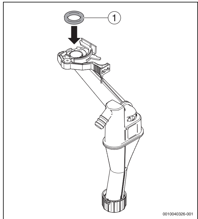
Afb. 68 De nieuwe dichting correct op de condenssifon plaatsen
