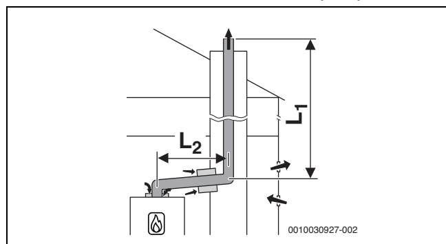
Afb. 19 Star rookgasafvoer door de schacht conform B 53p met open luchttoevoer aan het toestel en concentrisch verbindingstuk tussen opstellingsruimte en schacht
