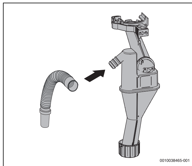
Afb. 36 Condensafvoer op het aansluitstuk steken
