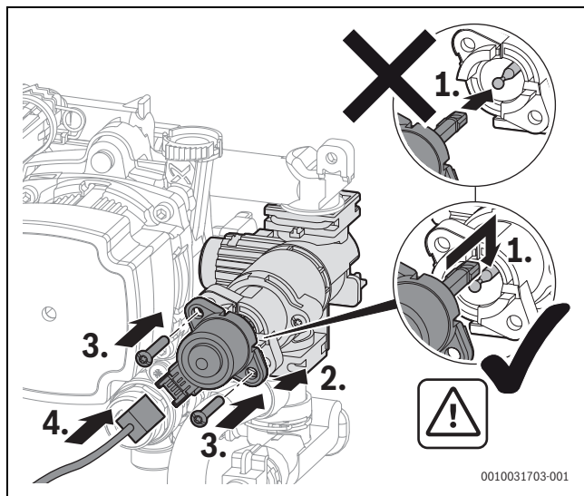
Afb. 74 Motor van de 3-wegklep inbouwen (variant met schroeven)
