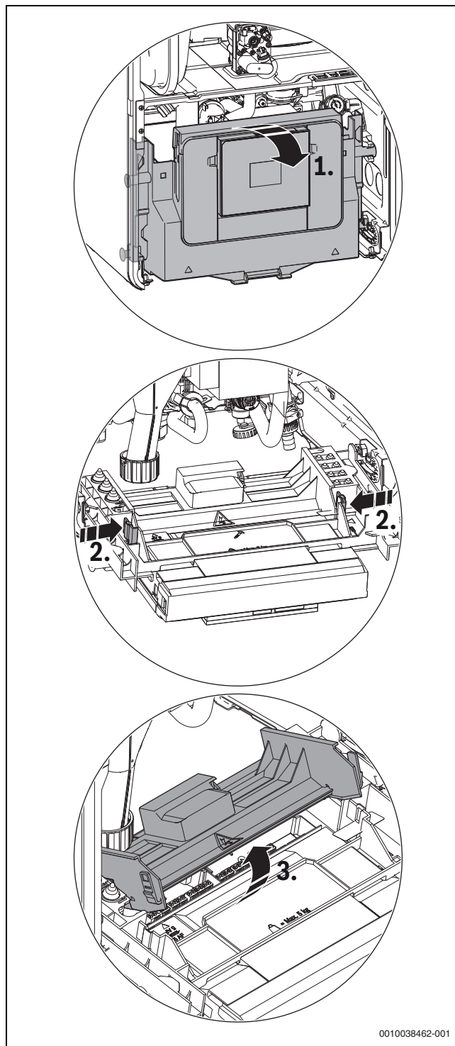
Afb. 41 Afdekking open klappen
