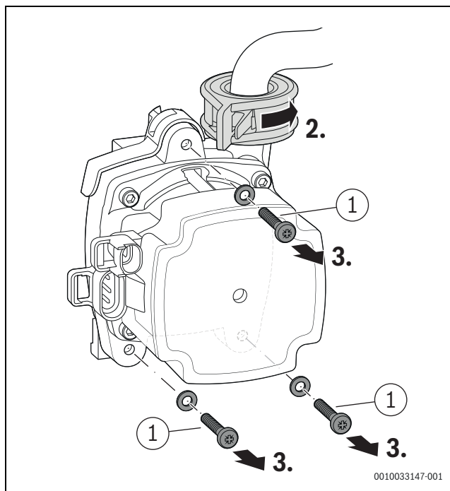
Afb. 54 Cv-pomp ontgrendelen en schroeven verwijderen
