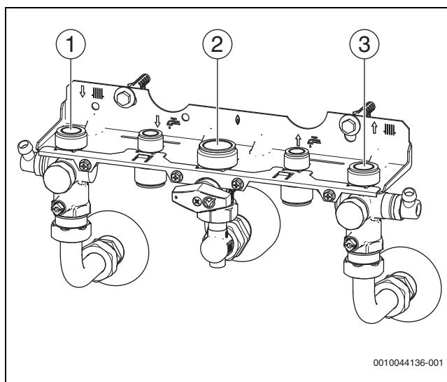
Afb. 40 Gas- en waterzijdige aansluitingen
