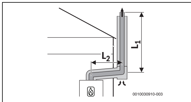
Afb. 16 Concentrisch luchttoevoer/rookgasafvoersysteem conform C 53x op de buitenmuur
