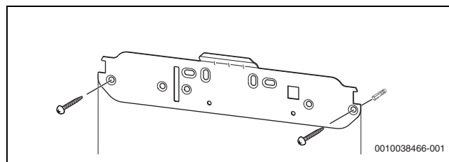
Afb. 32 Ophangbeugel monteren
