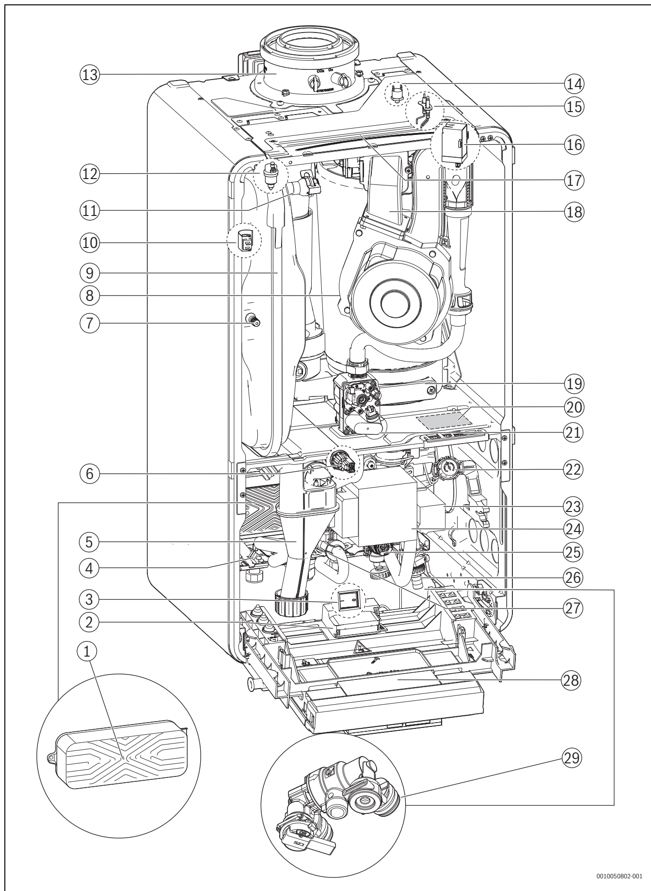
Afb. 6 Productoverzicht combitoestel
