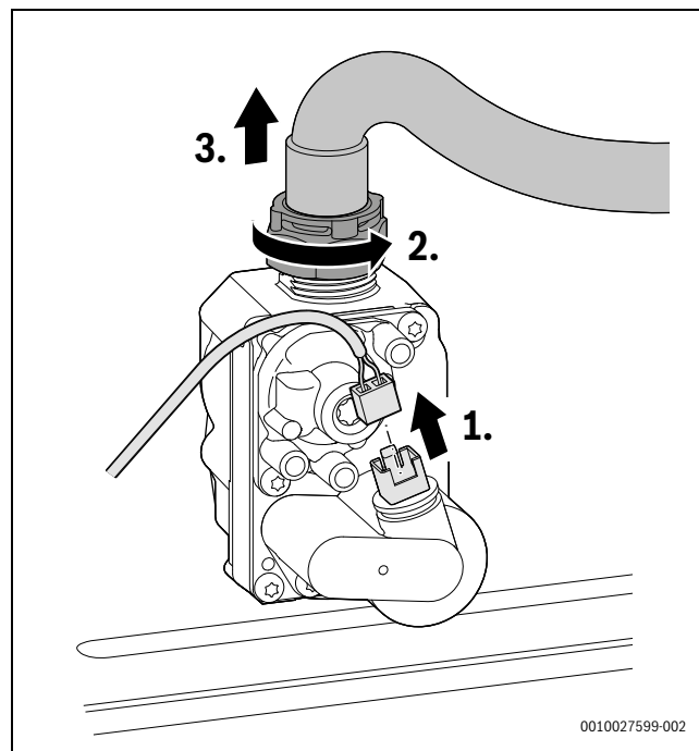
Afb. 57 Stekker op het gasblok lostrekken en wartelmoer met gasslang afnemen
