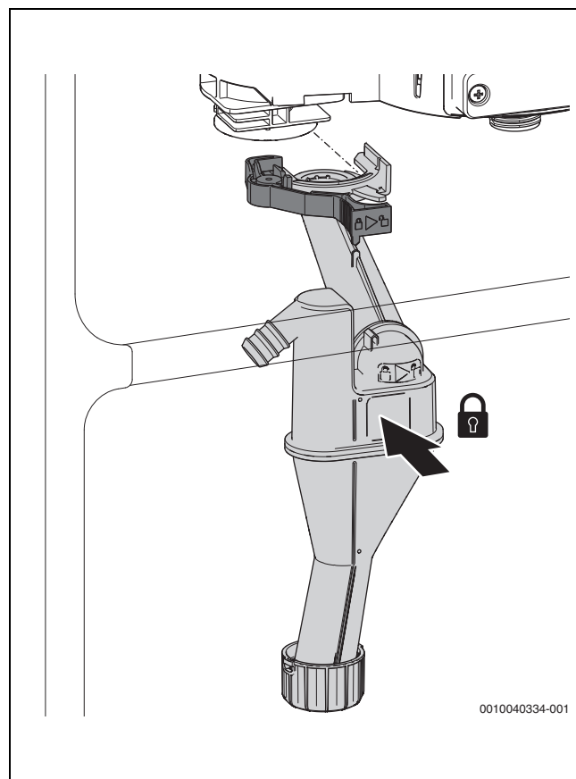
Afb. 70 Condenssifon plaatsen
