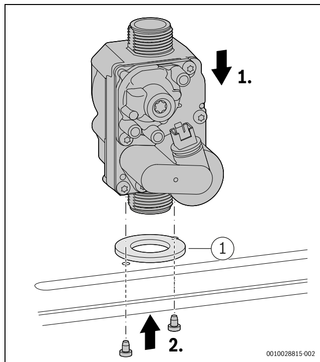
Afb. 61 Gasblok inbouwen
