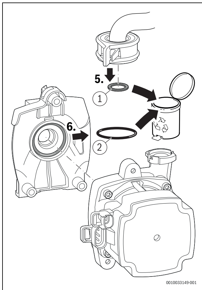
Afb. 56 Dichtingen afvoeren
