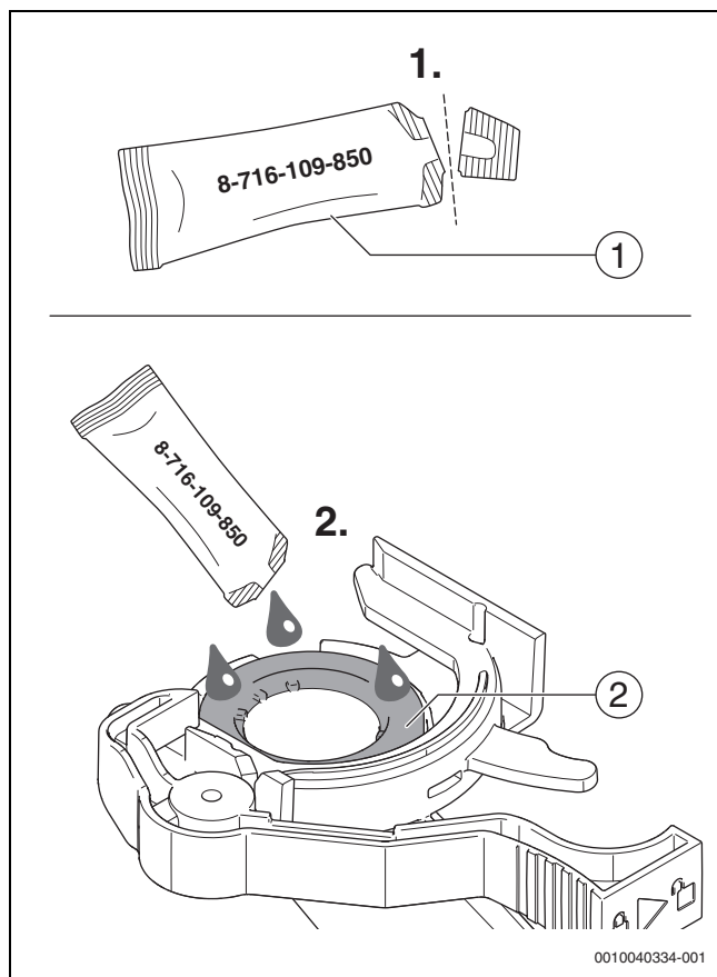
Afb. 69 Dichting smeren
