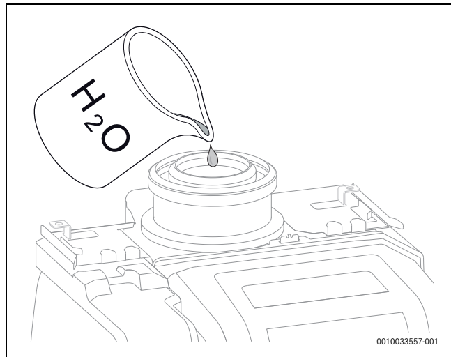
Afb. 37 Condenssifon met water vullen
