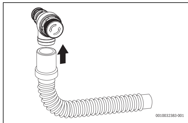
Afb. 35 Slang op veiligheidsventiel (verwarming) monteren
