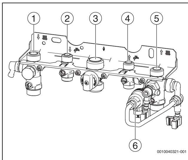
Afb. 39 Gas- en waterzijdige aansluitingen
