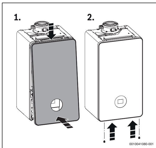
Afb. 44 Mantel monteren
