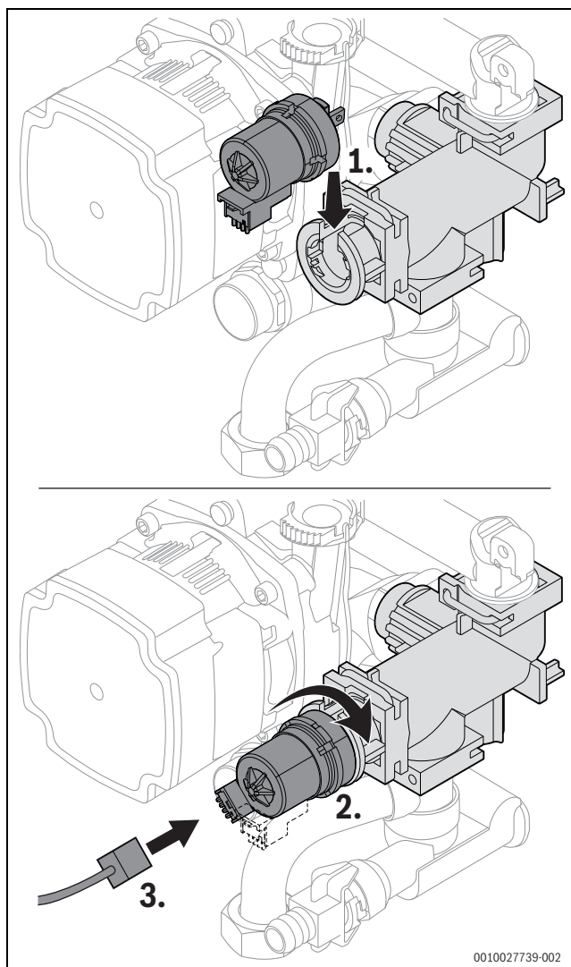
Afb. 72 Motor van de 3-wegklep inbouwen (variant zonder schroeven)
