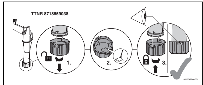
Afb. 67 Vuilfilter reinigen
