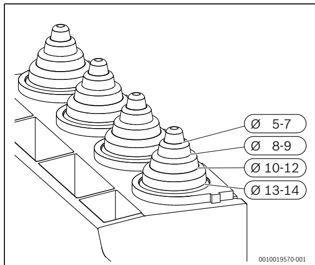
Afb. 42 Trekontlasting op kabeldiameter aanpassen
