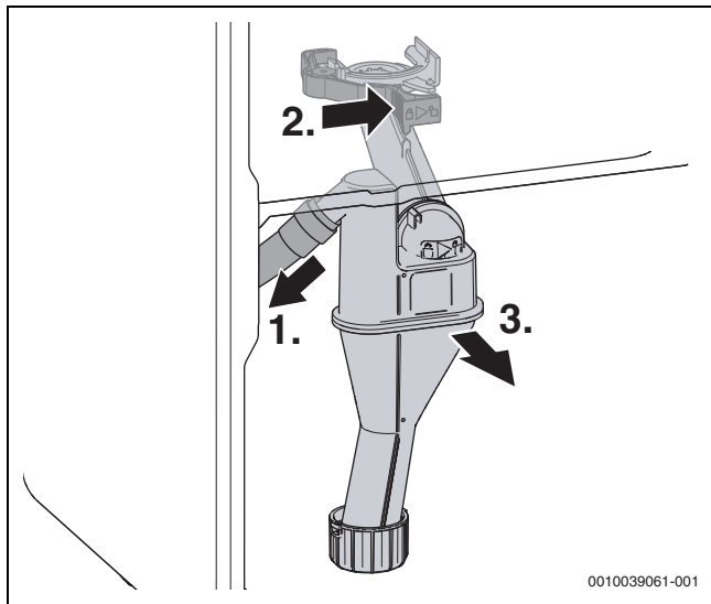
Afb. 66 Condenssifon demonteren
