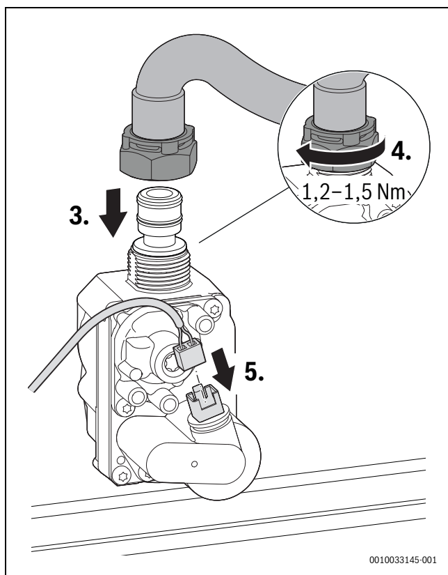
Afb. 64 Gasslang en stekker aansluiten – Draaimoment aanhouden
