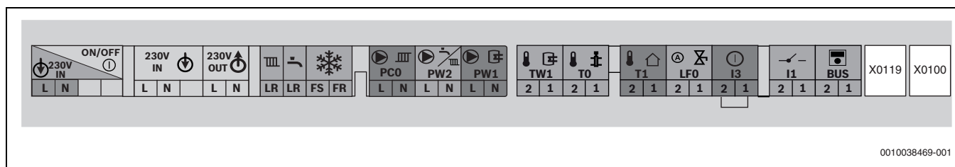
Afb. 43 Klemmenstrook voor extern toebehoren
