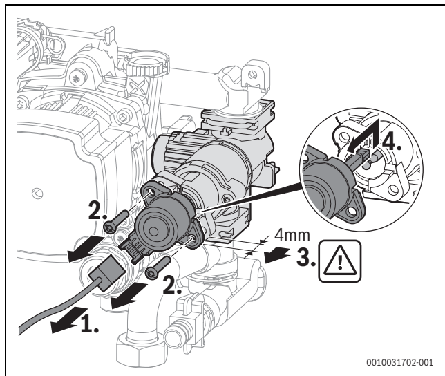
Afb. 73 Motor van de 3-wegklep uitbouwen (variant met schroeven)
