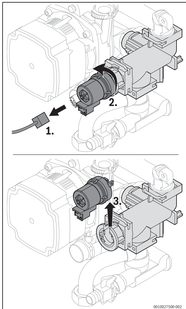
Afb. 71 Motor van de 3-wegklep uitbouwen (variant zonder schroeven)
