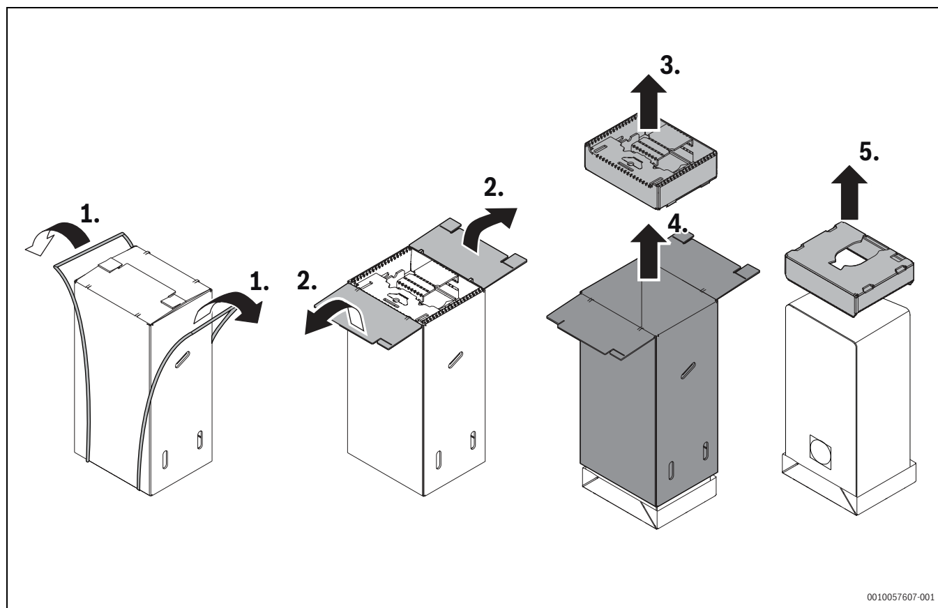
Afb. 31 Uitpakinstructies
