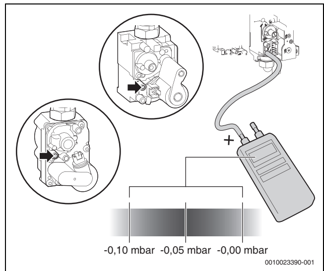
Afb. 48 Meten drukverschil
