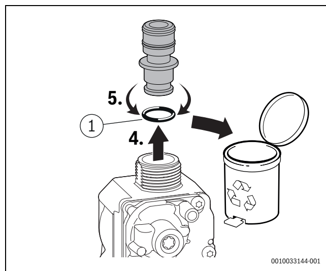
Afb. 58 Gassmoorklep afnemen
