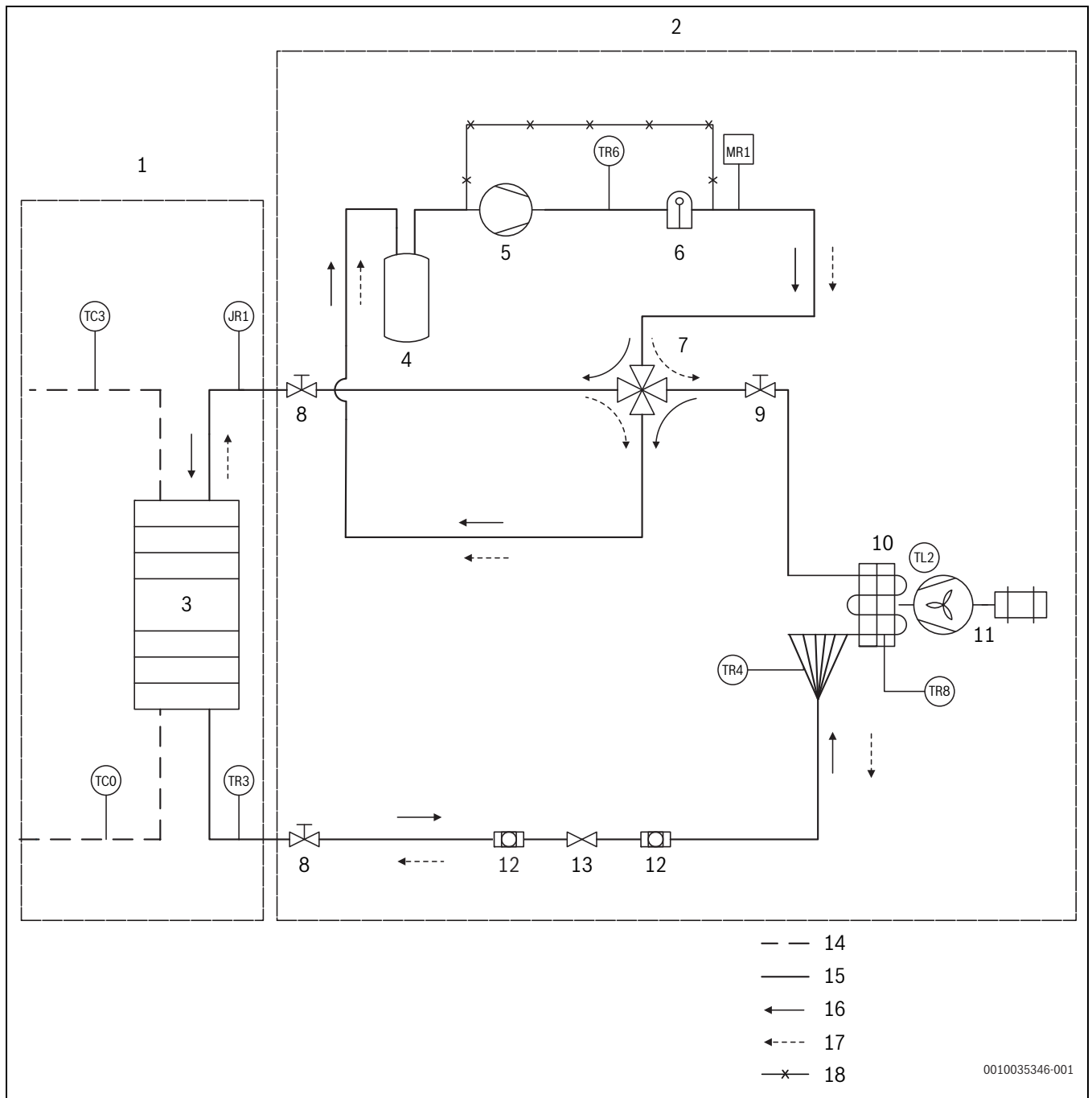
Afb. 25 Diagram koelmiddelcircuit
