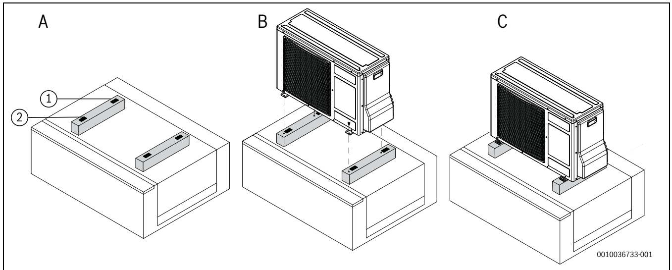
Afb. 9 Vloerstaande buiteneenheid
