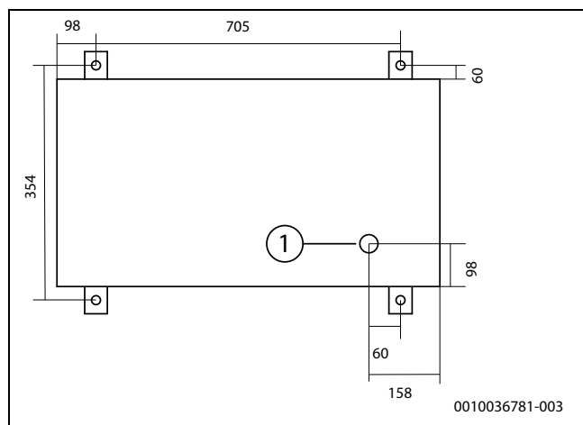
Afb. 7 Bodemplaat buiteneenheid (mm)
