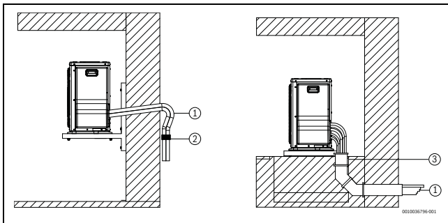
Afb. 17 Aansluiten van de buiteneenheid op de binneneenheid
