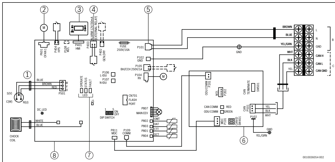
Afb. 26 Schakelschema buiteneenheid eenfase CS3400iAWS 4 OR-S
