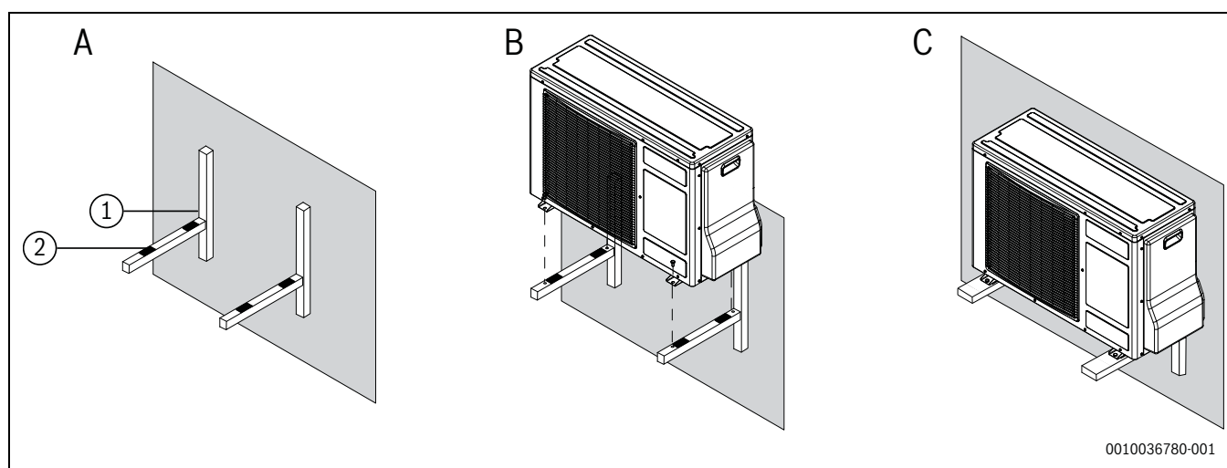
Afb. 8 Buiteneenheid voor wandmontage
