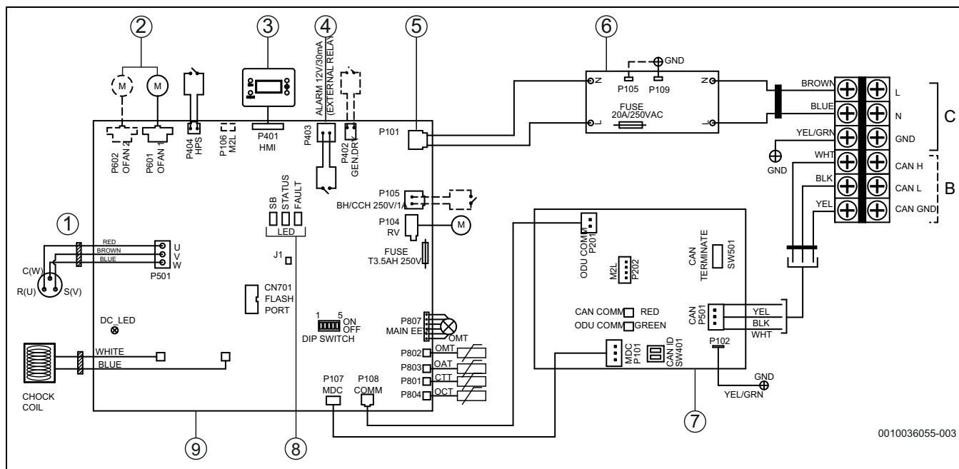
Afb. 27 Schakelschema buiteneenheid eenfase CS3400iAWS 6 OR-S, CS3400iAWS 8 OR-S en CS3400iAWS 10 OR-S
