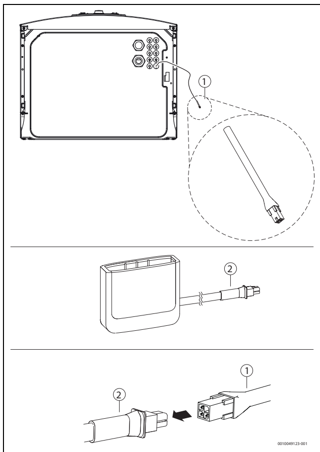
Afb. 26 Aansluiten van de Draadloze module.
