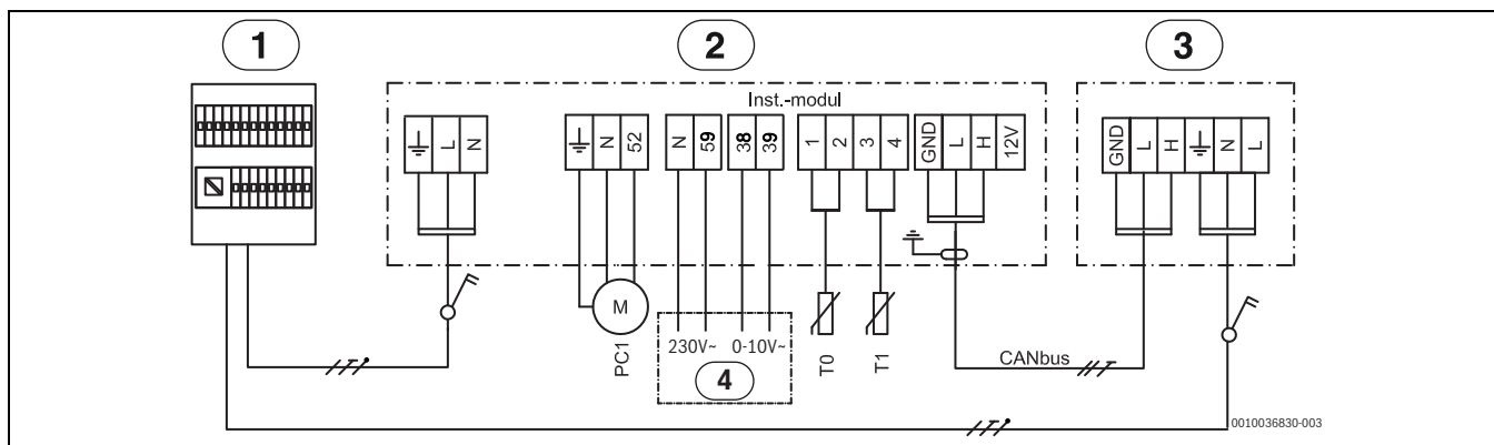
Afb. 41 Schakelschema 5,85 kW 3 N~
