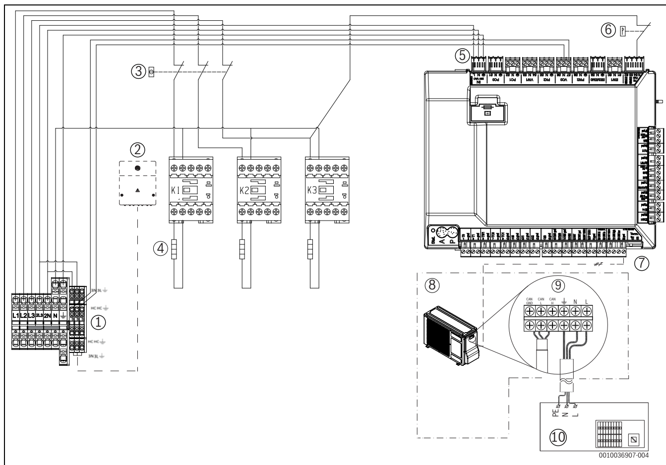
Afb. 42 400 V 3 N~ binneneenheid met 230 V~ buiteneenheid
