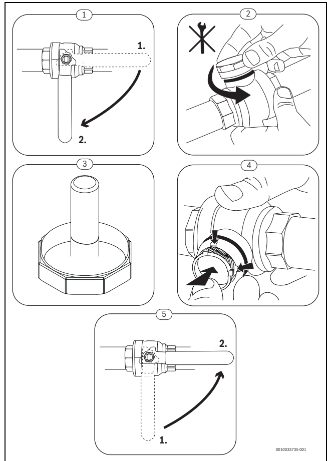
Afb. 17 Deeltjesfilter reinigen
