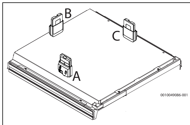
Afb. 27 Bevestigen van de houder op de bovenmantel van de binneneenheid. Naast de houder, toont de afbeelding ook de Draadloze module welke zich in de houder bevindt
