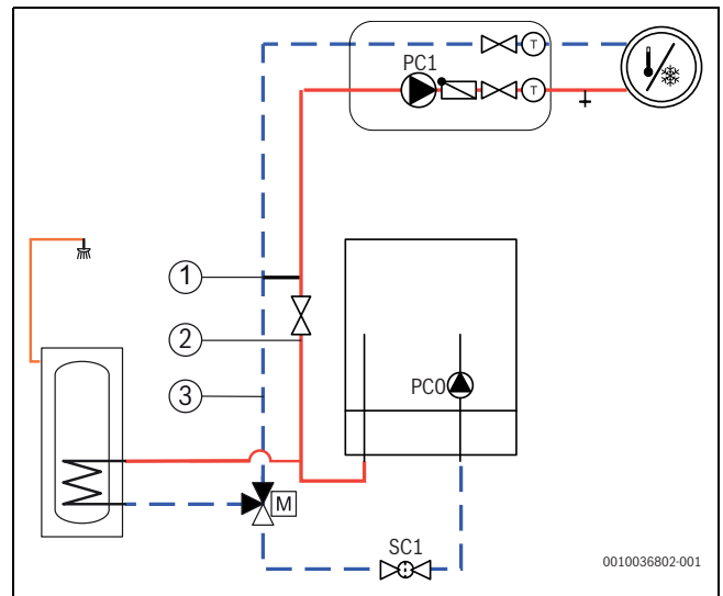
Afb. 32 Binneneenheid met cv-circuit en warmwaterbereiding
