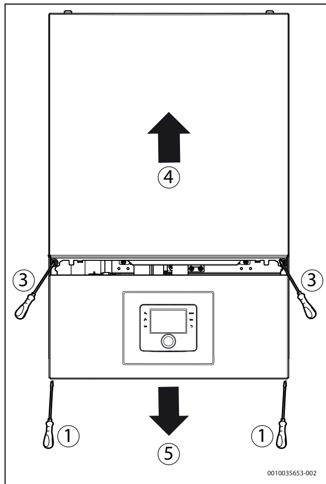
Afb. 6 Verwijder frontpaneel
