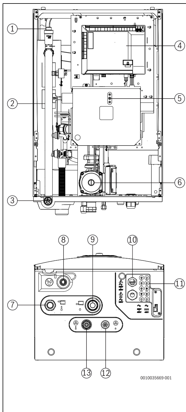
Afb. 3 Componenten en leidingaansluitingen van de binneneenheid met elektrische bijverwarming (aanzicht met lekbak)
