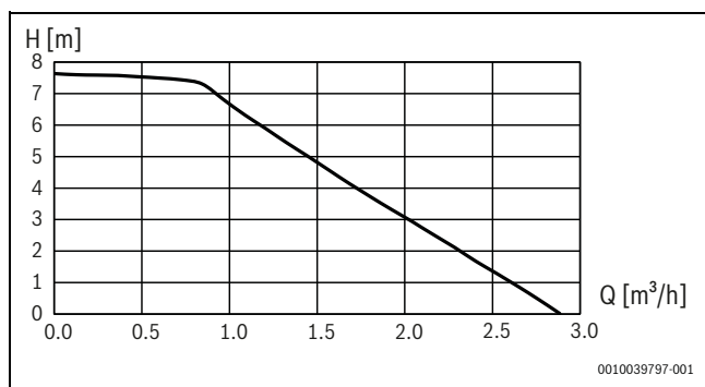
Afb. 30 Capaciteitscurve van de primaire circulatiepomp (PCO)
