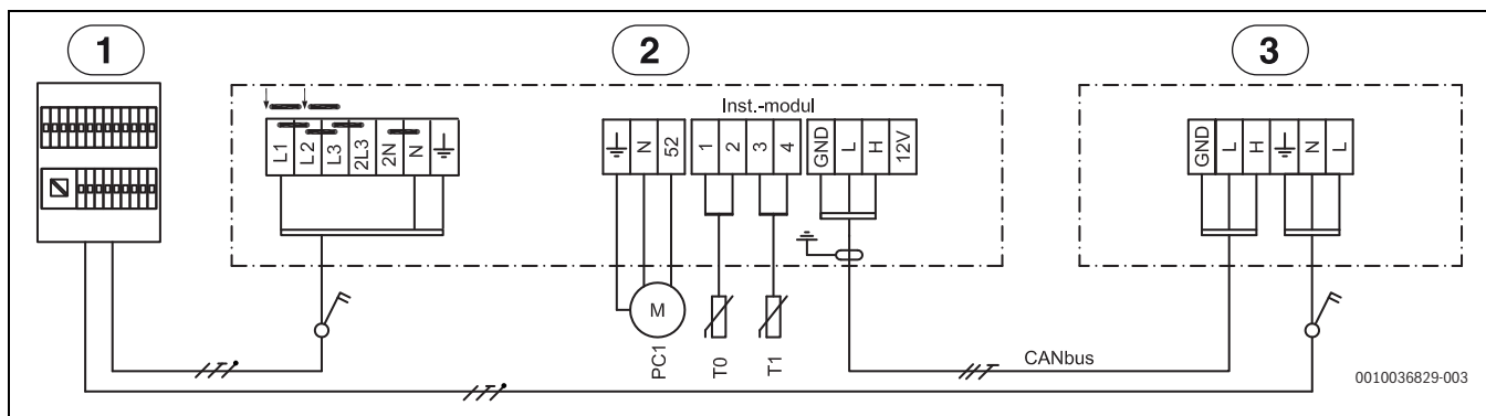
Afb. 40 Schakelschema 5,85 kW 230 V~
