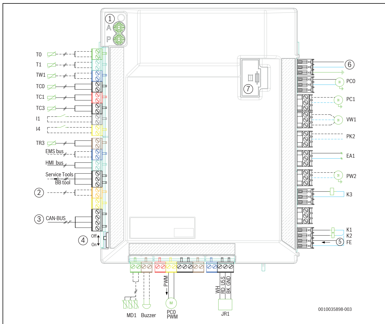
Afb. 38 Installatiemodule van de binneneenheid
