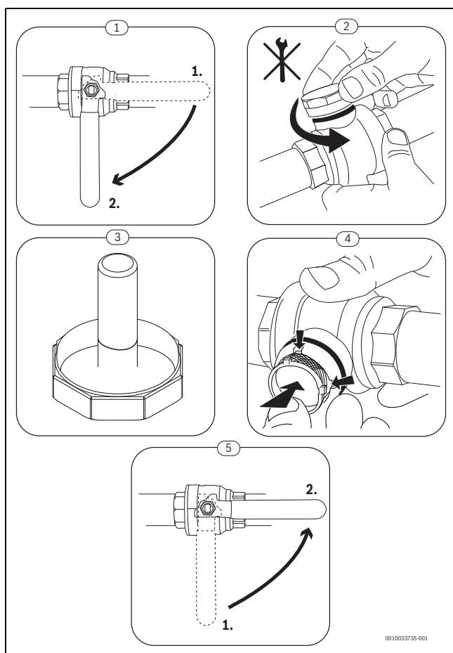
Afb. 6 Filterreiniging
