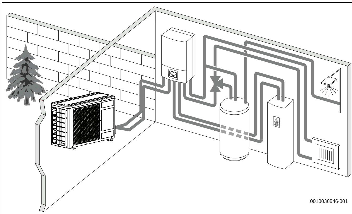
Afb. 2 Warmtepomp buiteneenheid, AWS B binneneenheid zonder elektrische bijverwarming, externe boiler en externe bijverwarming
