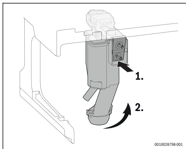
Afb. 59 Condenssifon uitnemen
