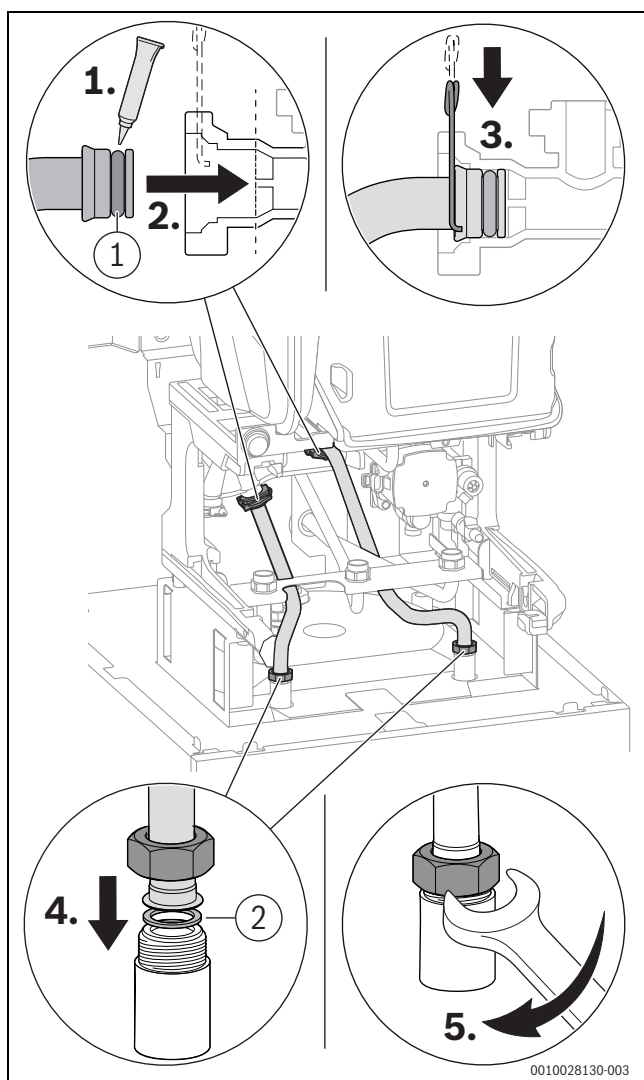
Afb. 60 Aanvoerleiding en retourleiding naar spiraalbuisboiler aansluiten
