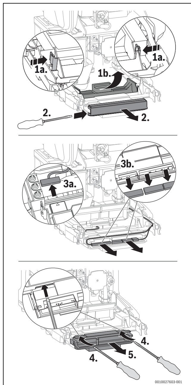
Afb. 140 Besturing uitnemen
