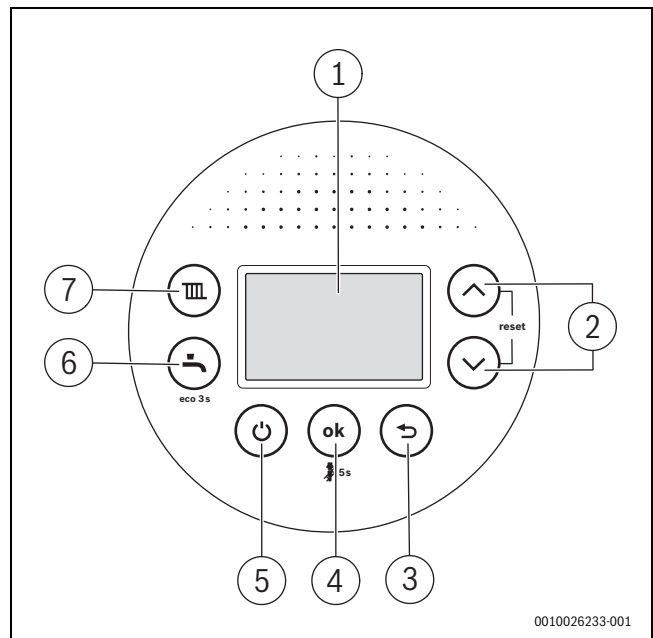
Afb. 93 Overzicht bedieningspaneel
