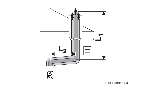
Afb. 23 Concentrisch luchttoevoer/rookgasafvoersysteem conform C 33x in schacht
