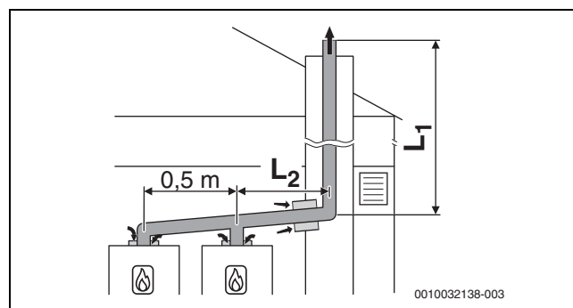
Afb. 40 Cascade met 2 toestellen:
