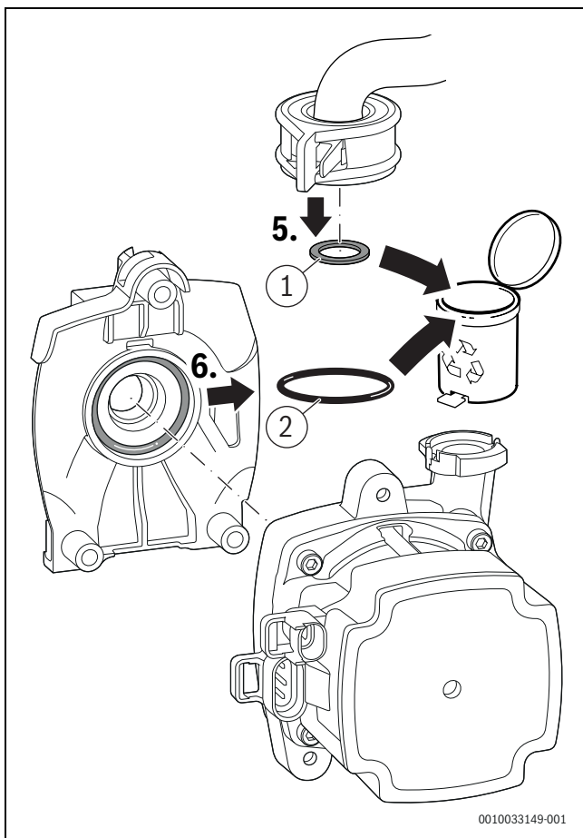
Afb. 131 Dichtingen afvoeren
