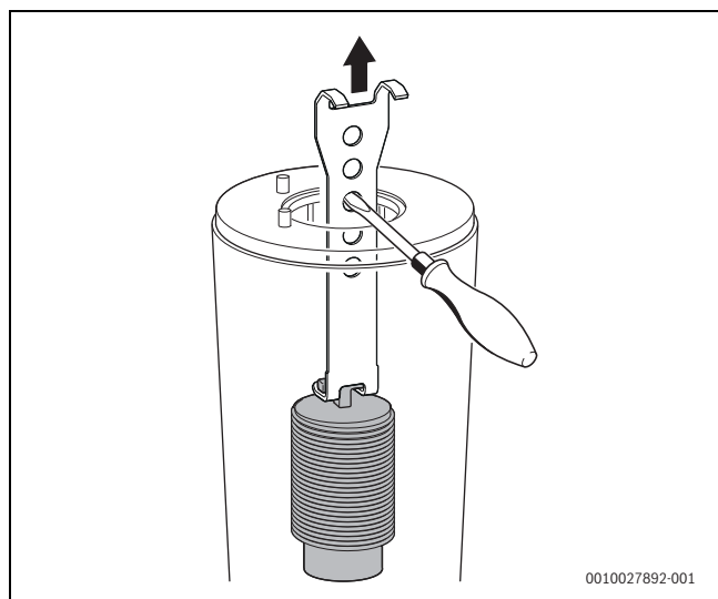
Afb. 119 Neem de onderste rookgasremmer uit
