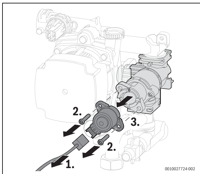
Afb. 145 Motor op 3-wegklep demonteren
