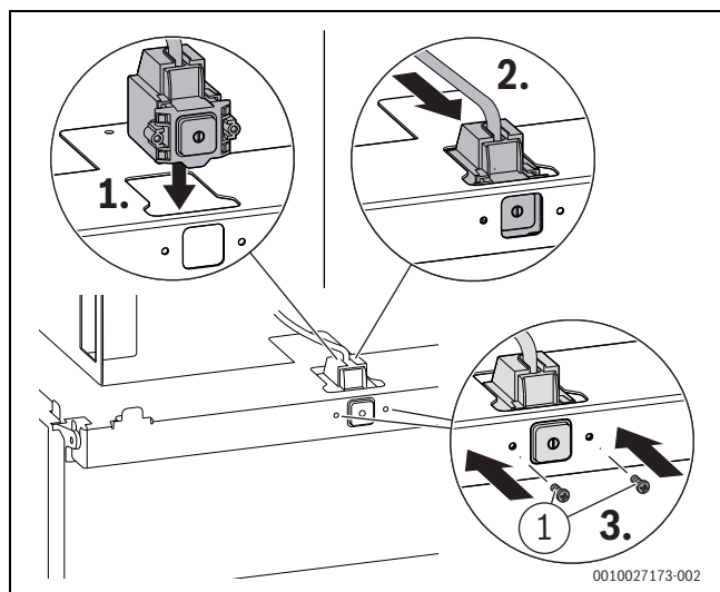
Afb. 77 Aan-uitschakelaar bevestigen
