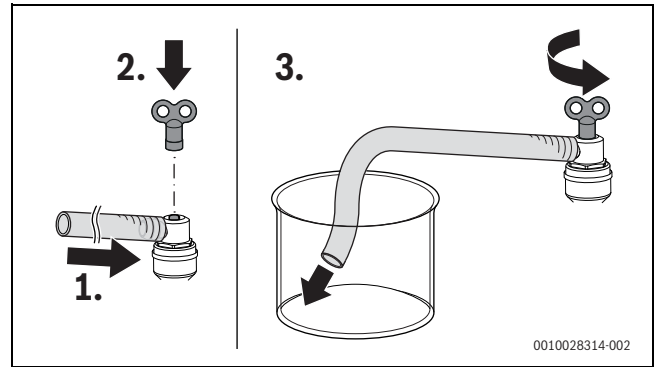
Afb. 75 Warmwatercircuit en cv-circuit ontluichten
