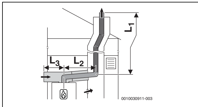
Afb. 26 Flexibel rookgasafvoersysteem conform C 53x in schacht en luchttoevoer/rookgasafvoersysteem met separate luchttoevoer en concentrische rookgasafvoer in opstellingsruimte
