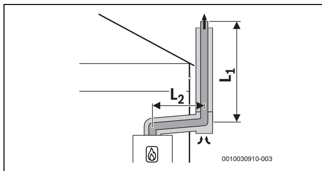
Afb. 27 Concentrisch luchttoevoer/rookgasafvoersysteem conform C 53x op de buitenmuur
