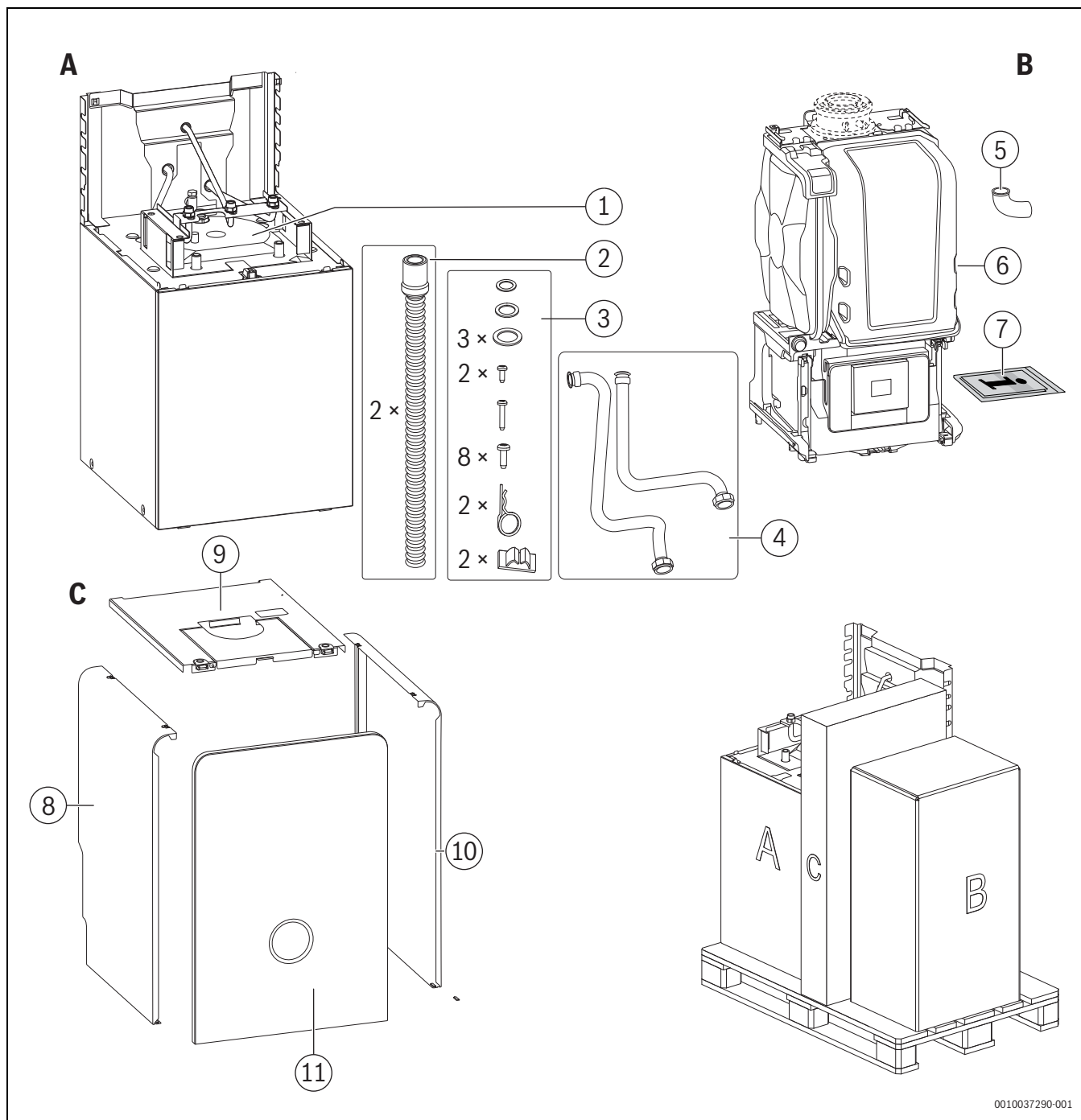
Afb. 4 Leveringsomvang
