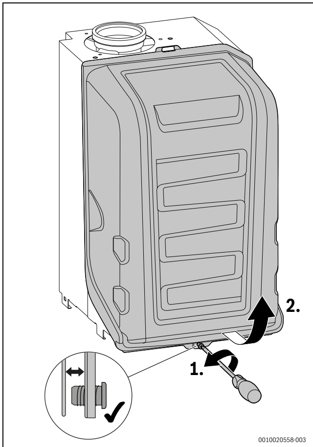
Afb. 74 Branderkap verwijderen
