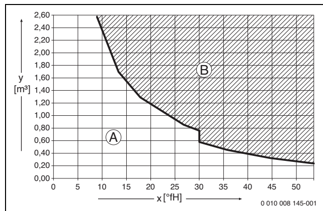
Afb. 44 Eisen aan het vul- en bijvulwater in °fH voor toestellen < 50 kW
