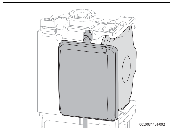
Afb. 46 2 expansievaten in het toestel gemonteerd
