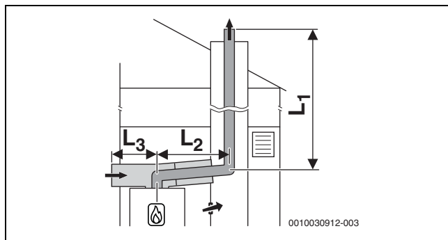
Afb. 25 Star rookgasafvoertraject conform C 53x in schacht en luchttoevoer/rookgasafvoersysteem met separate luchttoevoer en concentrische rookgasafvoer in opstellingsruimte
