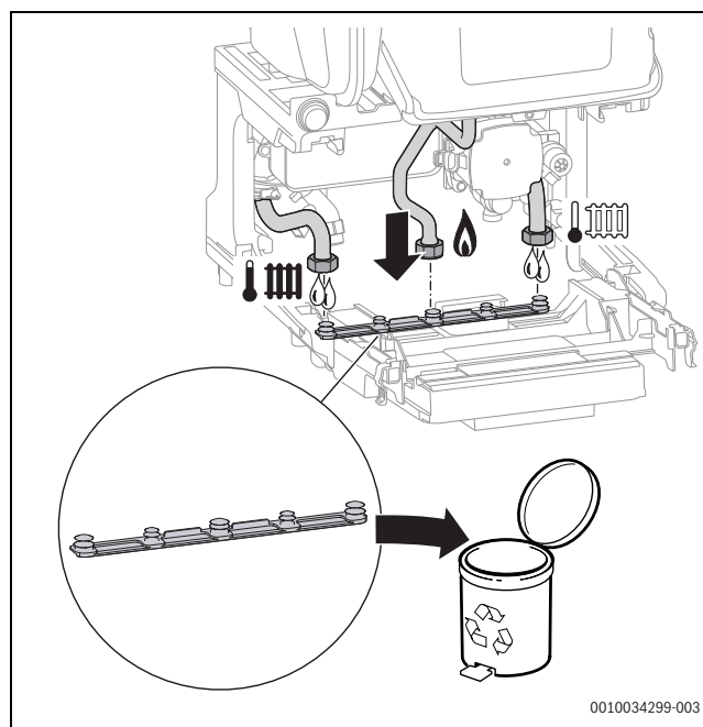
Fig. 55 Retirez la bande de protection de l'appareil
