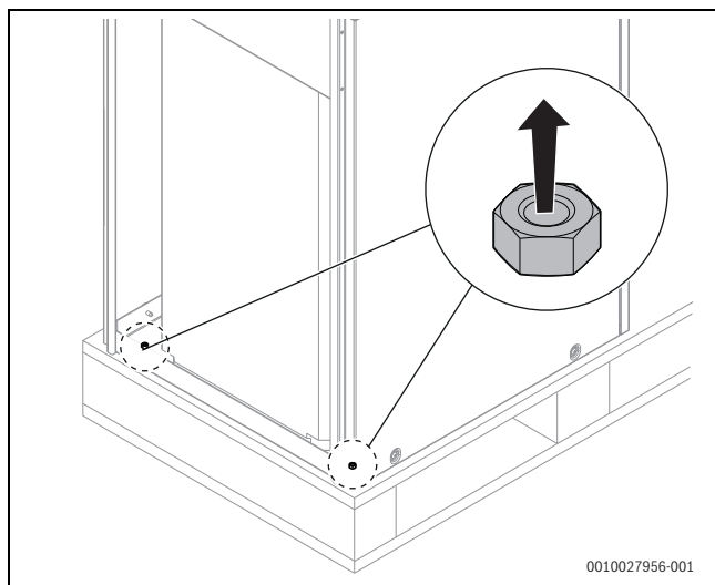
Fig. 49 Retirer la sécurisation pour le transport en bas de la partie arrière du ballon
