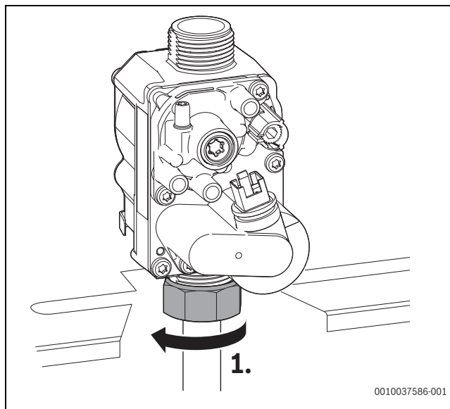
Fig. 134 Desserrage de l'écrou-raccord
