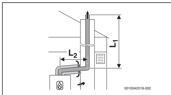
Fig. 31 Évacuation des fumées rigide dans le conduit selon B 53p avec arrivée d'air dépendant de l'air ambiant par le circuit d'air et de fumées concentrique dans le local d'installation
