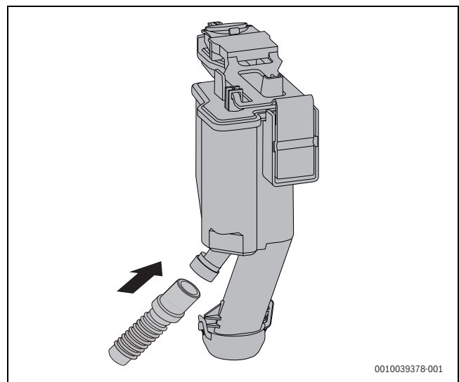
Fig. 68 Raccorder le tube au siphon de condensats
