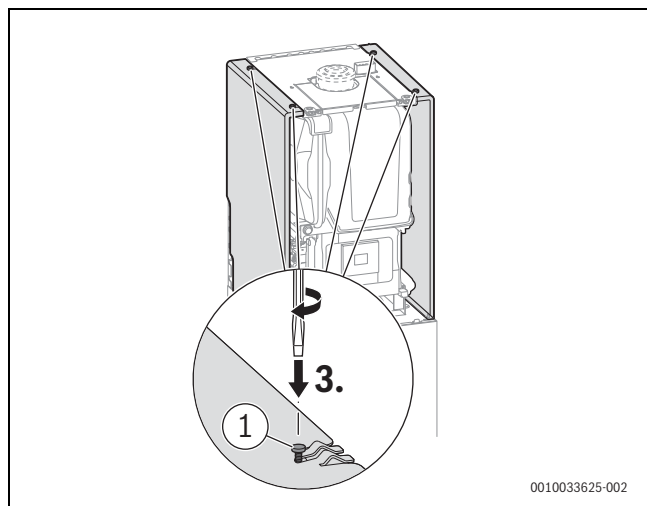
Fig. 87 Fixer les panneaux latéraux de l'habillage
