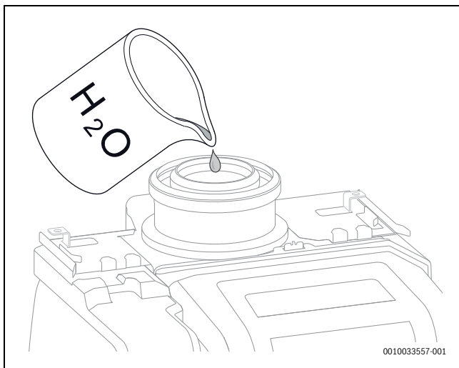
Fig. 70 Remplir le siphon des condensats avec de l'eau
