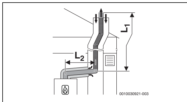
Fig. 29 Évacuation des fumées flexible selon C 93x dans le conduit et circuit d'air et de fumées concentrique dans le local d'installation
