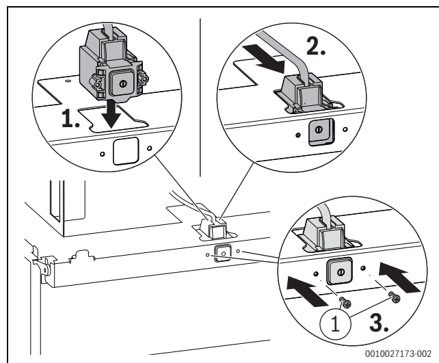
Fig. 77 Fixer l'interrupteur Marche/Arrêt
