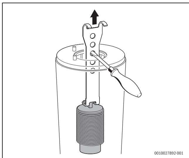
Fig. 119 Retirer le déflecteur inférieur
