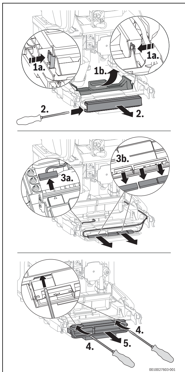
Fig. 140 Retirer l'appareil de commande
