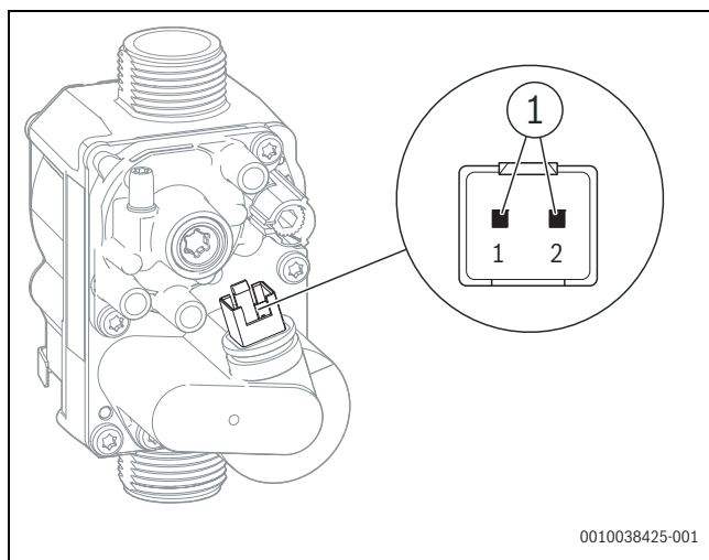
Fig. 110 Points de mesure du bloc gaz
