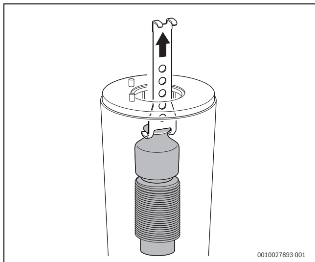
Fig. 118 Retirer le déflecteur supérieur
