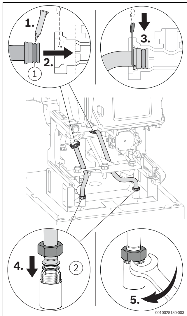
Fig. 60 Raccorder le tube de départ et le tube retour au ballon à serpentin
