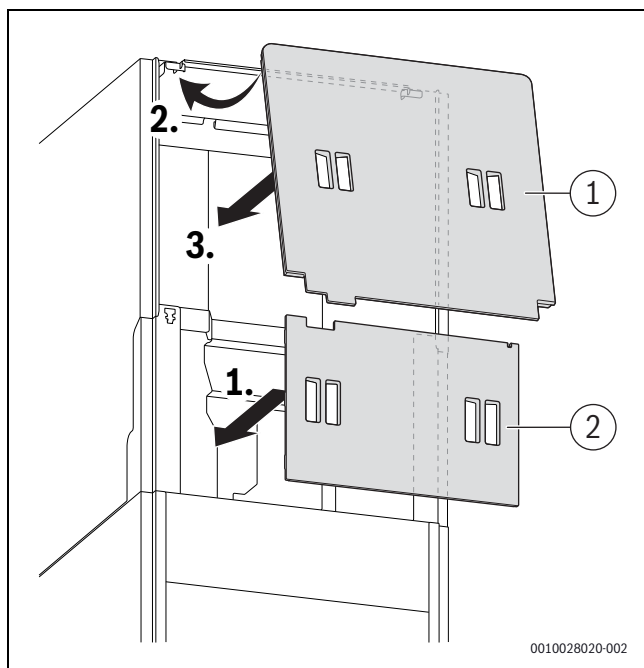
Fig. 91 Fixer l'isolation thermique à l'arrière de l'appareil (accessoire SF 13)
