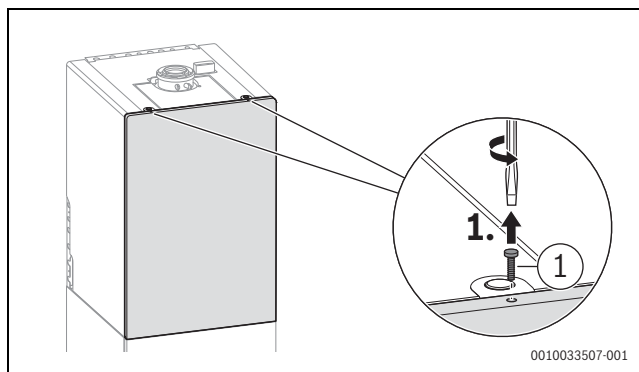
Fig. 105 Desserrer la vis de sécurité
