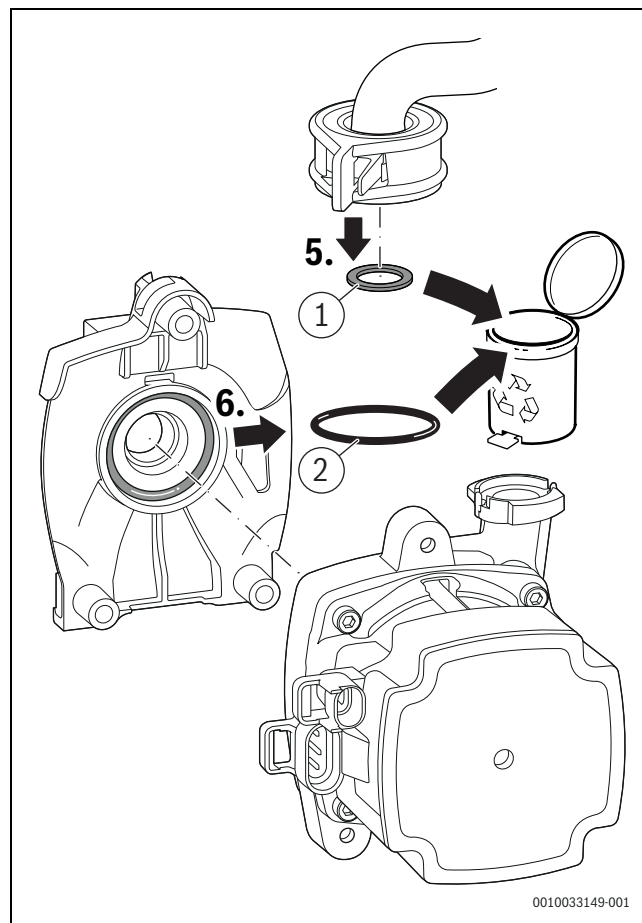
Fig. 131 Éliminer les joints
