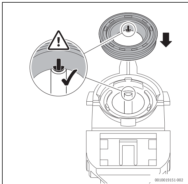
Fig. 142 Alignement du nouveau joint sur le siphon de condensats
