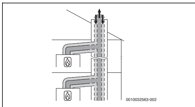
Fig. 34 Raccordement de plusieurs foyers selon C_{(10)3x} avec circuit d'air et de fumées concentrique dans le local d'installation
