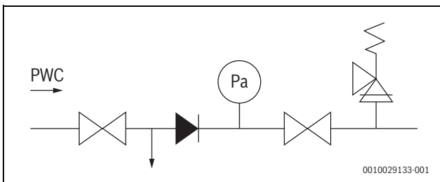
Fig. 66 Exemple : groupe de sécurité pour l'expansion de l'eau selon EN 1488
