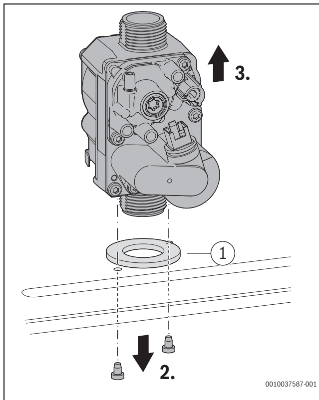
Fig. 135 Démontage du bloc gaz
