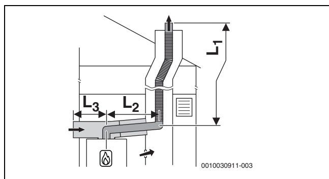
Fig. 26 Conduite d'évacuation des fumées flexible selon C 53x dans le conduit et circuit d'air et de fumées avec alimentation d'air séparée et conduite d'évacuation des fumées concentrique dans le local d'installation
