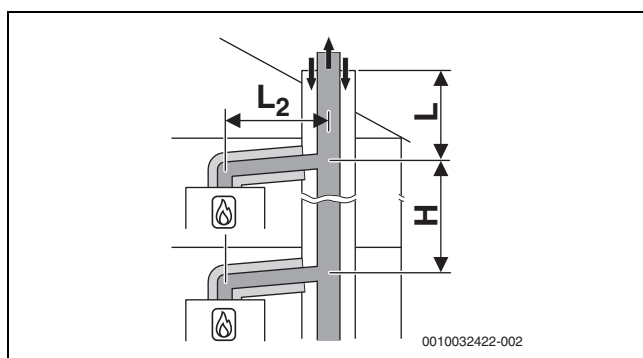
Fig. 38 Raccordement de plusieurs foyers selon C (14)3x avec évacuation des fumées rigide collective et circuit d'air et de fumées concentrique dans le local d'installation
