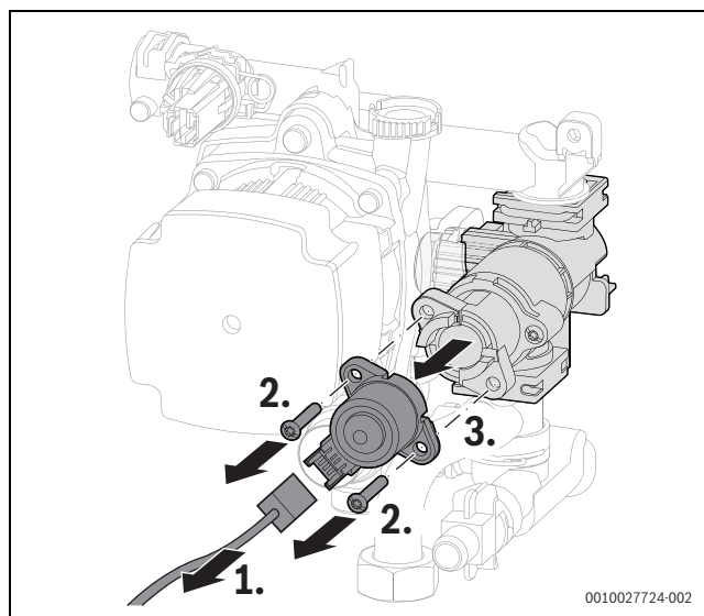
Fig. 145 Démonter le moteur de la vanne sélective
