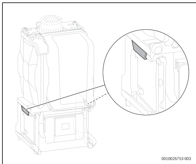
Fig. 56 Soulever l'appareil par les endroits colorés en gris et le transporter vers le ballon
