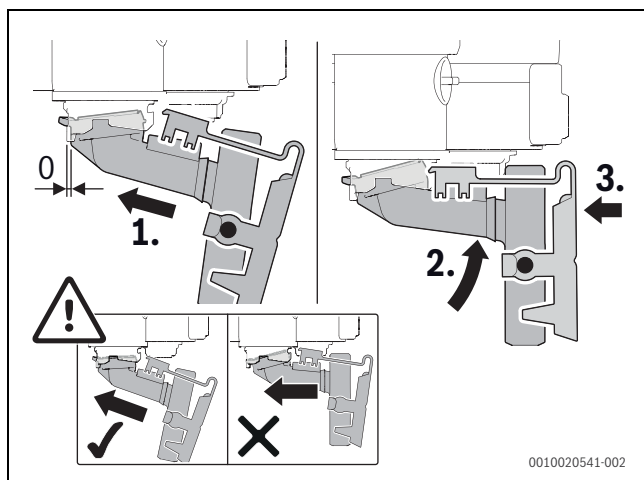
Fig. 62 Remplacer le siphon de condensats et vérifier la bonne fixation
