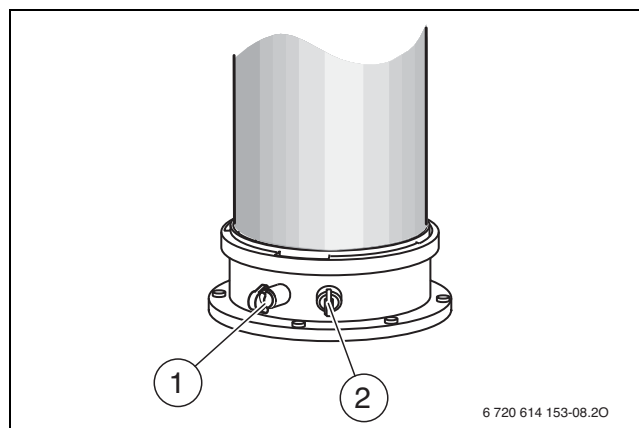
Fig. 102 Tubulure de mesure des fumées et de l'air de combustion
