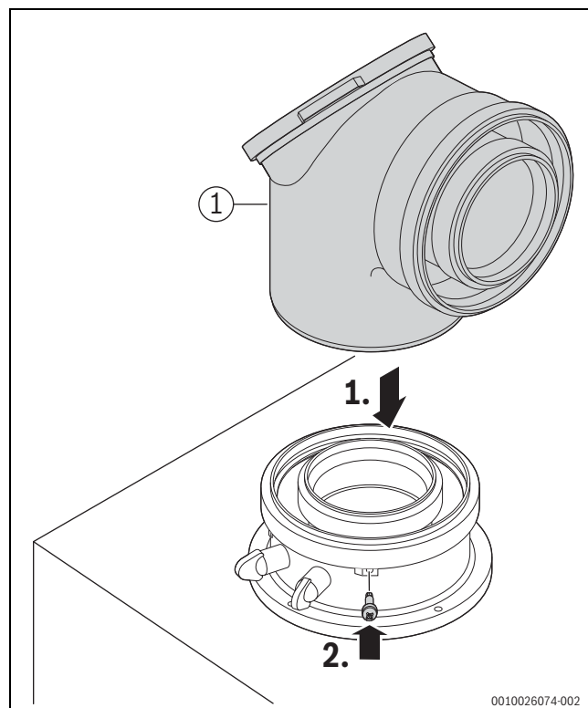
Fig. 71 Insérer les accessoires de fumisterie et fixer avec une vis.
