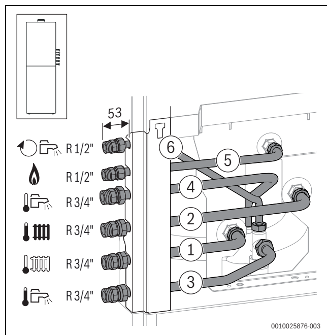
Fig. 52 Accessoire CS 10 monté sur le côté droit
