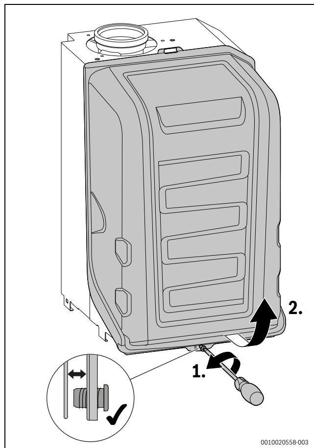
Fig. 74 Retirer le capot du brûleur
