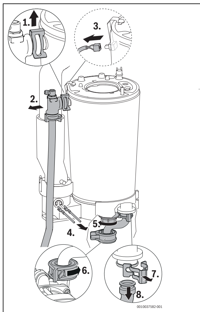
Fig. 126 Détacher le tube de départ, retirer le câble et détacher le tube retour
