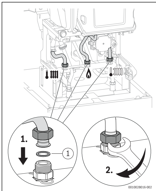
Fig. 61 Raccorder le départ chauffage, le tuyau de gaz, le retour chauffage
