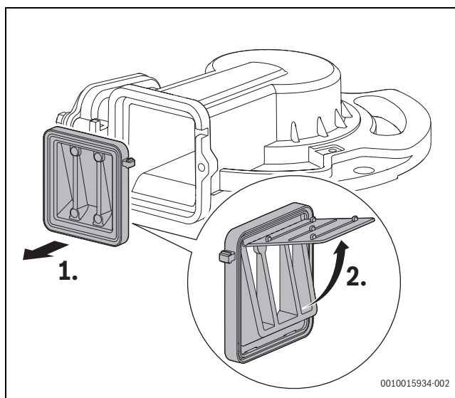
Fig. 116 Sécurité anti-refoulement du dispositif de mélange
