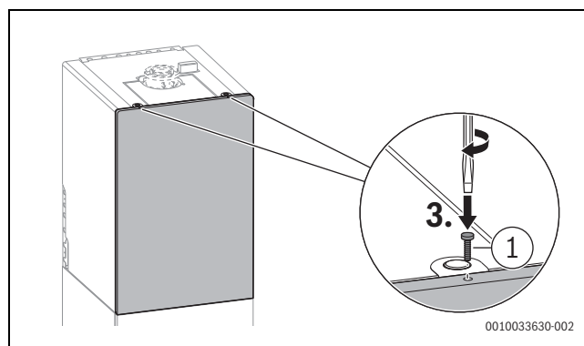
Fig. 89 Fixer le panneau avant de l'habillage avec une vis du contenu de la livraison
