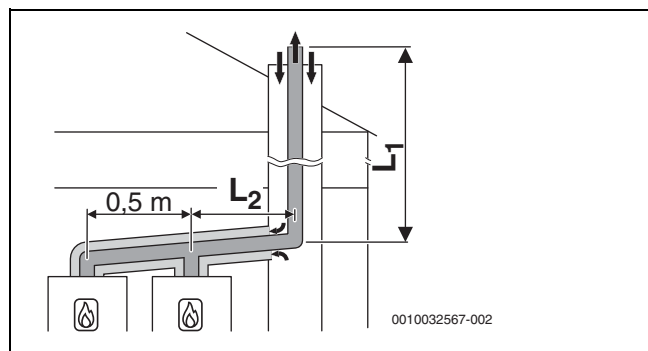
Fig. 41 Cascade avec 2 appareils : Evacuation des fumées rigide selon C 93x dans la gaine technique et circuit d'air et de fumées concentrique dans le local d'installation
