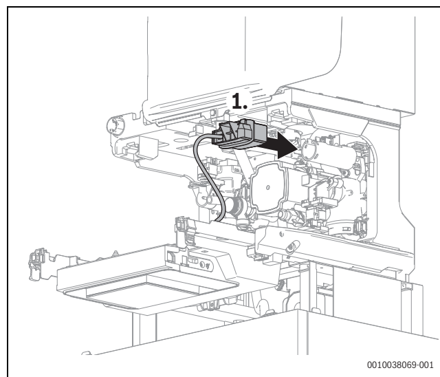
Fig. 63 Conduire le support Key sur la partie arrière de l'appareil
