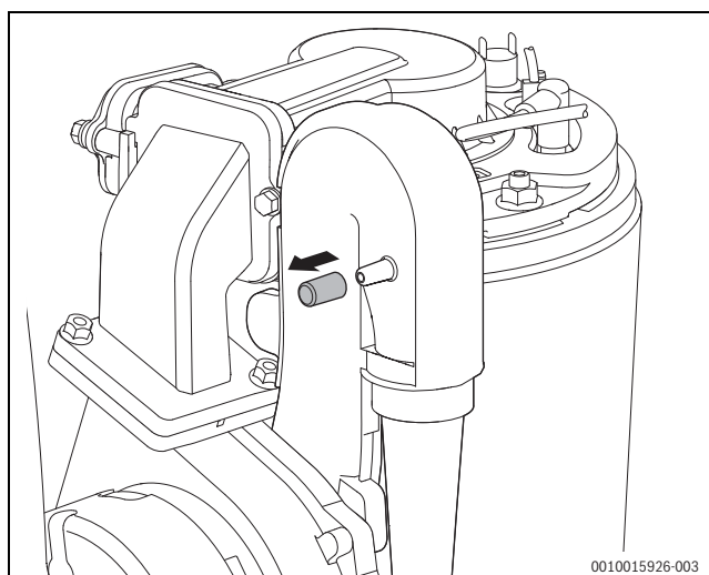
Fig. 109 Tubulure de mesure sur le dispositif de mélange
