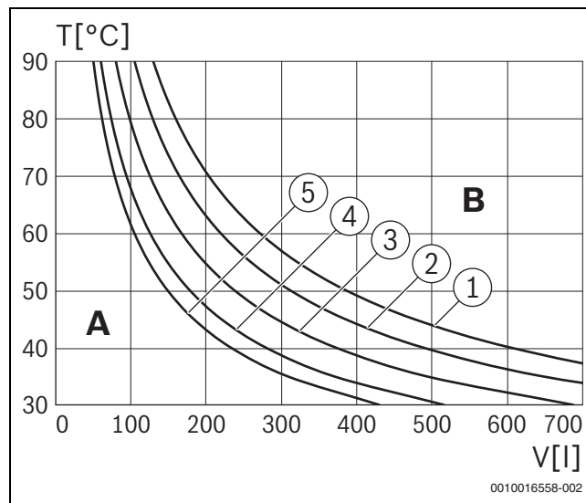
Fig. 45 Courbes caractéristiques pour le vase d'expansion (12 l)
