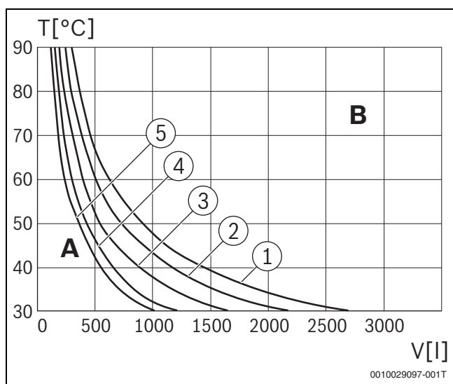
Fig. 47 Courbes caractéristiques pour le vase d'expansion (29 l)
