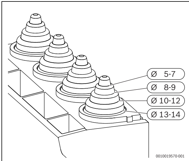
Fig. 81 Adaptation du serre-câbles au diamètre du câble
