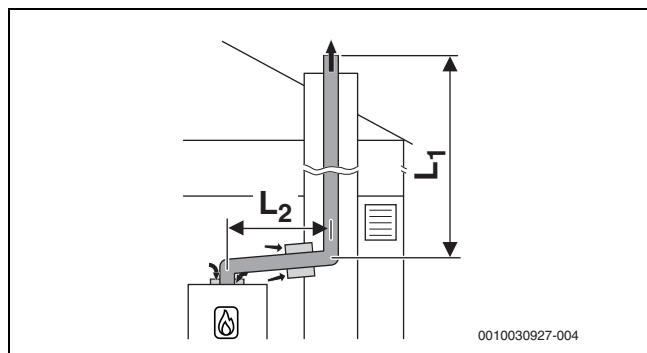
Fig. 30 Évacuation des fumées rigide dans le conduit selon B 53p avec alimentation d'air dépendant de l'air ambiant sur l'appareil et pièce de raccordement concentrique entre le local d'installation et le conduit
