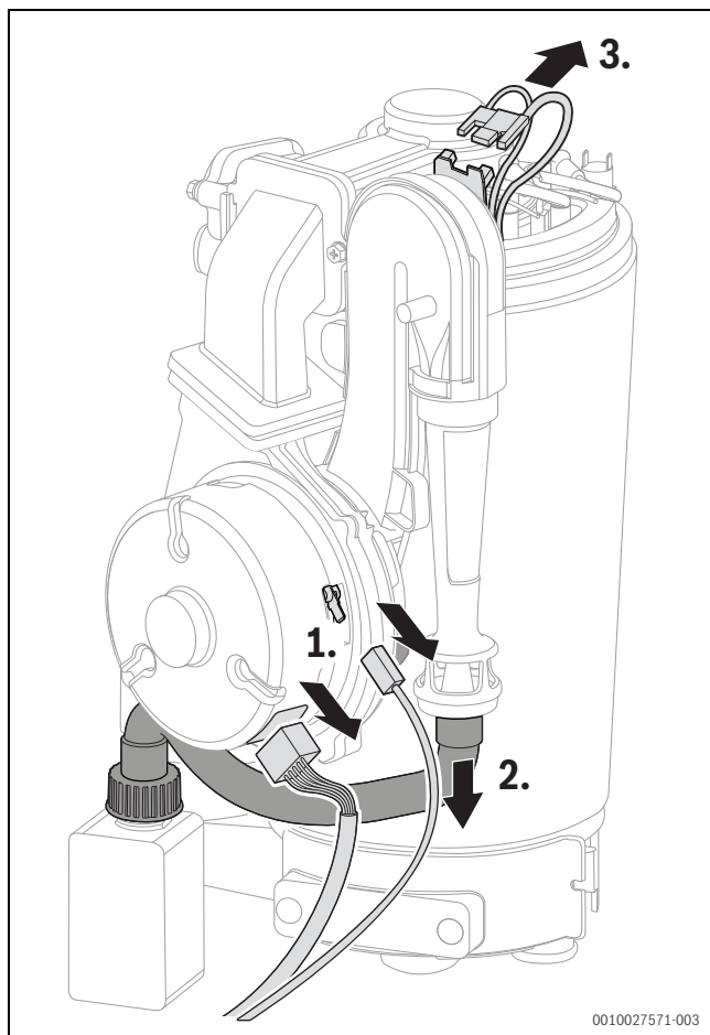
Fig. 111 Débrancher le connecteur et le tuyau de gaz
