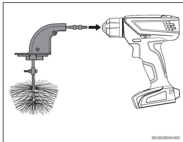
Fig. 121 Raccordement de la brosse avec le tournevis sans fil
