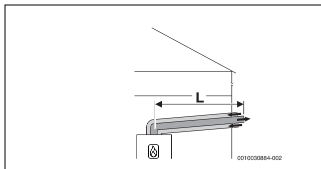
Fig. 21 Circuit d'air et de fumées concentrique horizontal selon C 13x par le mur extérieur
