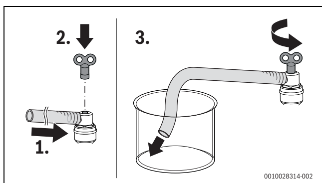
Fig. 75 Purger le circuit d'eau chaude sanitaire et le circuit de chauffage
