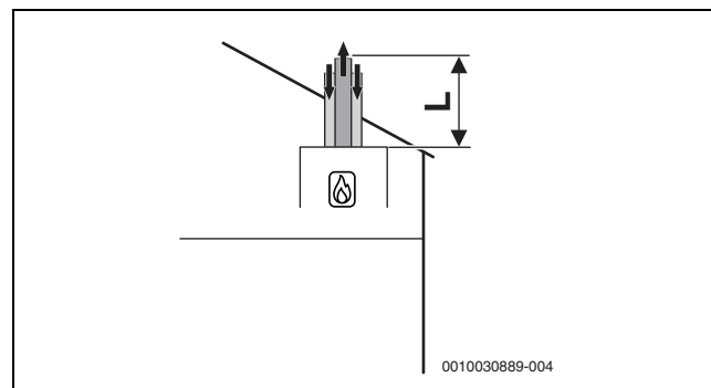
Fig. 24 Circuit d'air et de fumées vertical concentrique selon C 33x
