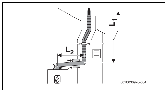
Fig. 32 Évacuation des fumées flexible dans le conduit selon B 53p avec alimentation d'air dépendant de l'air ambiant sur l'appareil et pièce de raccordement concentrique entre le local d'installation et le conduit
