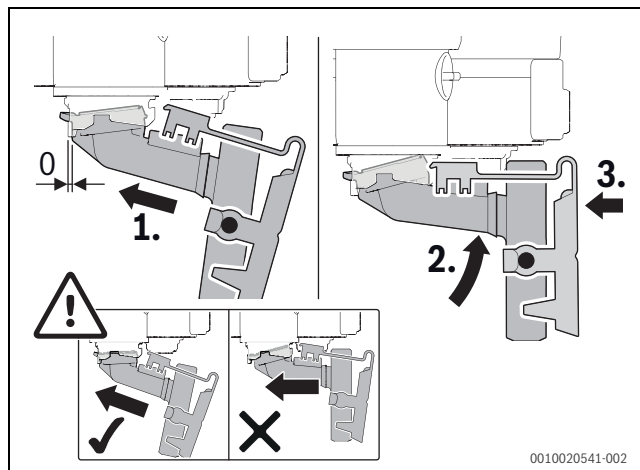
Fig. 144 Monter le siphon de condensats
