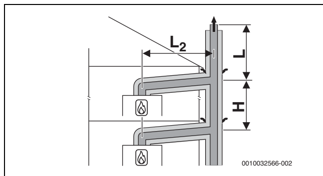
Fig. 37 Raccordement de plusieurs foyers selon C (13)3x avec circuit d'air et de fumées concentrique sur le mur extérieur et dans le local d'installation
