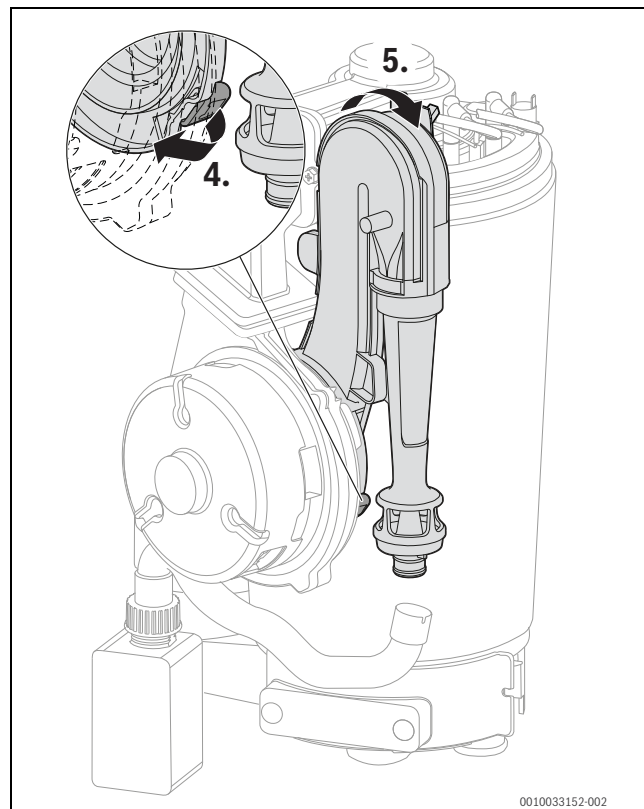
Fig. 112 Démontage du tube Venturi
