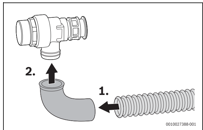
Fig. 67 Raccorder le tube à la soupape de sécurité
