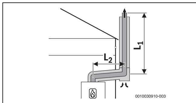
Fig. 27 Circuit d'air et de fumées concentrique selon C 53x sur le mur extérieur
