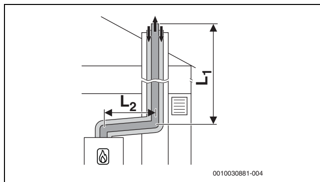
Fig. 23 Circuit d'air et de fumées concentrique selon C 33x dans le conduit
