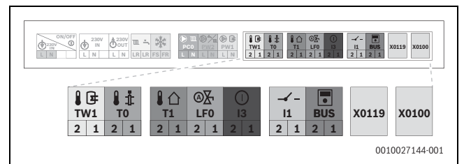
Fig. 83 Plage de basse tension : bornier
