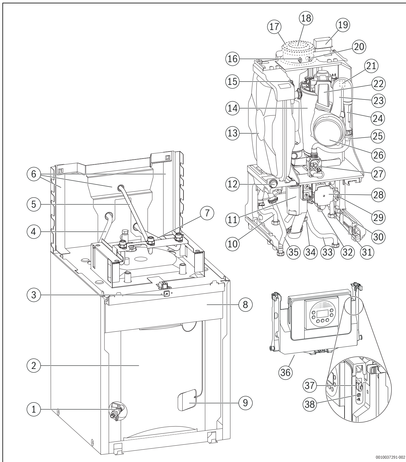
Fig. 5 Aperçu produit
