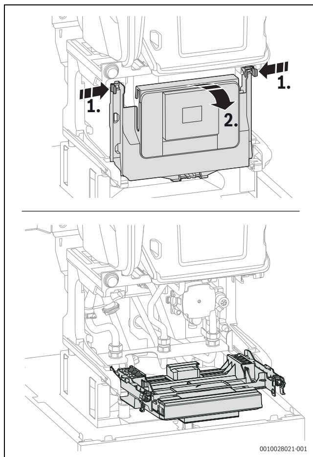
Fig. 108 Rabattre l'appareil de commande
