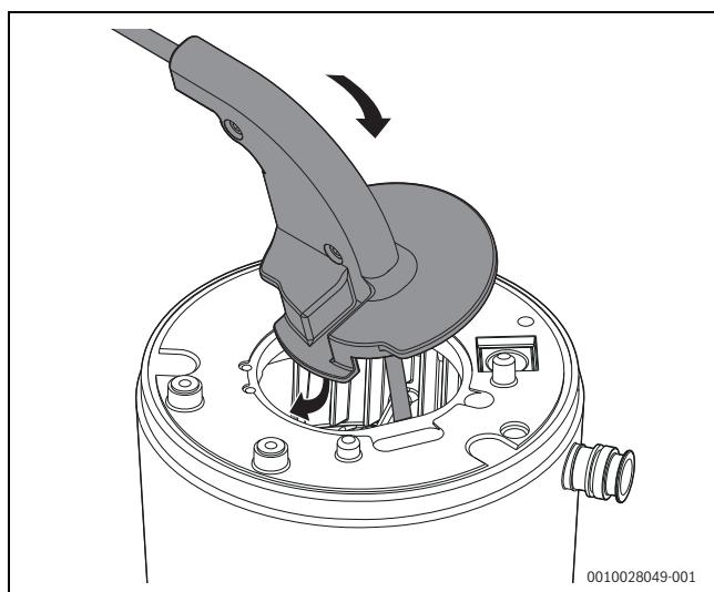
Fig. 120 Insertion de la brosse dans le corps de chauffe
