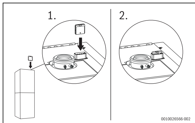
Fig. 72 Insérer le Control Key dans le support du Key
