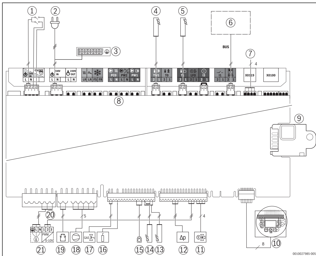
Fig. 148 Câblage électrique
