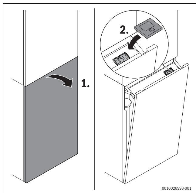
Fig. 73 Monter le module de commande CW 400
