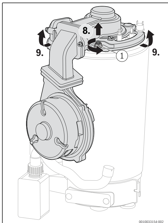
Fig. 114 Retirer le capot de brûleur avec le ventilateur et le dispositif de mélange
