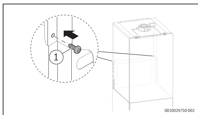
Fig. 90 Visser fermement les panneaux latéraux de l'habillage sur les côtés gauche et droit
