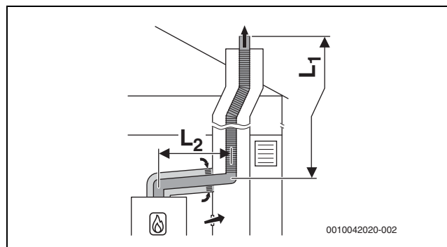
Fig. 33 Évacuation des fumées flexible dans le conduit selon B 53p avec arrivée d'air dépendant de l'air ambiant par le circuit d'air et de fumées concentrique dans le local d'installation
