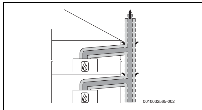
Fig. 36 Raccordement de plusieurs foyers selon C_{(12)3x} avec circuit d'air et de fumées concentrique dans le local d'installation
