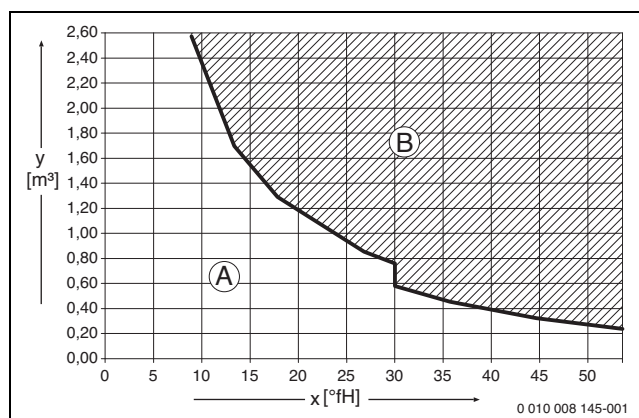
Fig. 44 Conditions requises pour l'eau de remplissage et d'appoint en °fH sur les appareils < 50 kW
