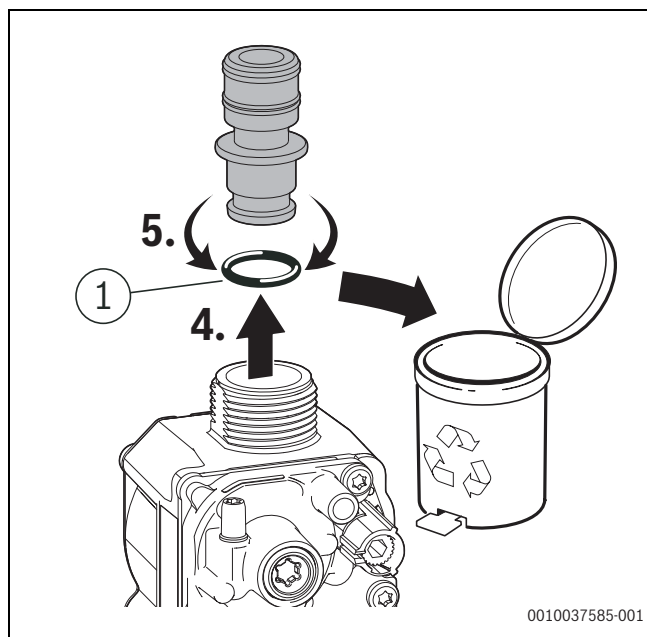
Fig. 133 Retirer l'injecteur
