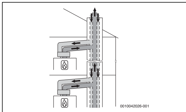
Fig. 35 Raccordement de plusieurs foyers selon C_{(10)3} avec circuit d'air et de fumées avec tubes séparés pour l'alimentation d'air et l'évacuation des fumées dans le local d'installation
