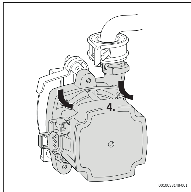
Fig. 130 Retirer la pompe de chaudière par l'avant
