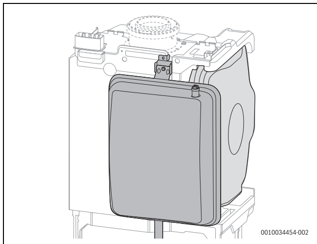
Fig. 46 2 vases d'expansion montés dans l'appareil
