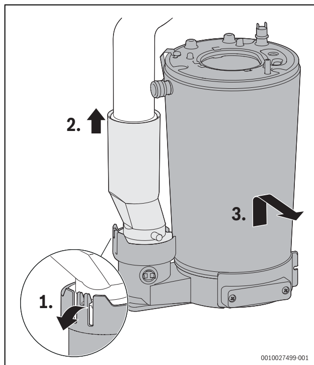
Fig. 127 Démontez le corps de chauffe
