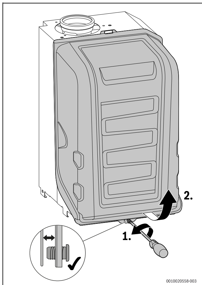
Fig. 99 Retirer le capot du brûleur
