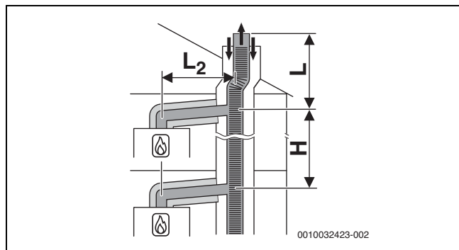
Fig. 39 Raccordement de plusieurs foyers selon C_{(14)3x} avec évacuation des fumées flexible collective et circuit d'air et de fumées concentrique dans le local d'installation
