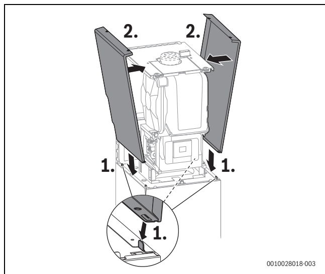
Fig. 86 Mettre en place les panneaux latéraux de l'habillage
