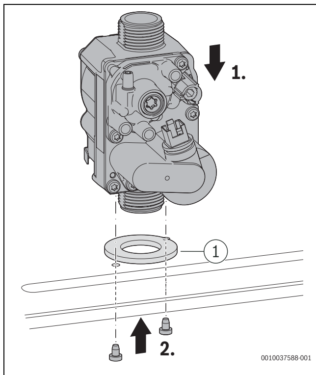
Fig. 136 Installation du bloc gaz
