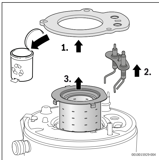
Fig. 117 Retirer le brûleur
