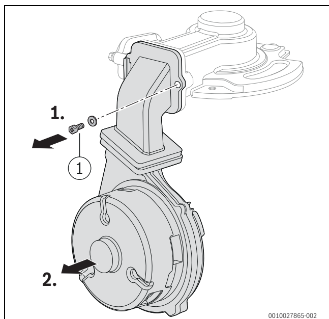
Fig. 115 Démonter le dispositif de mélange et le ventilateur
