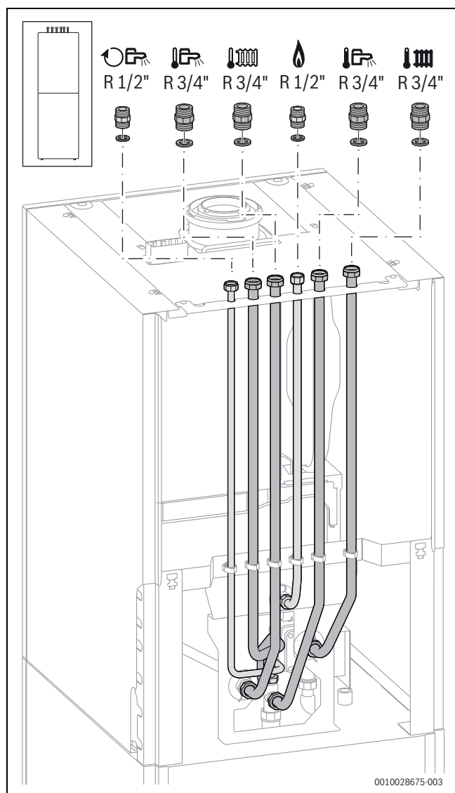
Fig. 53 Accessoire CS 33 monté
