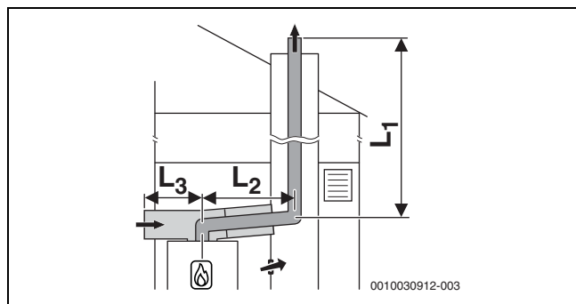
Fig. 25 Conduite d'évacuation des fumées rigide selon C 53x dans le conduit et circuit d'air et de fumées avec alimentation d'air séparée et conduite d'évacuation des fumées concentrique dans le local d'installation
