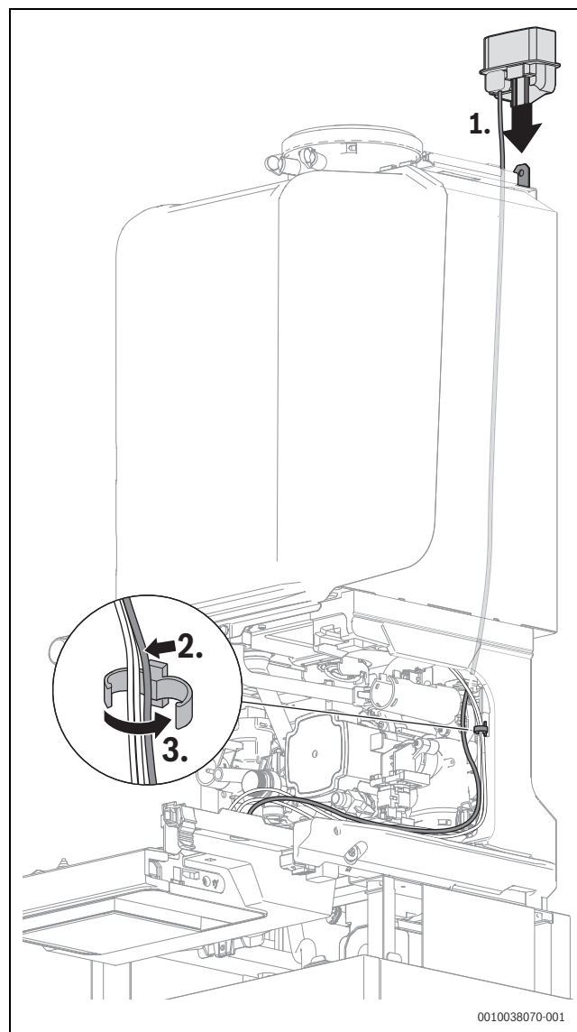
Fig. 64 Insérer le support de Key dans l'emplacement et fixer le câble dans le support de câbles
