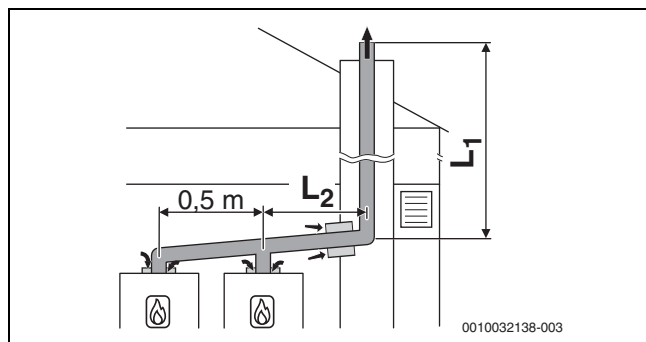
Fig. 40 Cascade avec 2 appareils : évacuation des fumées dans le conduit rigide selon B 53P avec arrivée d'air dépendant de l'air ambiant sur l'appareil
