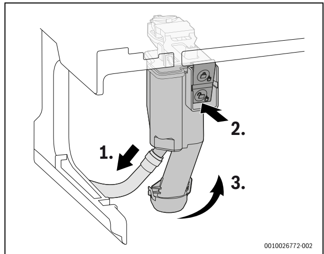
Fig. 141 Démonter le siphon des condensats
