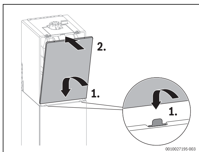
Fig. 88 Mettre en place le panneau avant de l'habillage
