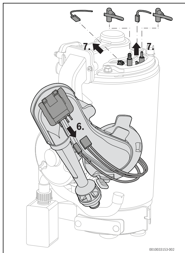
Fig. 113 Retirer le câble
