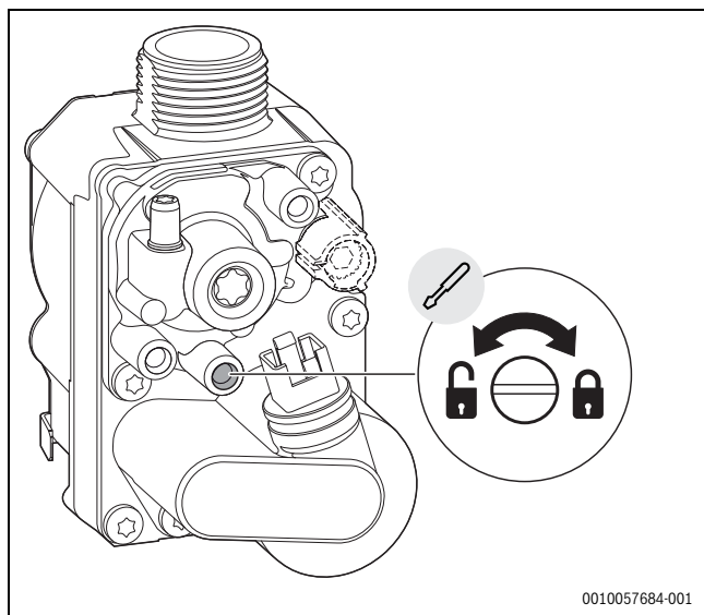
Fig. 100 Mesure de la pression de raccordement du gaz
