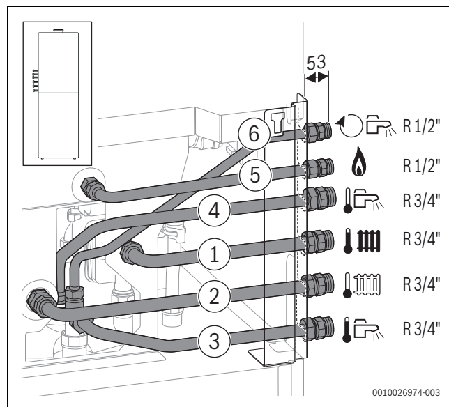
Fig. 51 Accessoire CS 10 monté sur le côté gauche
