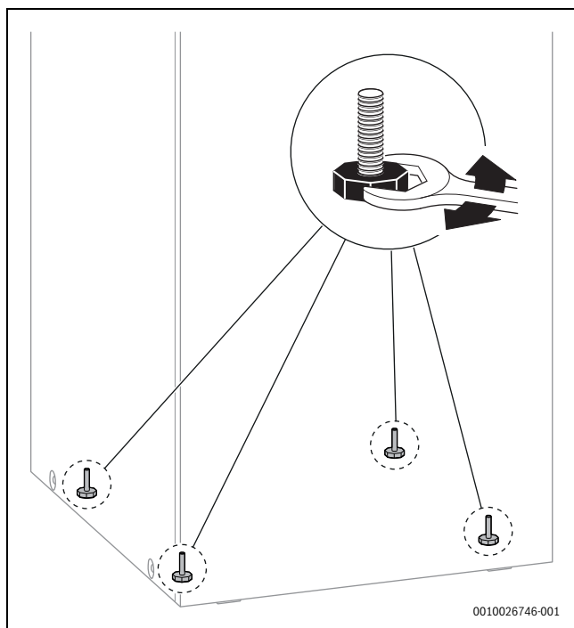
Fig. 92 Sur le lieu d'installation final, les défauts de planéité du sol peuvent être compensés à l'aide des pieds réglables
