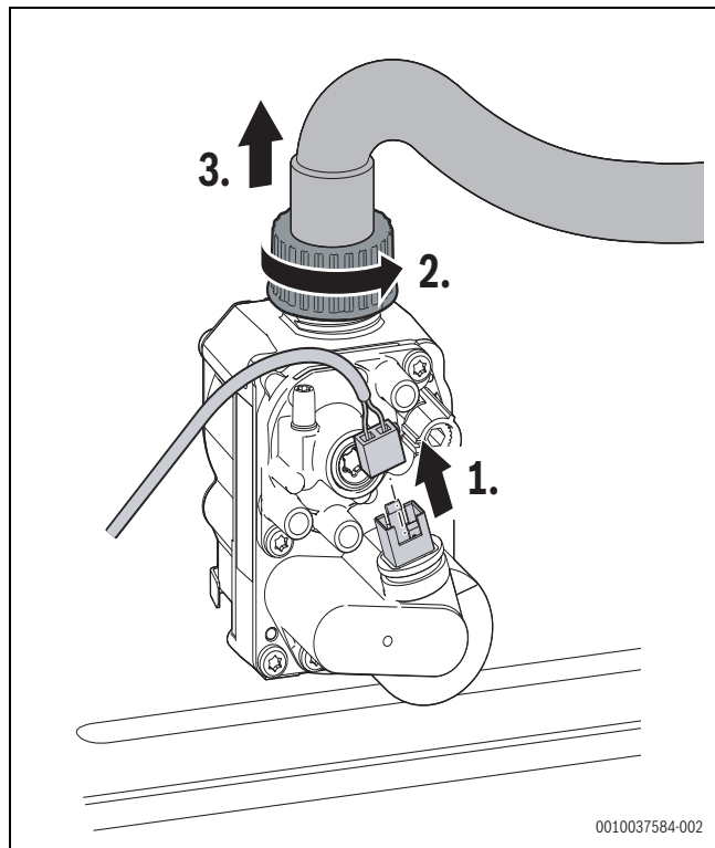
Fig. 132 Retrait du connecteur du bloc gaz et de l'écrou-raccord avec le tuyau du gaz
