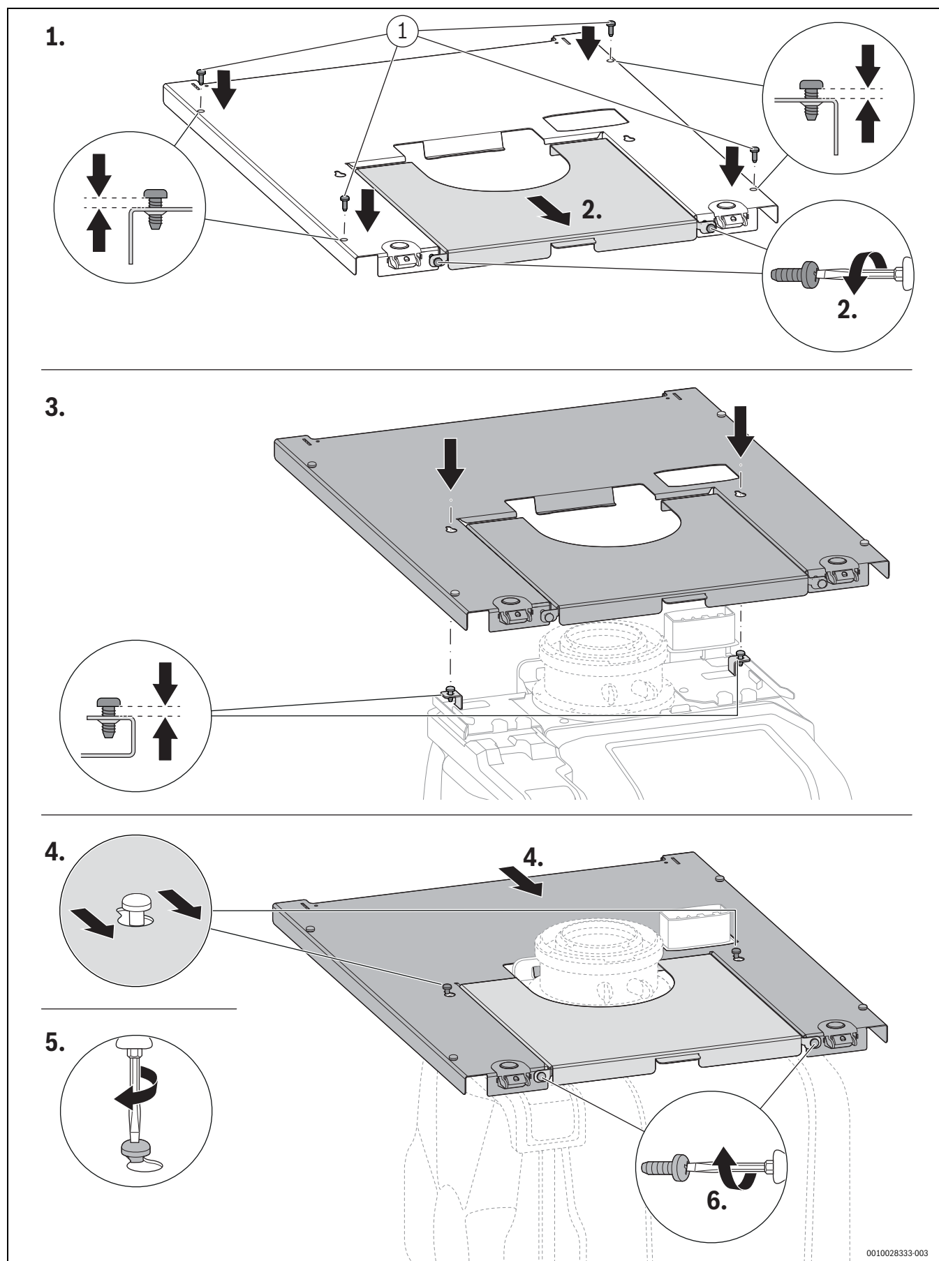
Fig. 85 Fixer la partie supérieure de l'habillage. Si nécessaire, les deux pièces de l'habillage peuvent être montées l'une après l'autre.
