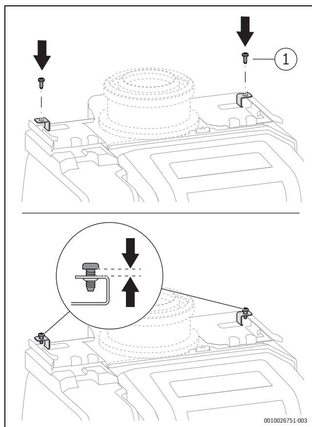
Fig. 54 Visser les vis de la partie supérieure de l'habillage sans trop serrer
