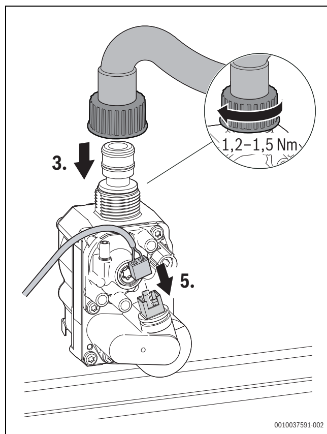
Fig. 139 Raccordement du tuyau du gaz et du connecteur – Respect du couple de serrage
