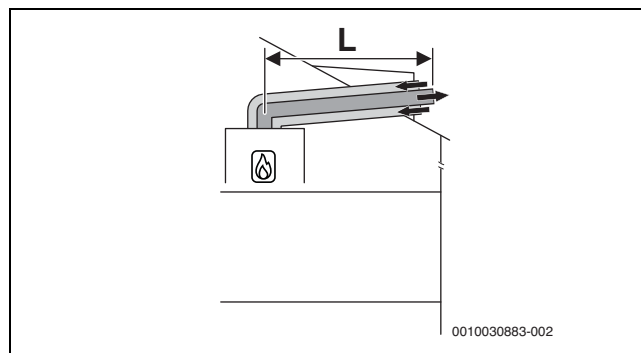
Fig. 22 Circuit d'air et de fumées concentrique horizontal selon C 13x par le toit
