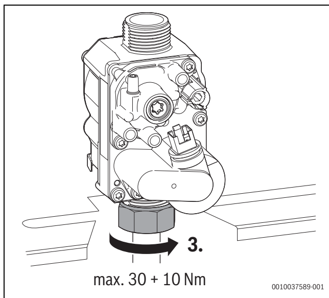
Fig. 137 Respect du couple de serrage
