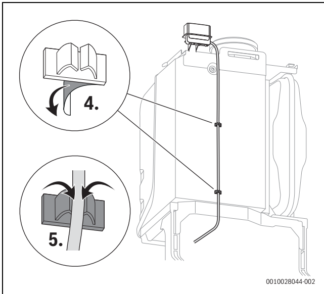
Fig. 65 Fixer le support de câbles à l'arrière de l'appareil et fixer les câbles
