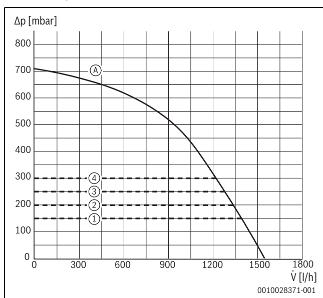
Fig. 149 Diagrammes de pompe et courbes caractéristiques de pompe (24 kW)
