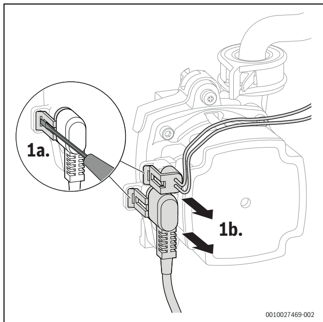
Fig. 128 Débrancher le connecteur de la pompe de chaudière
