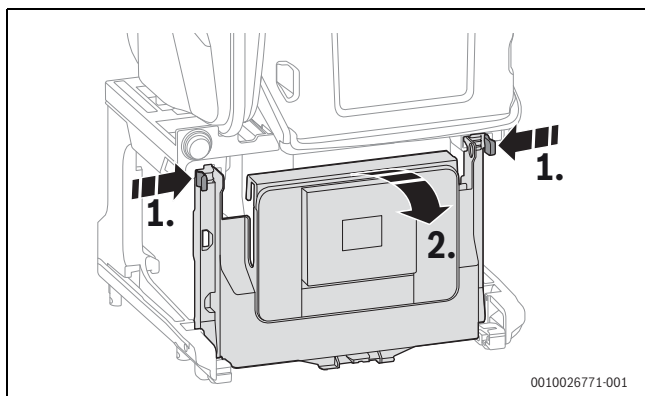
Fig. 58 Rabattre le boîtier de commande
