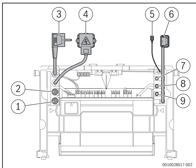
Fig. 80 État à la livraison de l'appareil de commande avec composants raccordés
