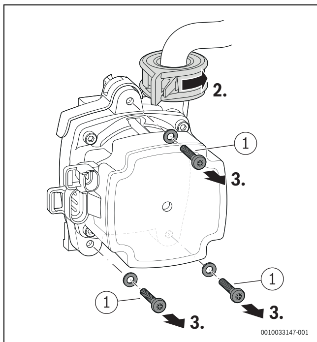
Fig. 129 Déverrouiller la pompe de chaudière et retirer les vis
