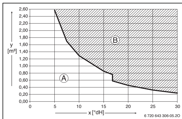
Fig. 43 Conditions requises pour l'eau de remplissage et d'appoint en °dH sur les appareils < 50 kW
