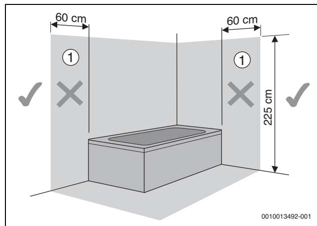
Fig. 42 Volumes de protection
