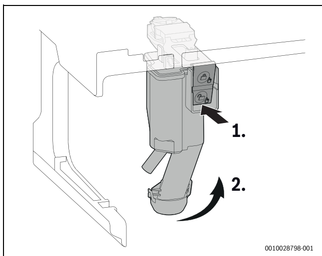
Fig. 59 Retrait du siphon de condensats
