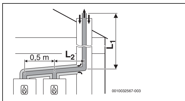
Fig. 22 Cascade avec 2 appareils : Evacuation des fumées rigide selon C 93x dans la gaine technique et circuit d'air et de fumées concentrique dans le local d'installation
