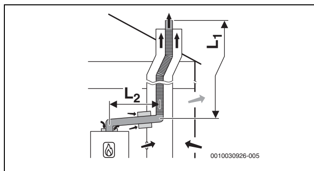
Fig. 16 Évacuation des fumées flexible dans le conduit selon B 53p avec alimentation d'air dépendant de l'air ambiant sur l'appareil ; ouverture de ventilation dans le conduit
