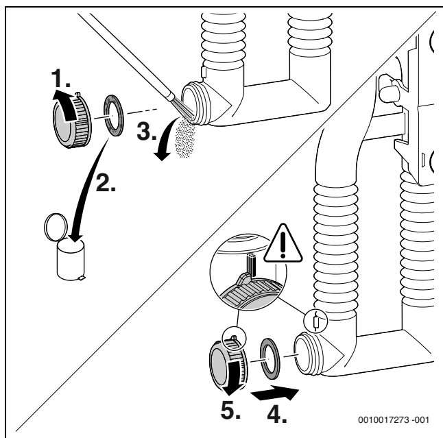
Fig. 45 Nettoyage du siphon de condensats
