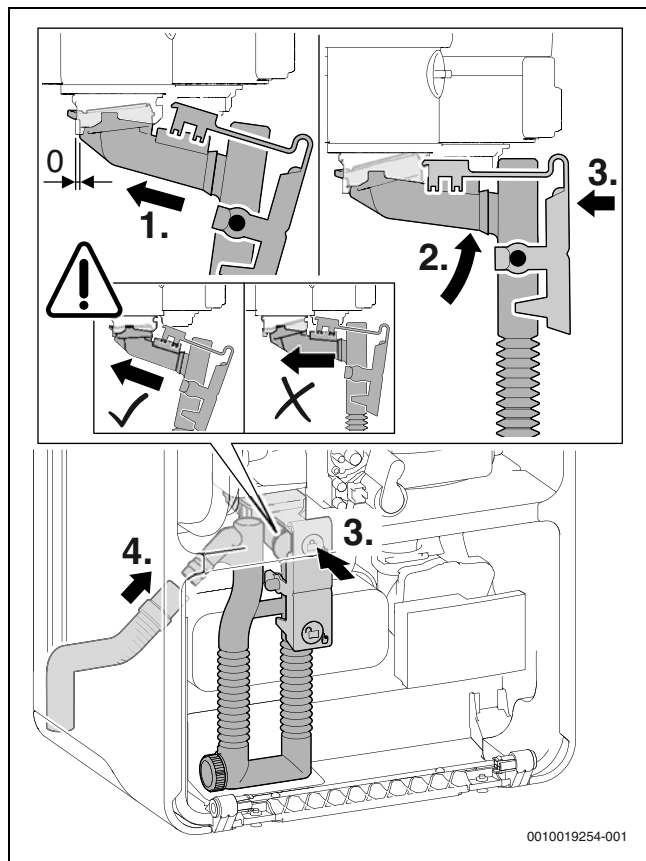
Fig. 49 Insertion du siphon de condensats
