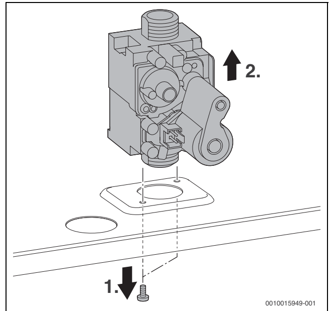
Fig. 54 Démontage du bloc gaz
