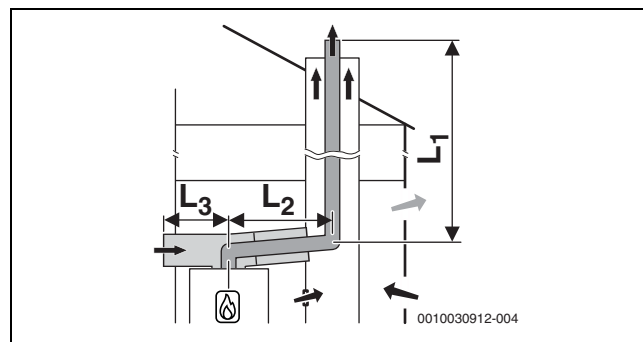
Fig. 8 Évacuation des fumées rigide selon C 53x dans le conduit technique et circuit d'air et de fumées avec alimentation d'air séparée et conduite d'évacuation des fumées concentrique dans le local d'installation
