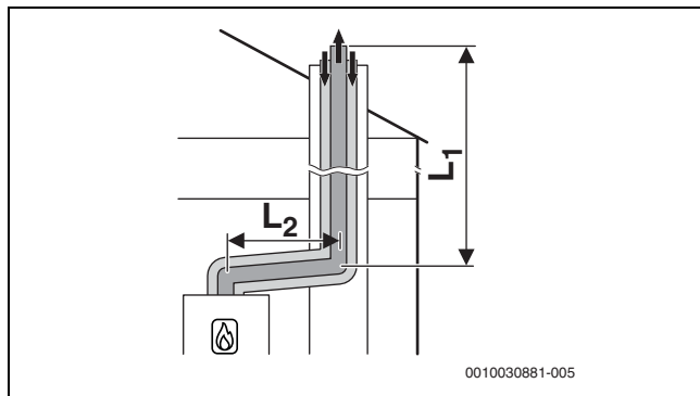
Fig. 5 Circuit d'air et de fumées concentrique selon C 33x dans le conduit
