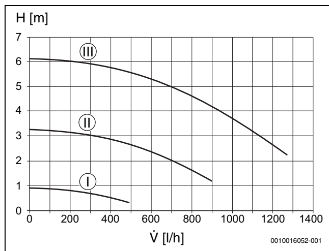
Fig. 31 Courbe caractéristique de la pompe de chauffage (vitesse de rotation constante)
