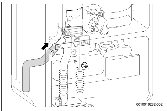
Fig. 28 Monter le tuyau sur le siphon des condensats
