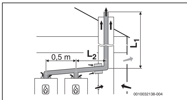
Fig. 21 Cascade avec 2 appareils : évacuation des fumées dans le conduit rigide selon B 53p avec arrivée d'air dépendant de l'air ambiant sur l'appareil ; le conduit avec ouverture de ventilation
