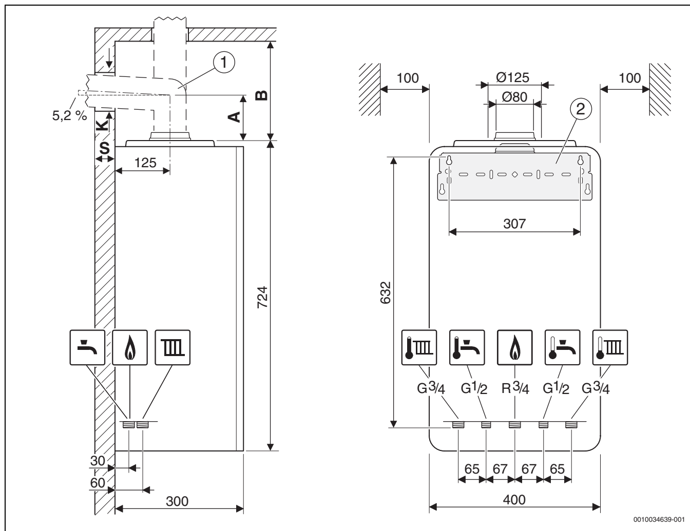
Fig. 1 Dimensions et distances minimums (mm)
