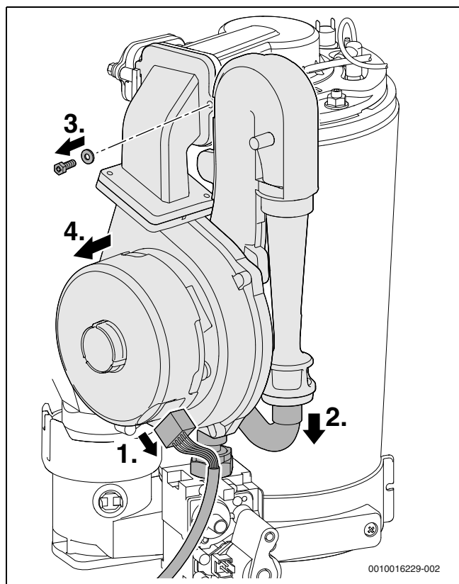
Fig. 35 Démontage du ventilateur avec le dispositif de mélange
