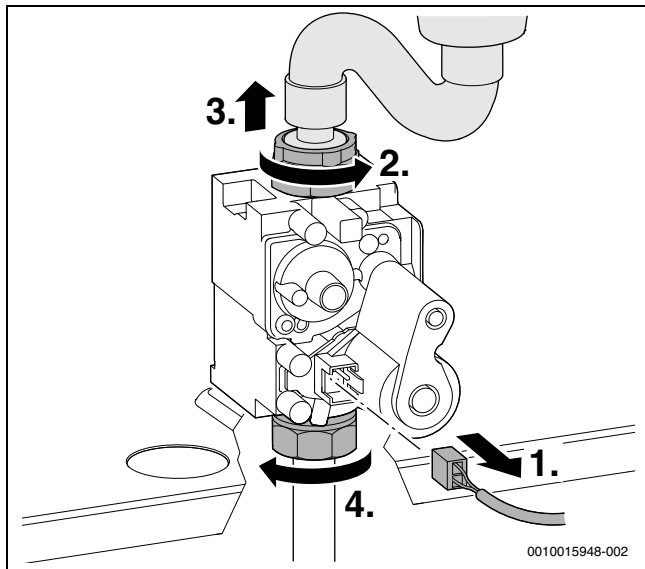
Fig. 53 Retrait du connecteur et desserrage des écrous-raccords
