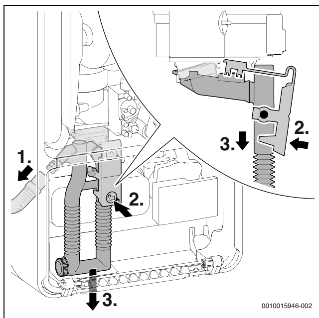
Fig. 44 Démontez le siphon des condensats
