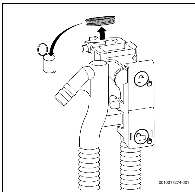
Fig. 46 Retrait du joint en haut sur le siphon de condensats
