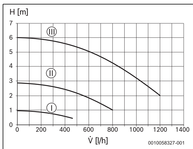
Fig. 32 Courbe caractéristique de la pompe de chaudière (pression constante)
