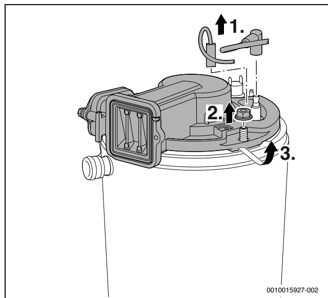
Fig. 36 Détacher le couvercle du brûleur
