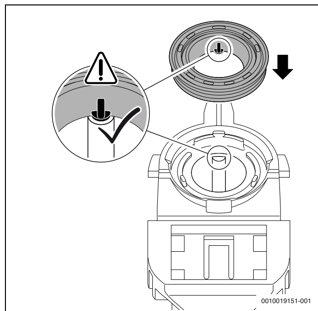
Fig. 47 Alignement du nouveau joint sur le siphon de condensats
