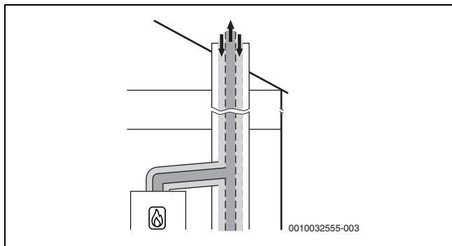
Fig. 7 Circuit d'air et de fumées concentrique selon C 43x dans le local d'installation
