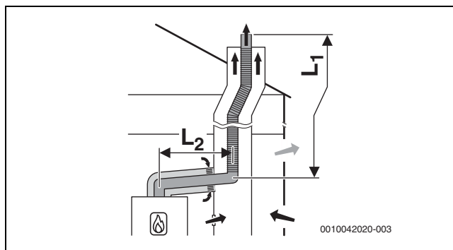
Fig. 14 Évacuation des fumées flexible dans le conduit selon B_{53p} avec arrivée d'air dépendant de l'air ambiant par le circuit d'air et de fumées concentrique dans le local d'installation ; ouverture de ventilation dans le conduit
