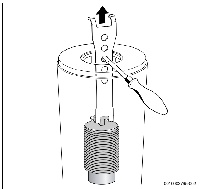
Fig. 40 Retirer la masse de déplacement inférieur
