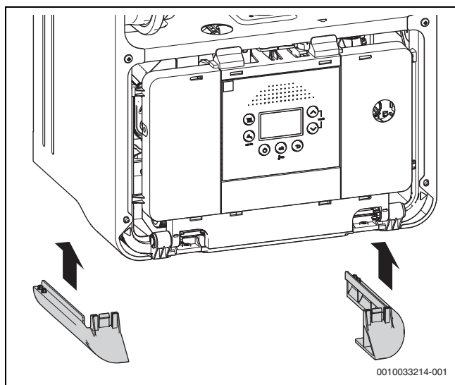
Fig. 61 Mise en place des baguettes latérales en plastique
