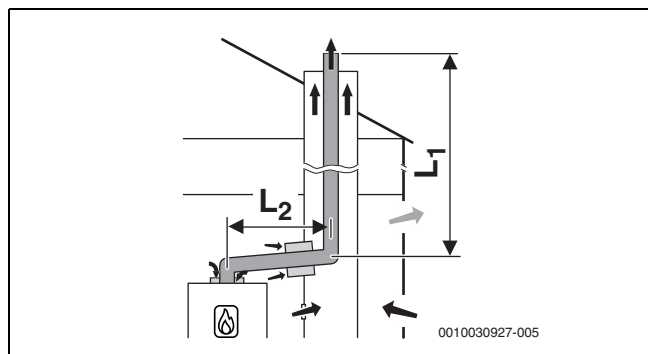
Fig. 15 Évacuation des fumées rigide dans le conduit selon B 53p avec alimentation d'air dépendant de l'air ambiant sur l'appareil ; ouverture de ventilation dans le conduit
