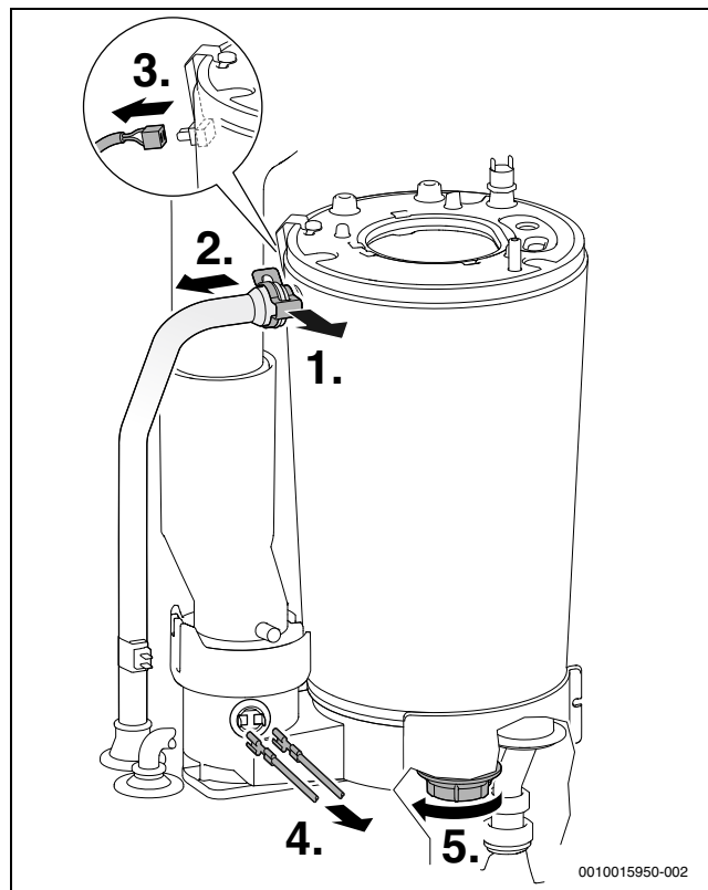
Fig. 58 Détacher le tuyau de départ et retirer le câble
