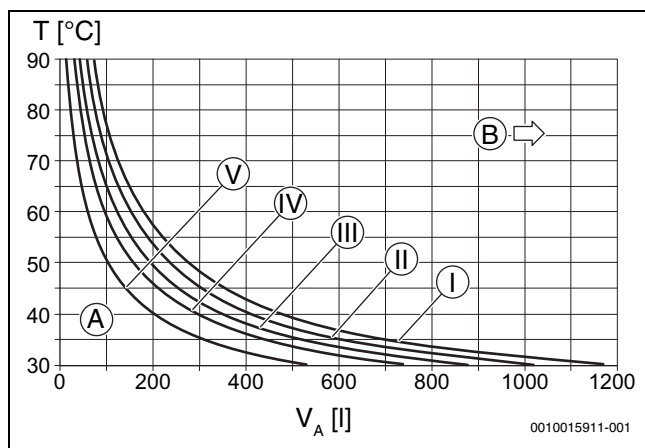
Fig. 25 Courbes caractéristiques du vase d'expansion
