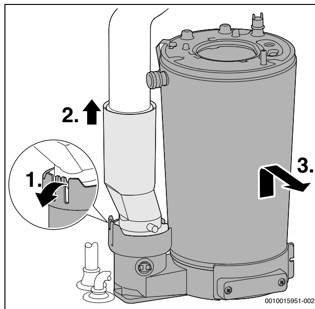
Fig. 59 Démontez le corps de chauffe
