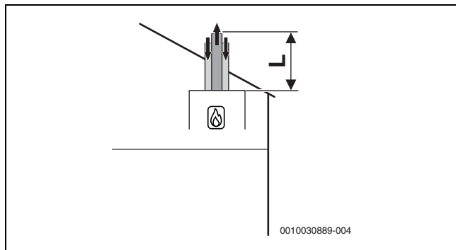
Fig. 6 Circuit d'air et de fumées vertical concentrique selon C 33x par le toit
