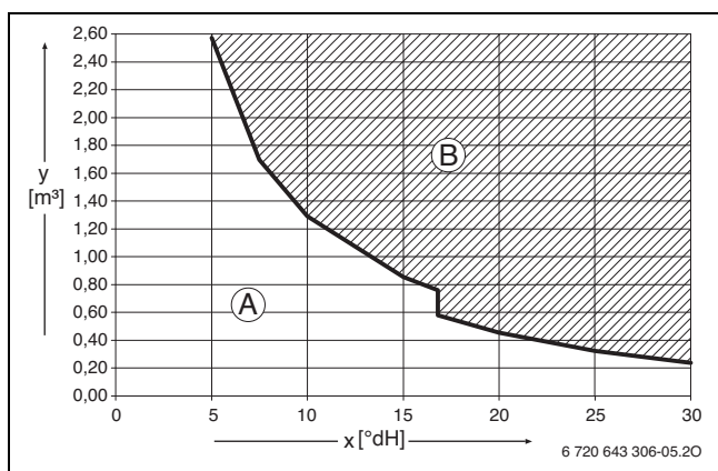
Fig. 23 Conditions requises pour l'eau de remplissage et d'appoint en °dH sur les appareils < 50 kW
