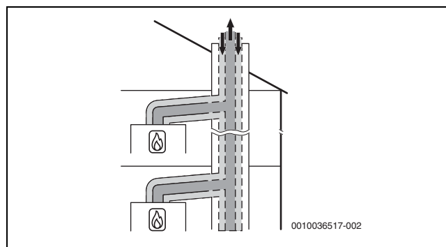
Fig. 17 Raccordement de plusieurs foyers selon C 43p avec circuit d'air et de fumées concentrique dans le local d'installation
