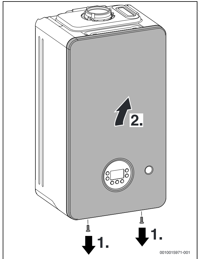
Fig. 26 Retirer l'habillage avant.
