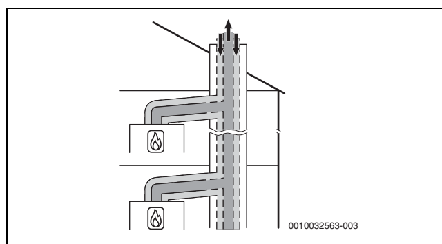
Fig. 18 Raccordement de plusieurs foyers selon C (10)3x avec circuit d'air et de fumées concentrique dans le local d'installation
