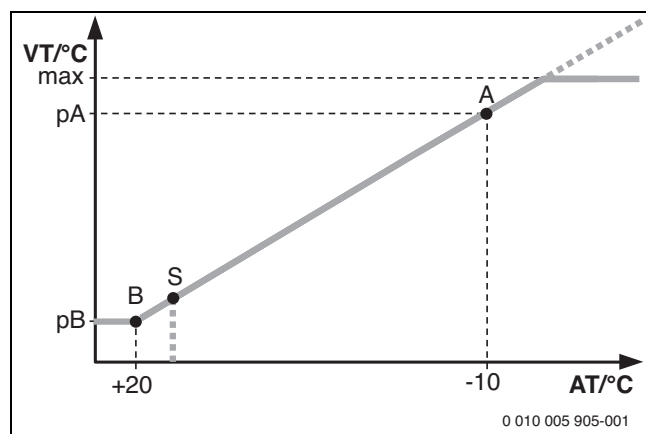
Fig. 63 Courbe de chauffe
