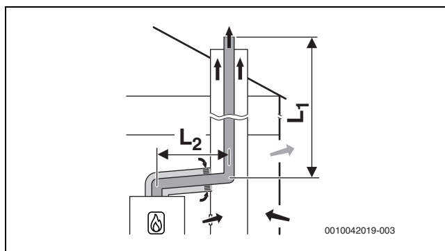
Fig. 13 Évacuation des fumées rigide dans le conduit selon B_{53p} avec amenée d'air dépendant de l'air ambiant par la conduite de raccordement concentrique dans le local d'installation ; ouverture de ventilation dans le conduit.
