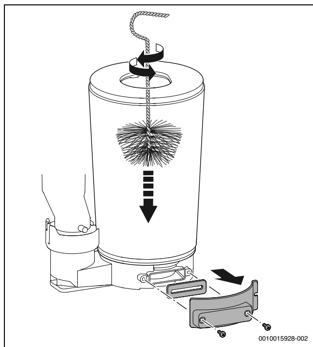
Fig. 41 Nettoyer le corps de chauffe
