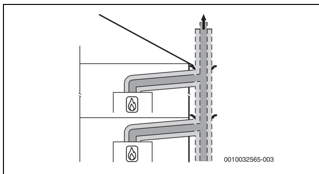
Fig. 19 Raccordement de plusieurs foyers selon C (12)3x avec circuit d'air et de fumées concentrique dans le local d'installation
