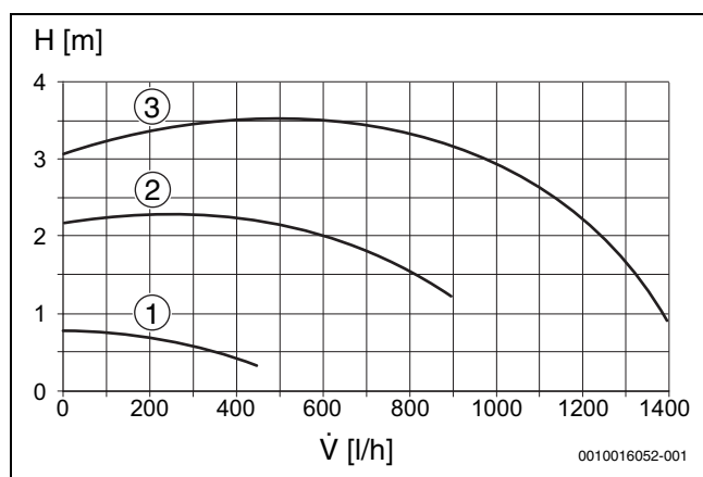
Fig. 33 Courbe caractéristique de la pompe de chauffage (pression proportionnelle)
