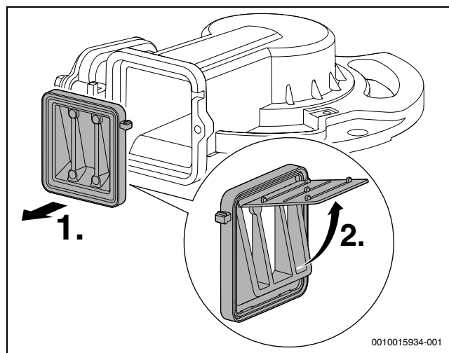
Fig. 37 Clapet anti-retour du dispositif de mélange
