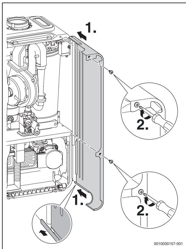
Fig. 60 Mise en place de l'habillage latéral
