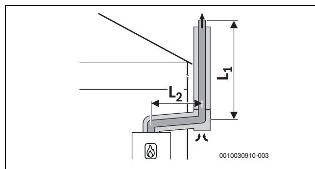
Fig. 9 Circuit d'air et de fumées concentrique selon C 53x sur le mur extérieur
