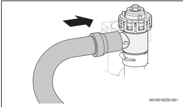
Fig. 27 Monter le flexible sur la soupape de sécurité
