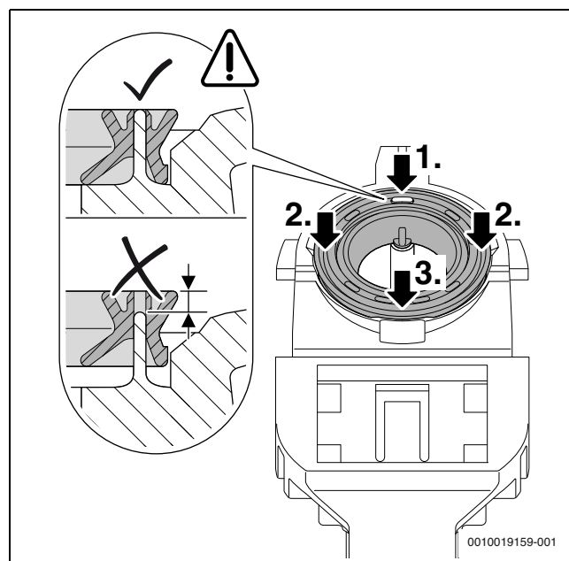
Fig. 48 Appui sur le joint
