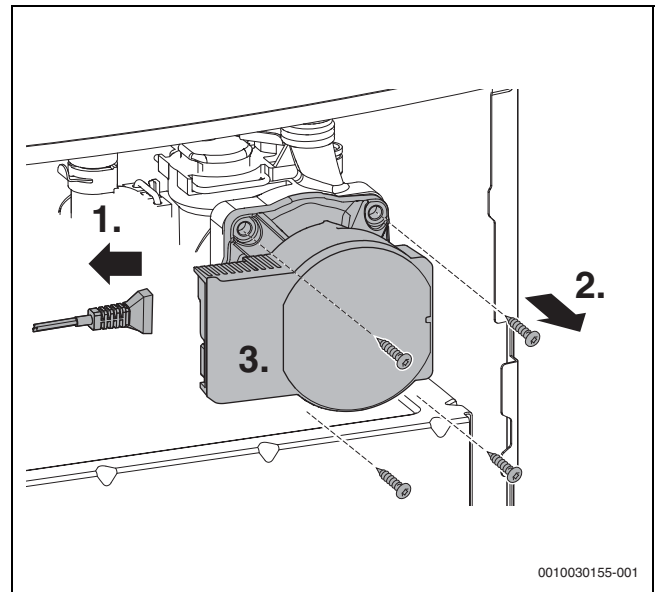
Fig. 55 Démontez la pompe de chauffage
