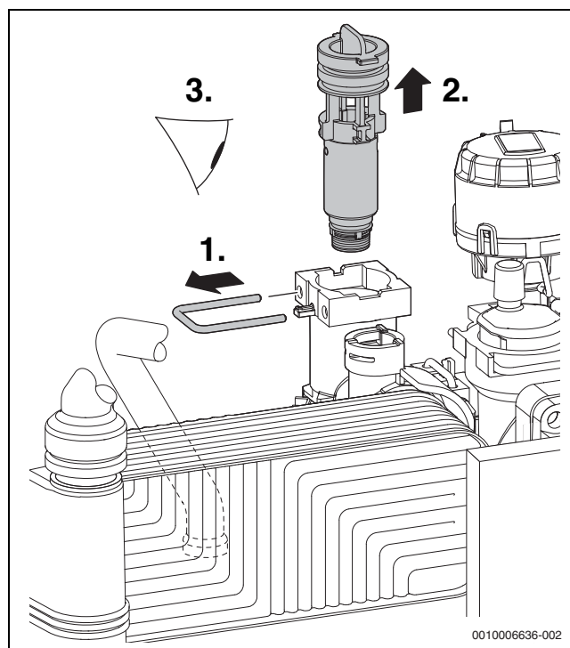
Fig. 51 Contrôle du filtre dans le tuyau d'eau froide
