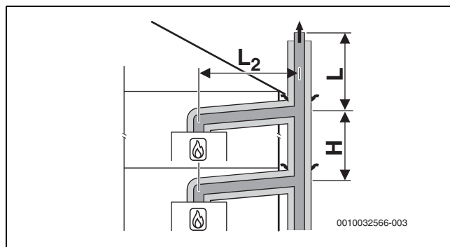
Fig. 20 Raccordement de plusieurs foyers selon C (13)3x avec circuit d'air et de fumées concentrique sur le mur extérieur et dans le local d'installation
