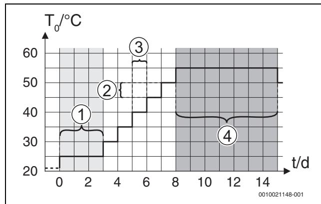
Fig. 6 Déroulement du séchage de dalle avec les réglages de base en phase de mise en température
