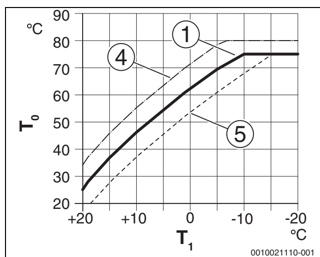
Fig. 5 Réglage de la courbe de chauffage pour radiateur Déplacement parallèle par Offset temp. ambiante ou température ambiante souhaitée
