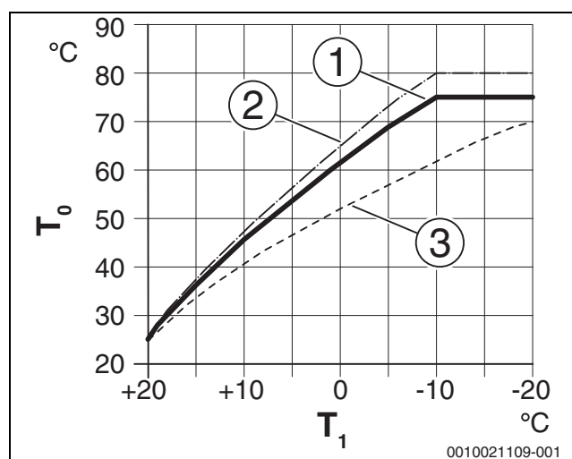
Fig. 4 Réglage de la courbe de chauffage pour radiateur pente ascendante au-dessus de la température de détermination T_0 et température extérieure minimale T_{1,min}
