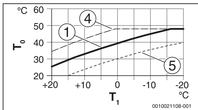
Fig. 3 Réglage de la courbe de chauffage pour chauffage par le sol Déplacement parallèle par Offset temp. ambiante ou température ambiante souhaitée
