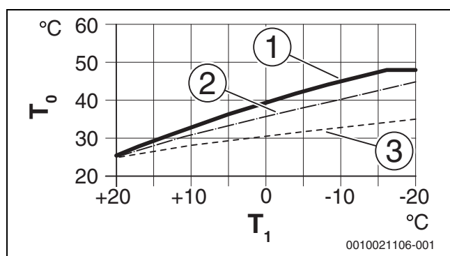
Fig. 2 Réglage de la courbe de chauffage pour chauffage par le sol pente ascendante au-dessus de la température de conception T_0 et température extérieure minimale T_{1,min}
