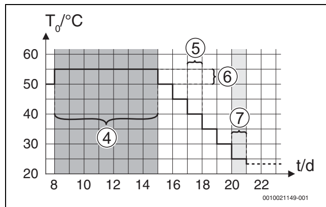
Fig. 7 Déroulement du séchage de dalle avec les réglages de base en phase de refroidissement
