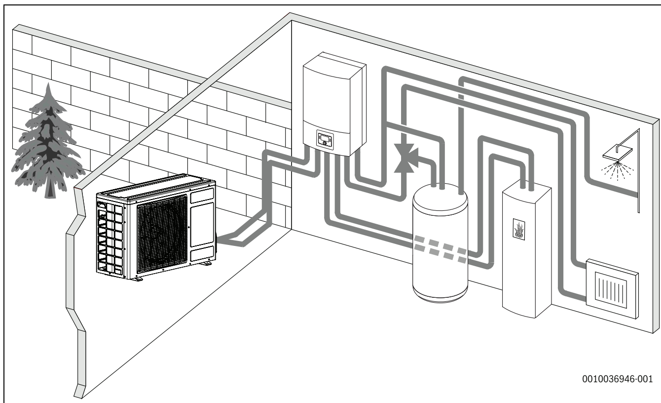
Fig. 2 La pompe à chaleur de l'unité extérieure, l'unité intérieure AWS B sans chauffage d'appoint électrique, le ballon d'eau chaude sanitaire externe et le chauffage d'appoint externe
