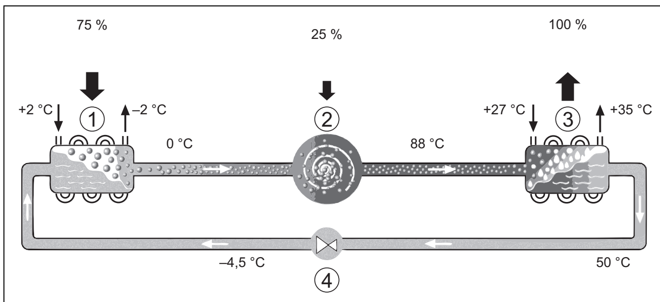
Fig. 1 Principe de fonctionnement du circuit du fluide frigorigène dans la pompe à chaleur
