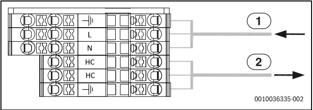
Fig. 16 Bornes de raccordement pour le raccordement électrique
