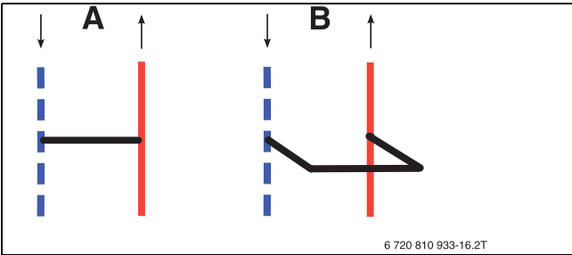
Fig. 36 Bypass [A] By-pass, modèle droit [B] By-pass, modèle en U
