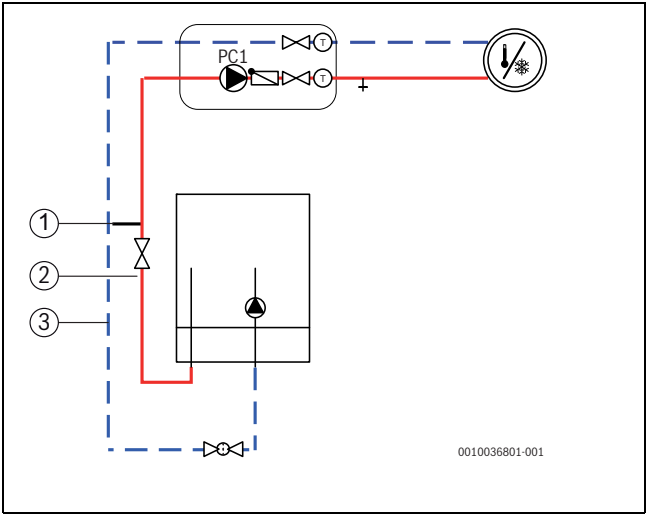
Fig. 33 Unité intérieure avec circuit de chauffage et by-pass
