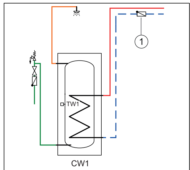
Fig. 21 Ballon d'eau chaude sanitaire
