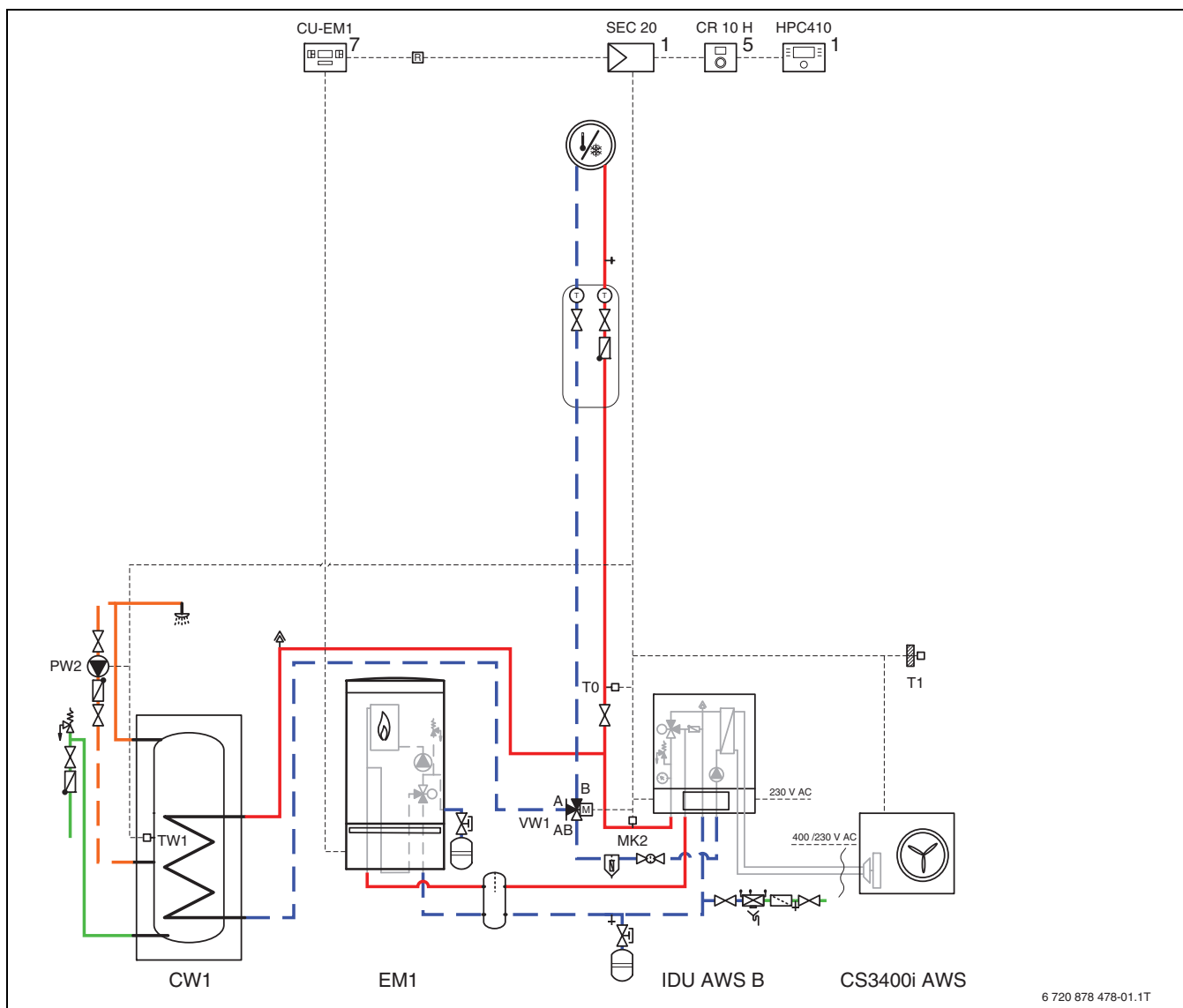
Fig. 37 Unité extérieure avec unité intérieure, chauffage d'appoint externe, ECS et un circuit de chauffage
