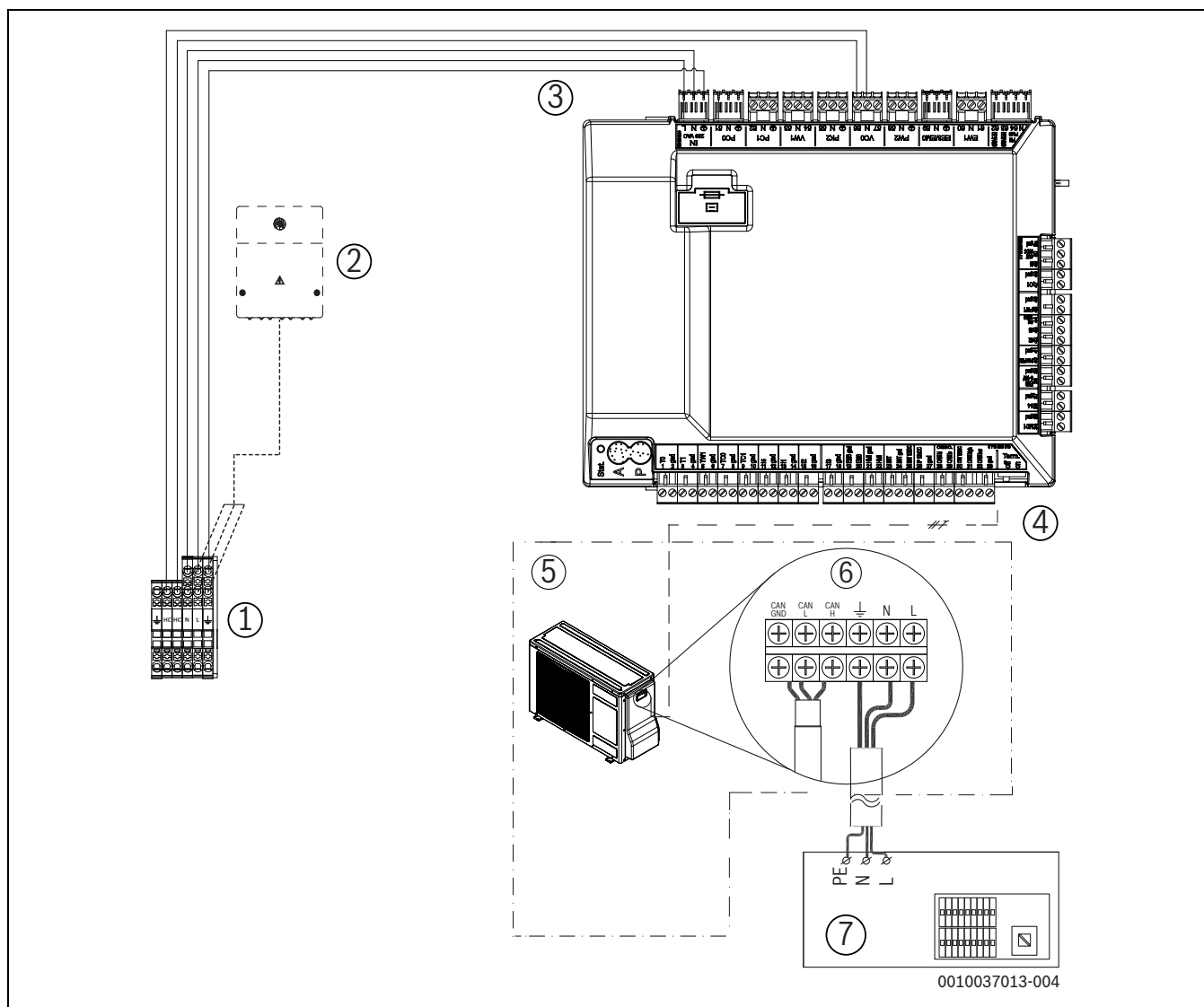
Fig. 43 Unité intérieure avec unité extérieure 230 V~
