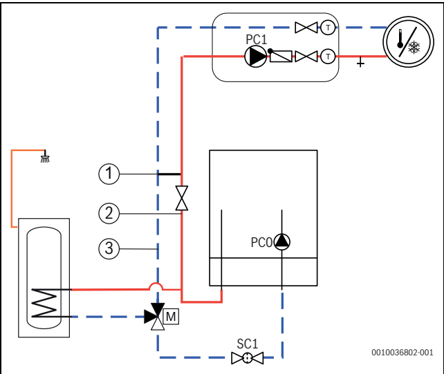
Fig. 34 Unité intérieure avec circuit de chauffage et production d'eau chaude sanitaire
