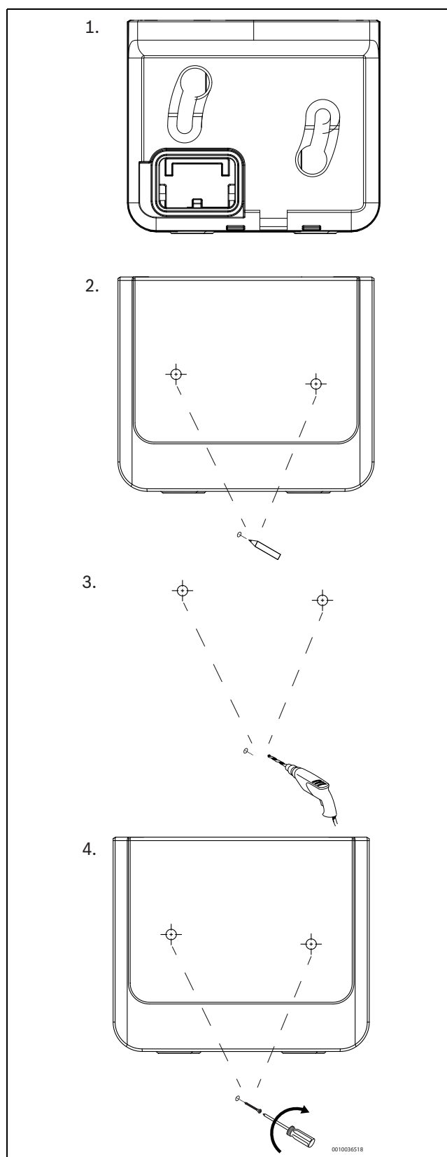
Fig. 31 Monter le support au mur
