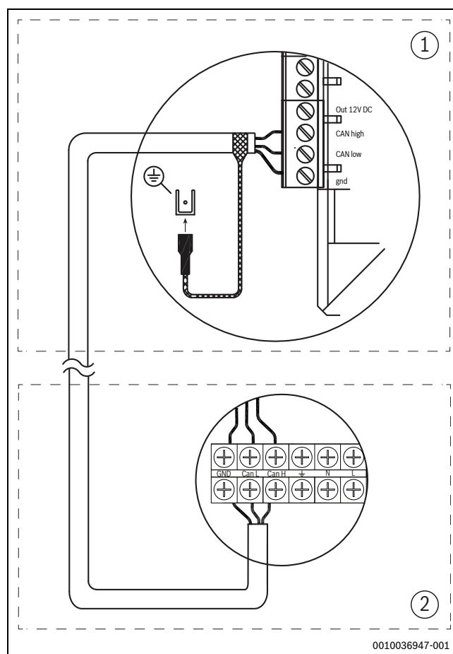
Fig. 12 Connexion CAN-BUS
