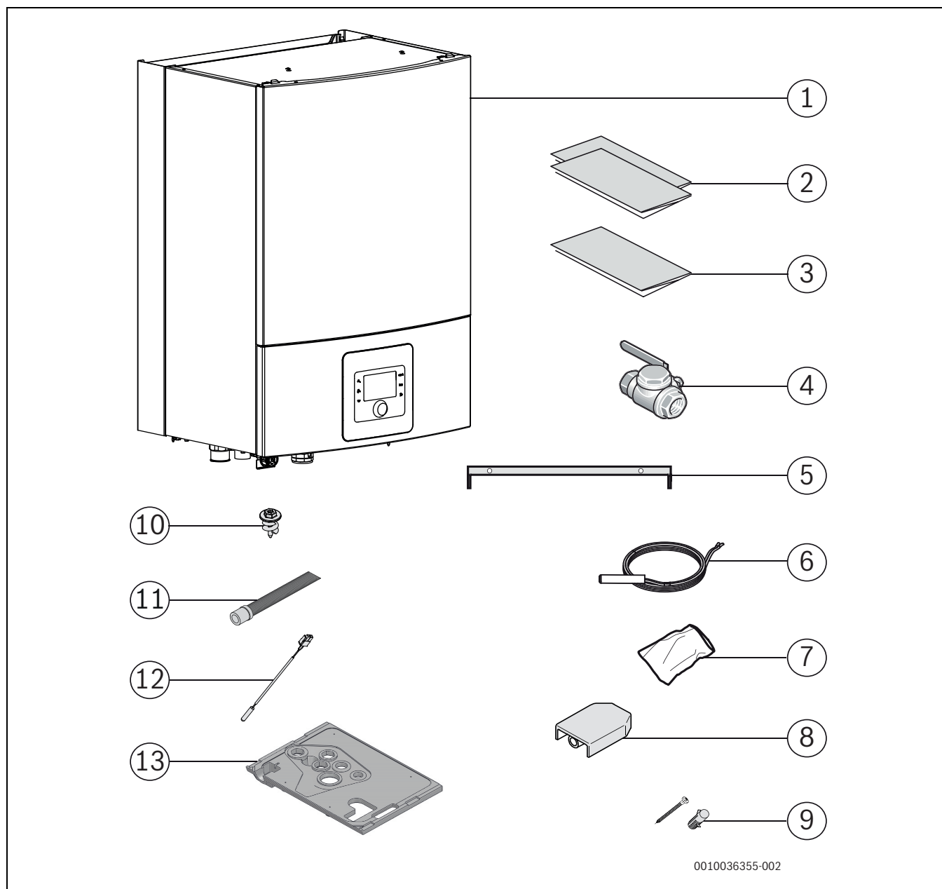
Fig. 2 Pièces fournies
