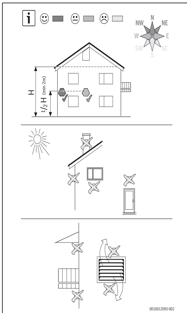
Fig. 13 Positionnement de la sonde de température extérieure
