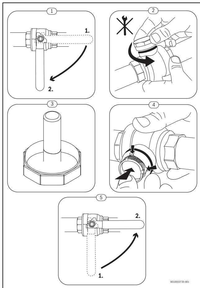
Fig. 19 Nettoyage du filtre
