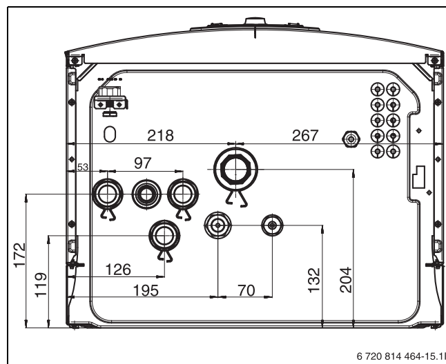
Fig. 5 Dimensions et raccordements (vue sans bac de récupération)
