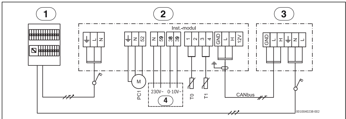
Fig. 42 Schéma de câblage
