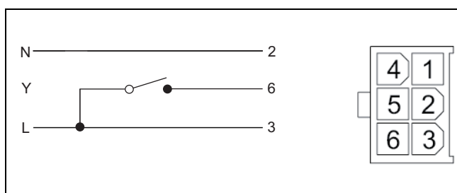
Fig. 23 Connecteur Molex
