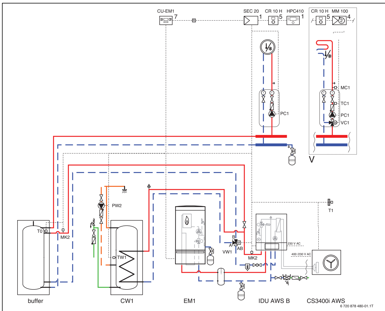
Fig. 39 Unité extérieure avec unité intérieure et deux circuits de chauffage
