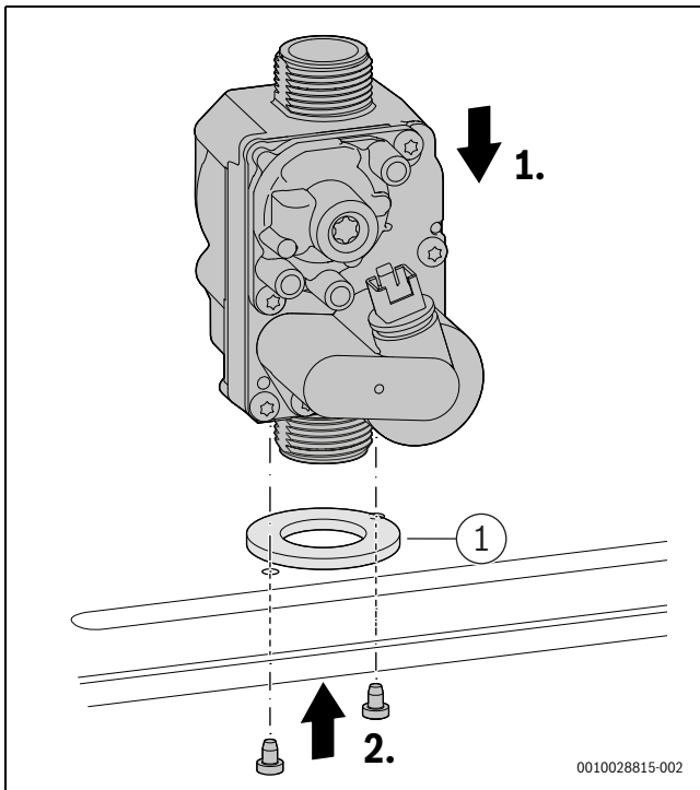
Bild 74 Gasarmatur einbauen
