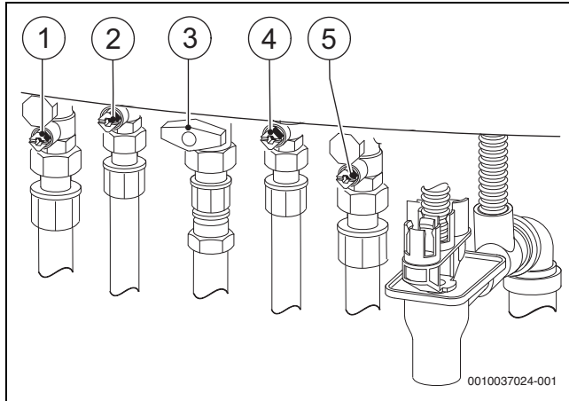
Bild 38 Gas- und wasserseitige Anschlüsse
