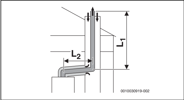
Bild 14 Starre Abgasführung nach C 93x im Schacht und konzentrische Luft-Abgas-Führung im Aufstellraum
