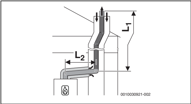
Bild 15 Flexible Abgasführung nach C 93x im Schacht und konzentrische Luft-Abgas-Führung im Aufstellraum
