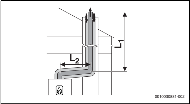
Bild 9 Konzentrische Luft-Abgas-Führung nach C 33x im Schacht
