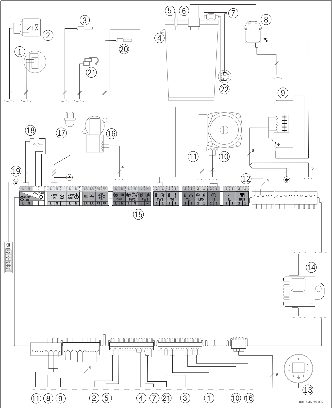
Bild 83 Elektrische Verdrahtung
