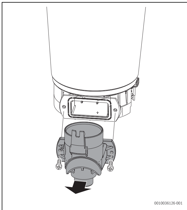
Bild 60 Prüfföffnung öffnen
