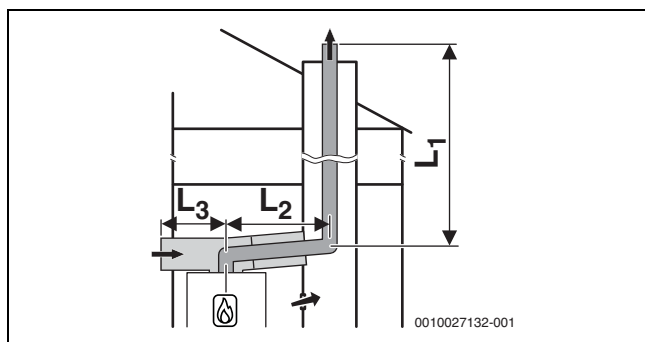
Bild 11 Starre Abgasführung nach C 53x im Schacht und Luft-Abgas-Führung mit separater Luftzufuhr und konzentrischer Abgasableitung im Aufstellraum
