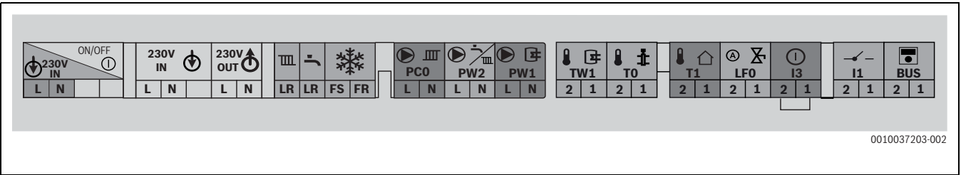
Bild 41 Klemmleiste für externes Zubehör
