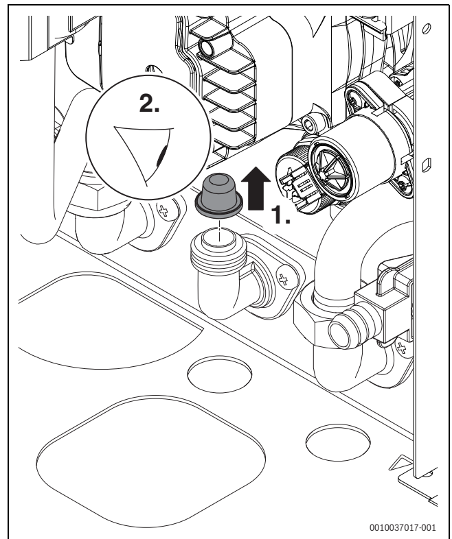
Bild 69 Sieb im Kaltwasserrohr prüfen
