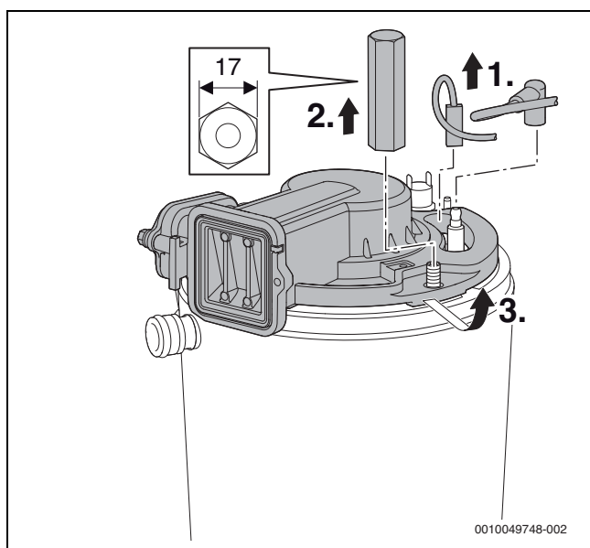
Bild 52 Brennerdeckel lösen
