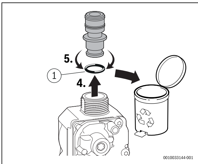
Bild 71 Gasdrossel abnehmen
