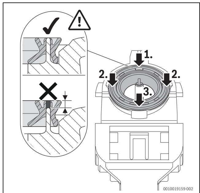
Bild 66 Dichtung andrücken
