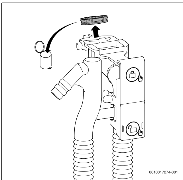
Bild 64 Dichtung oben am Kondensatsiphon entfernen
