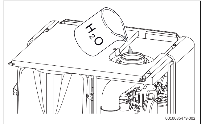
Bild 36 Kondensatsiphon mit Wasser füllen
