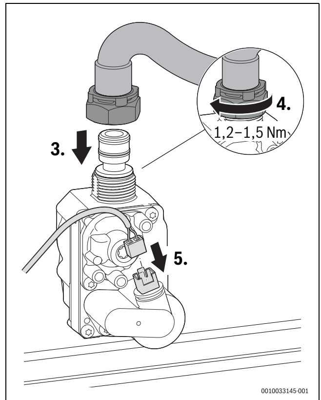
Bild 77 Gasschlauch und Stecker anschließen – Anzugsdrehmoment beachten
