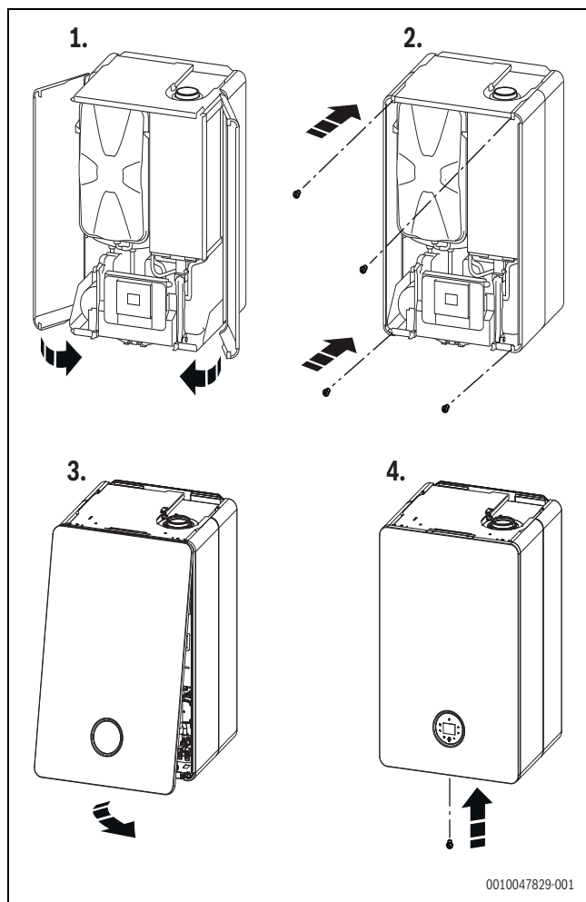
Bild 42 Verkleidung montieren
