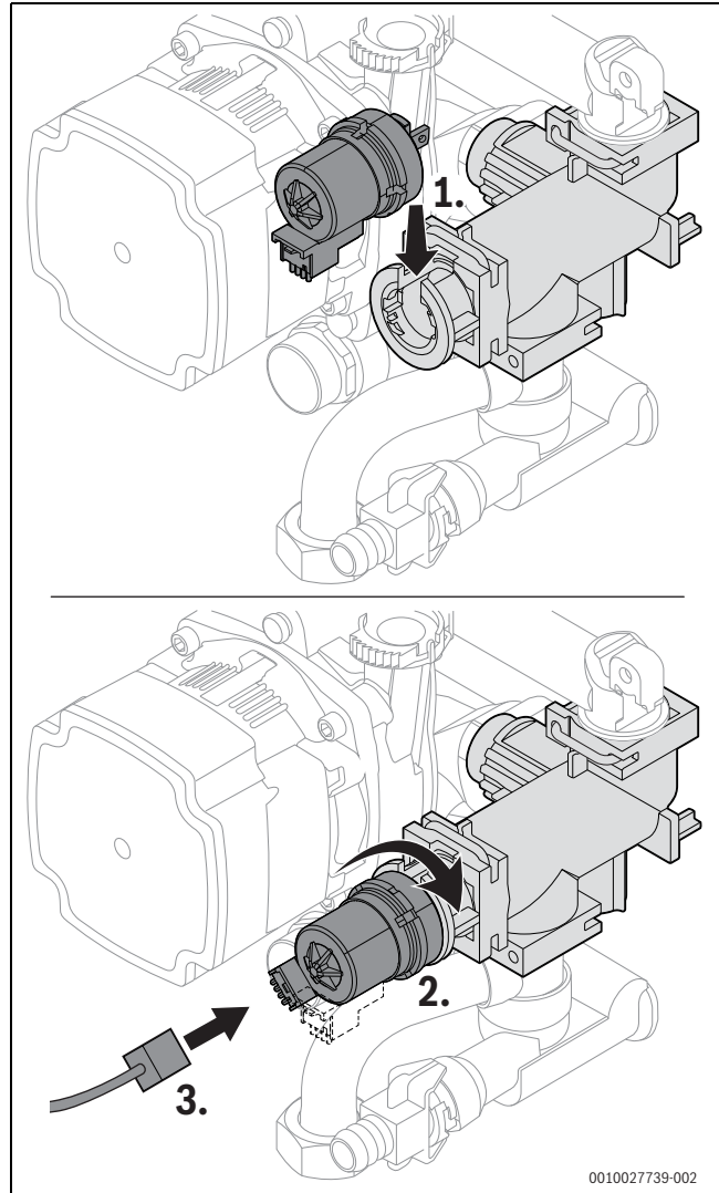
Bild 79 Motor am 3-Wege-Ventil einbauen (Variante ohne Schrauben)
