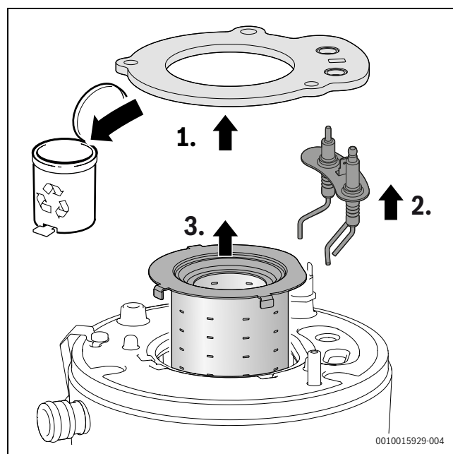
Bild 54 Brenner herausnehmen
