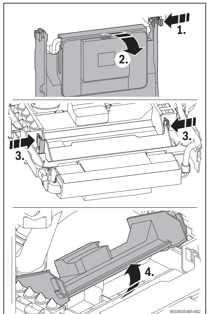
Bild 39 Steuergerät öffnen
