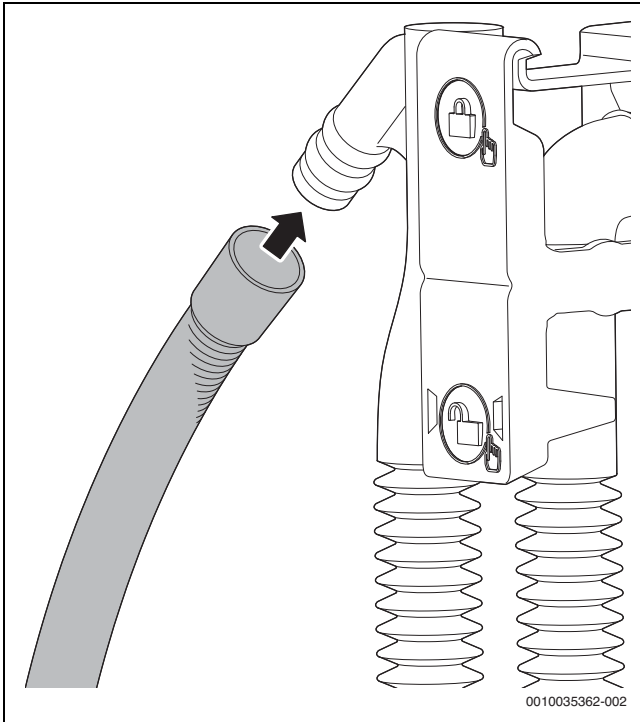
Bild 34 Kondensatschlauch am Kondensatsiphon montieren
