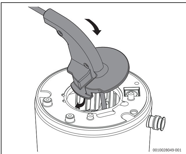
Bild 57 Bürste in den Wärmeblock einsetzen
