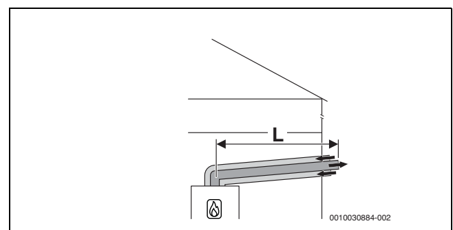
Bild 7 Horizontale konzentrische Luft-Abgas-Führung nach C 13x durch die Außenwand
