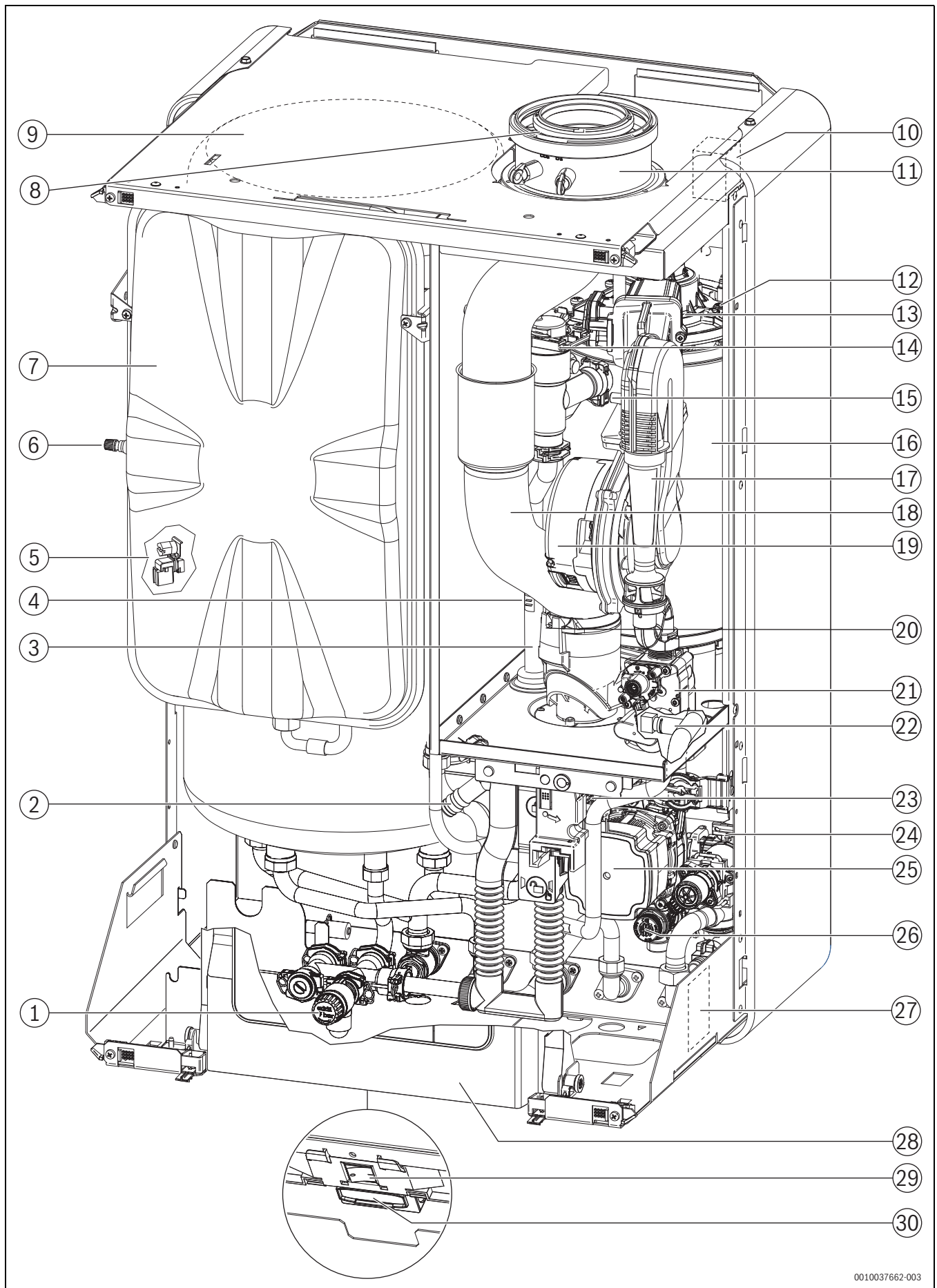
Bild 4 Produktübersicht
