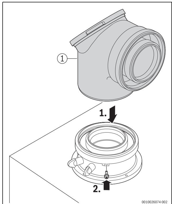
Bild 37 Abgaszubehör einsetzen und mit Schraube sichern
