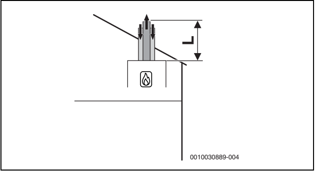
Bild 10 Vertikale konzentrische Luft-Abgas-Führung nach C 33x
