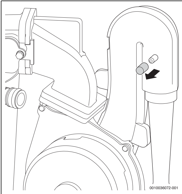
Bild 49 Messstutzen an der Mischeinrichtung
