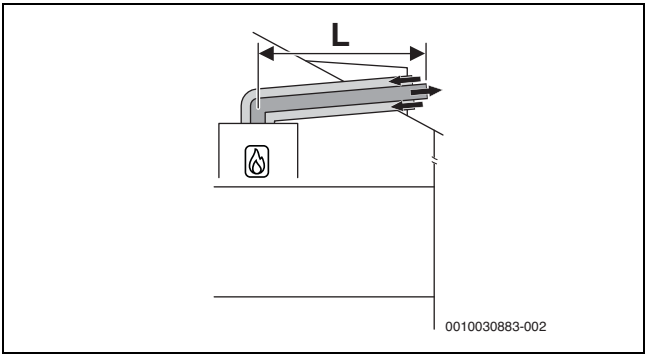
Bild 8 Horizontale konzentrische Luft-Abgas-Führung nach C 13x über das Dach
