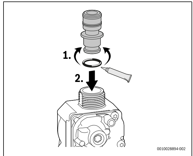
Bild 76 Gasdrossel einsetzen
