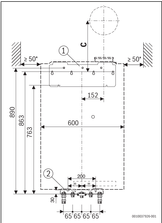
Bild 3 Frontansicht (mm)
