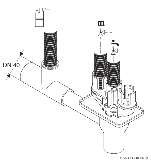
Bild 35 Kondensatschlauch und Schläuche der Sicherheitsventile am Siphon montieren
