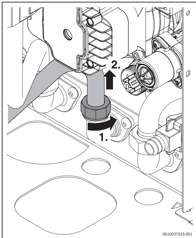
Bild 68 Rohr am Kaltwasseranschluss abnehmen
