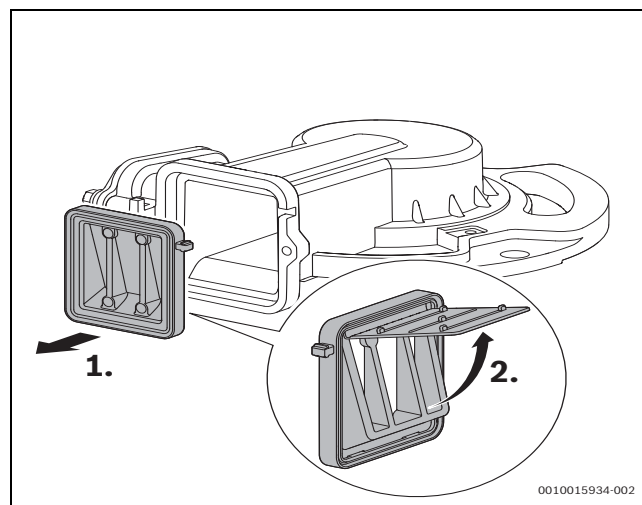
Bild 53 Rückschlagklappe in der Mischeinrichtung
