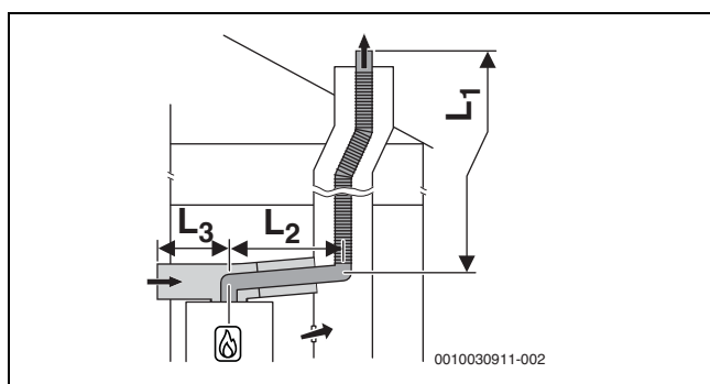
Bild 12 Flexible Abgasführung nach C 53x im Schacht und Luft-Abgas-Führung mit separater Luftzufuhr und konzentrischer Abgasableitung im Aufstellraum
