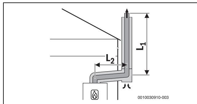
Bild 13 Konzentrische Luft-Abgas-Führung nach C 53x an der Außenwand
