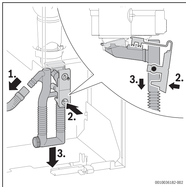
Bild 62 Kondensatsiphon ausbauen
