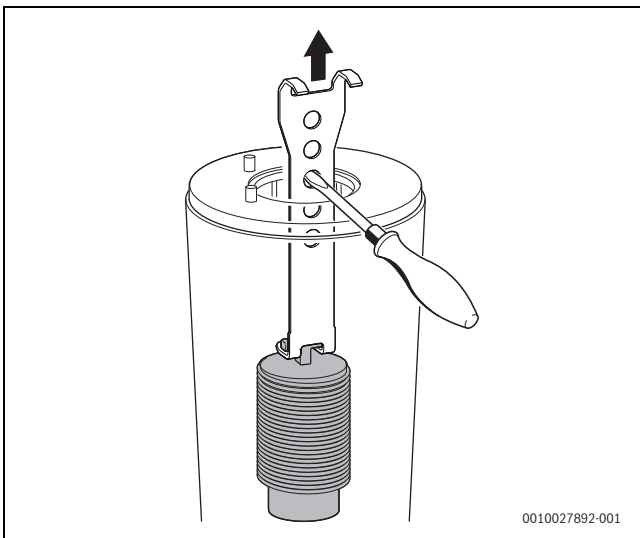
Bild 56 Unteren Verdrängungskörper herausnehmen
