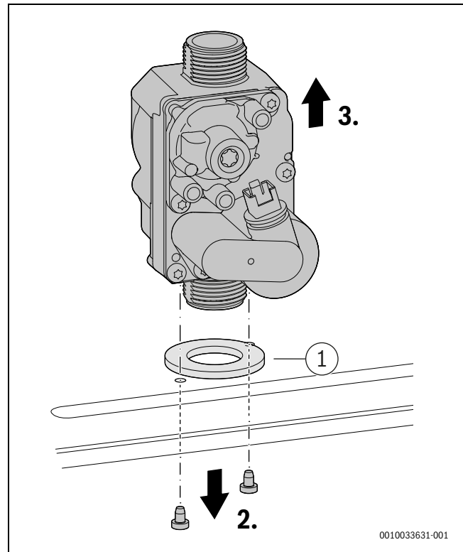
Bild 73 Gasarmatur ausbauen
