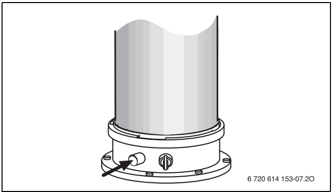
Bild 47 Stopfen abnehmen
