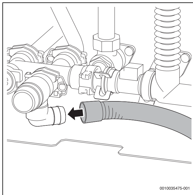
Bild 33 Schlauch am Sicherheitsventil (Warmwasserkreis) montieren
