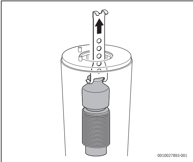
Bild 55 Oberen Verdrängungskörper herausnehmen
