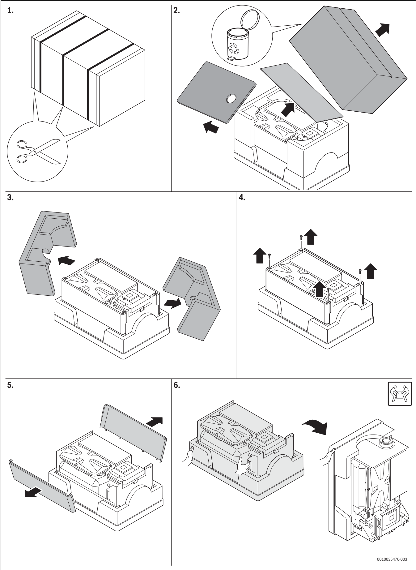
Bild 29 Auspackanweisung
