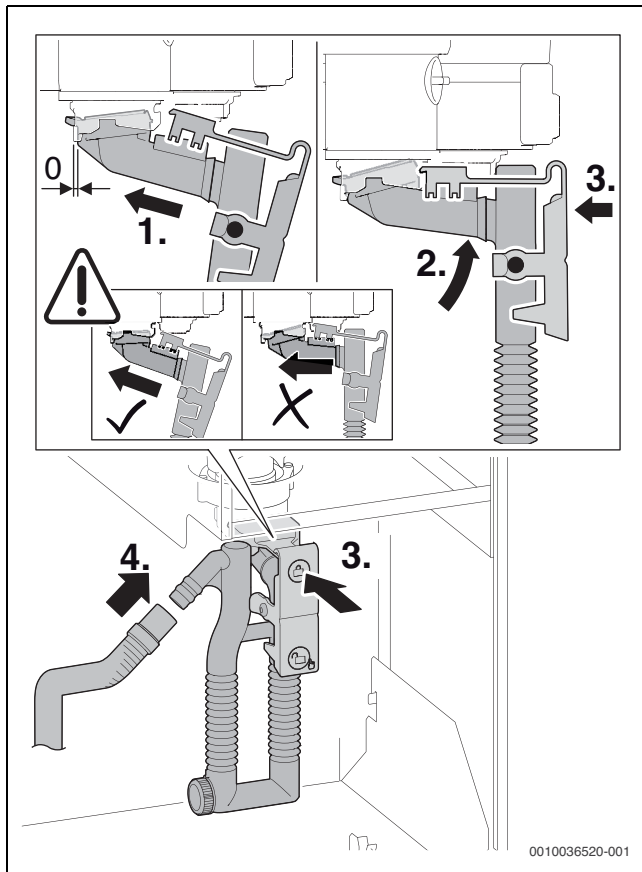
Bild 67 Kondensatsiphon einsetzen
