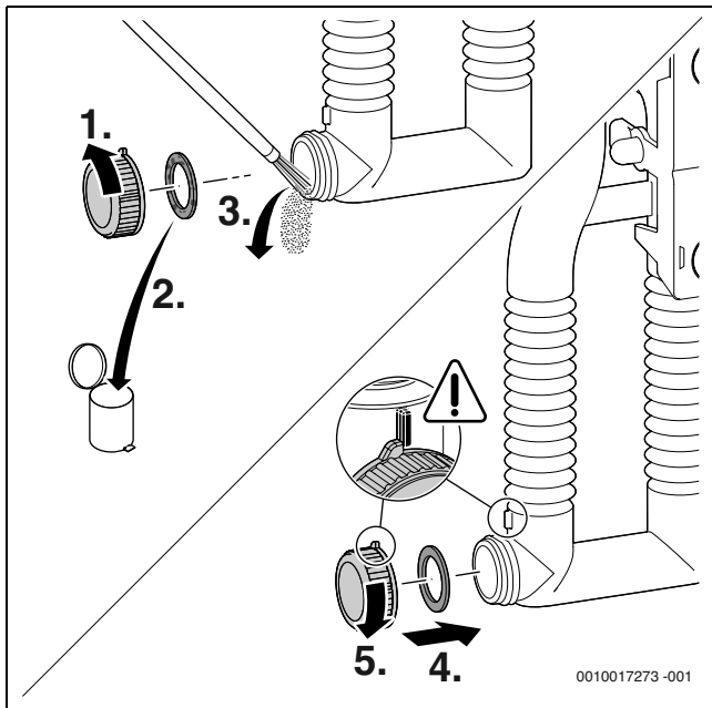
Bild 63 Kondensatsiphon reinigen
