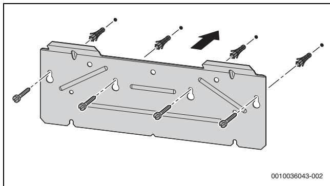
Bild 30 Aufhängeschiene montieren
