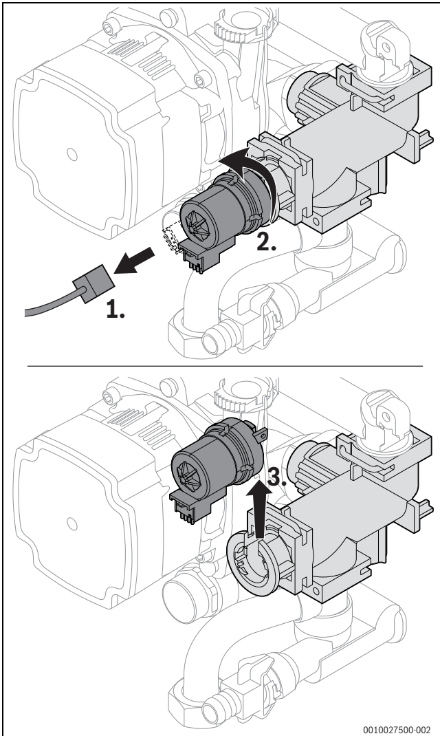
Bild 78 Motor am 3-Wege-Ventil ausbauen (Variante ohne Schrauben)
