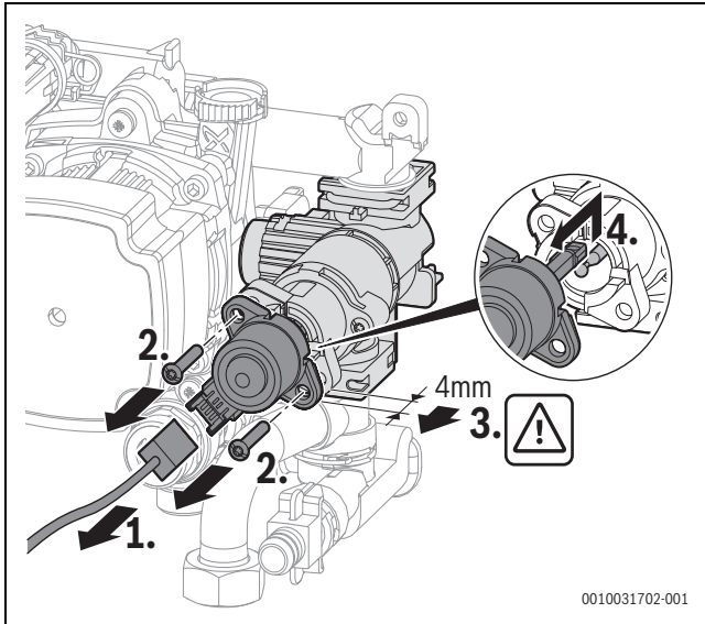
Bild 80 Motor am 3-Wege-Ventil ausbauen (Variante mit Schrauben)
