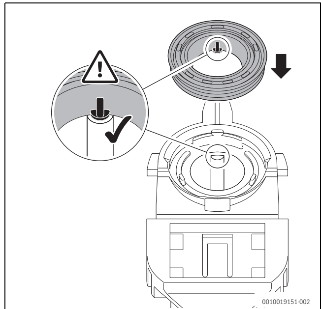
Bild 65 Neue Dichtung am Kondensatsiphon ausrichten
