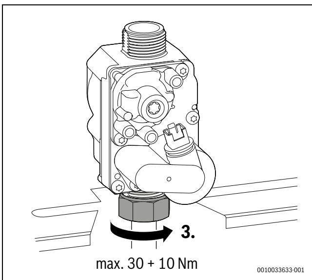
Bild 75 Anzugsdrehmoment beachten
