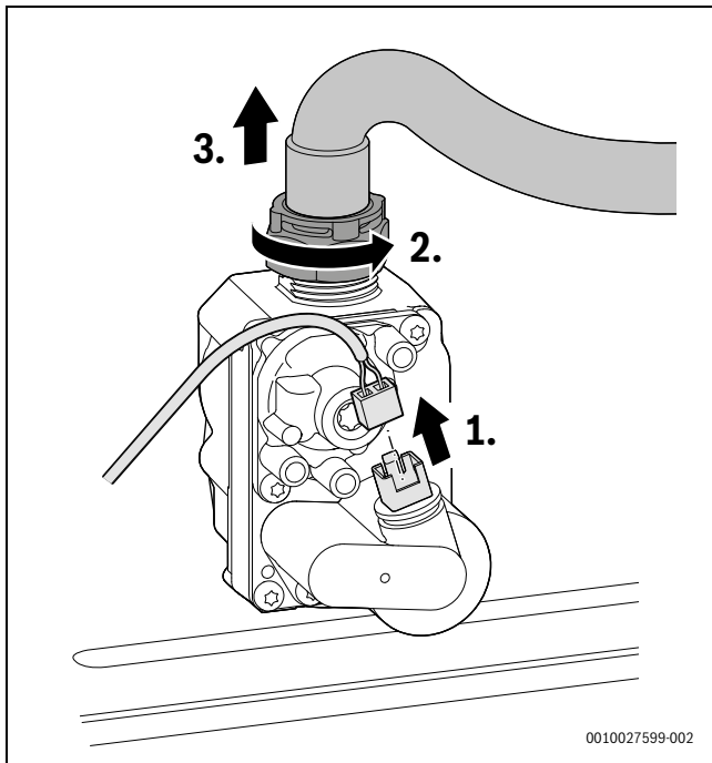
Bild 70 Stecker an der Gasarmatur abziehen und Überwurfmutter mit Gasschlauch abnehmen
