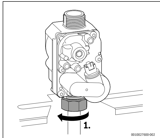
Bild 72 Überwurfmutter lösen
