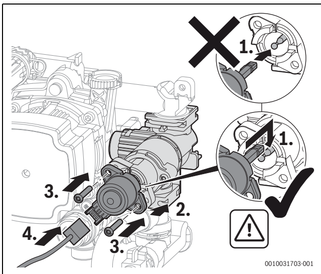
Bild 81 Motor am 3-Wege-Ventil einbauen (Variante mit Schrauben)
