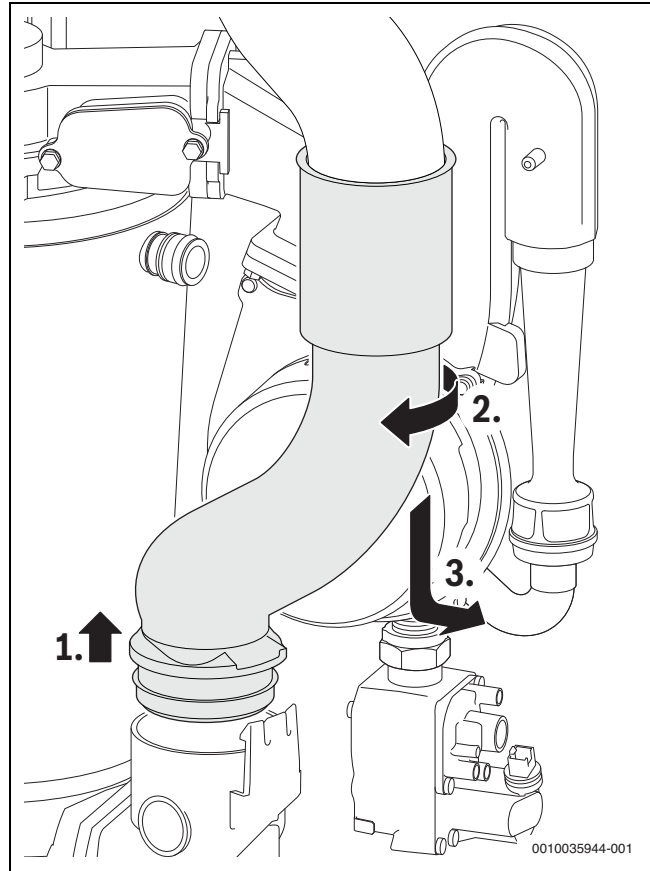
Bild 50 Abgasrohr ausbauen
