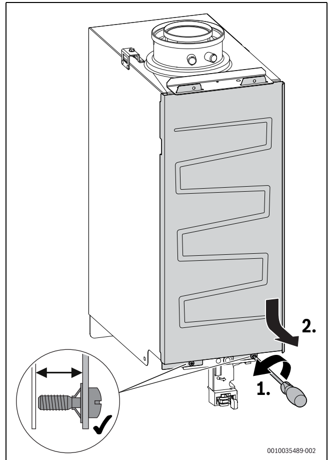
Bild 45 Brennerhaube abnehmen
