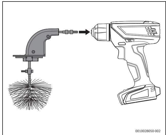
Afb. 58 Borstel met accuschroefmachine verbinden
