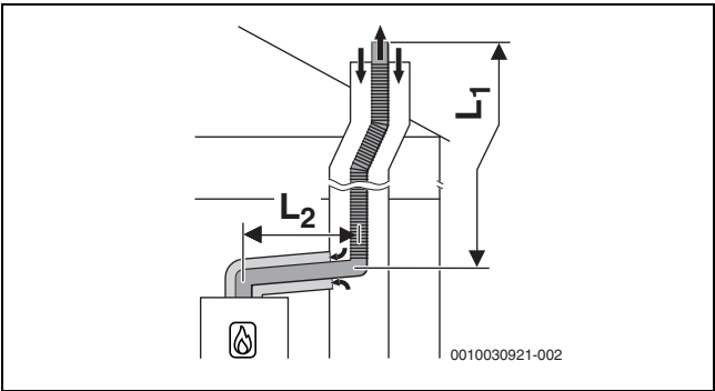
Afb. 15 Flexibel rookgasafvoertraject conform C 93x in de schacht en concentrisch luchttoevoer/rookgasafvoersysteem in de opstellingsruimte
