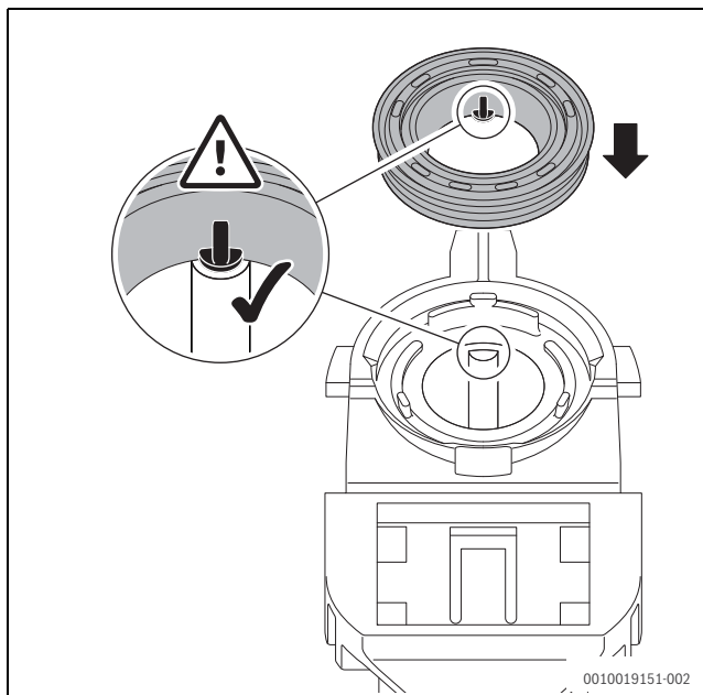
Afb. 65 Dichting correct op de condenssifon plaatsen
