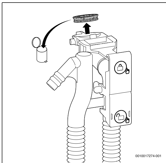
Afb. 64 Verwijder de dichting boven op de condenssifon
