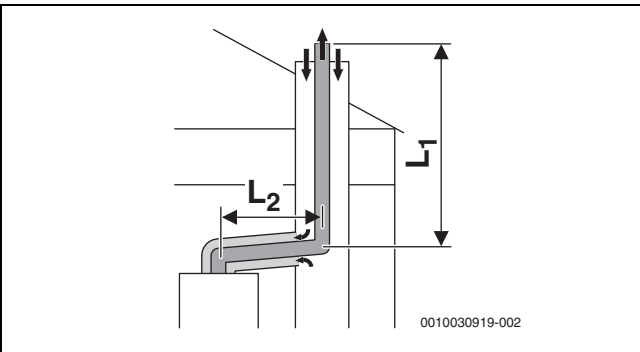
Afb. 14 Star rookgasafvoertraject conform C 93x in de schacht en concentrisch luchttoevoer/rookgasafvoersysteem in de opstellingsruimte
