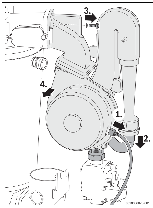
Afb. 51 Ventilator met menginrichting demonteren
