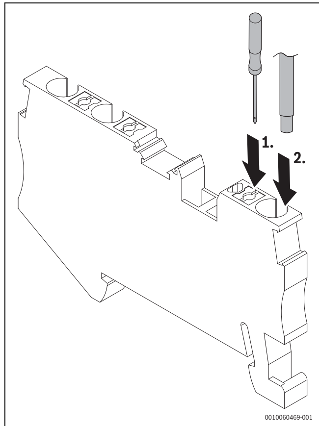
Afb. 35 Netkabelaansluiting
