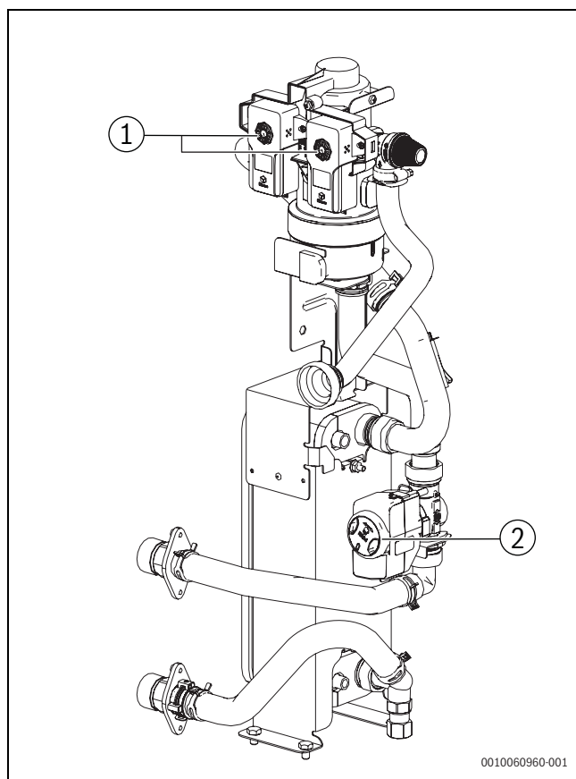
Afb. 42 Propaanveiligheidskit
