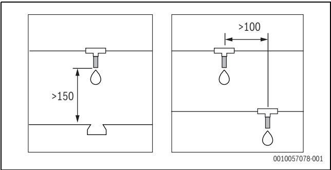
Afb. 23 Benodigde ruimte voor installatie van antivriesventielen in millimeter (mm)
