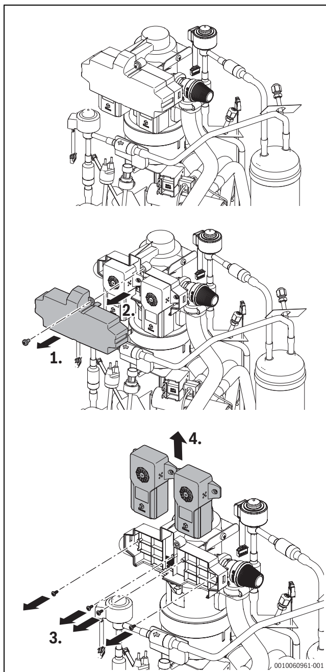
Afb. 43 Vervanging van de R290-sensoren
