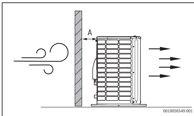
Afb. 19 Vrijstaande warmtepomp
