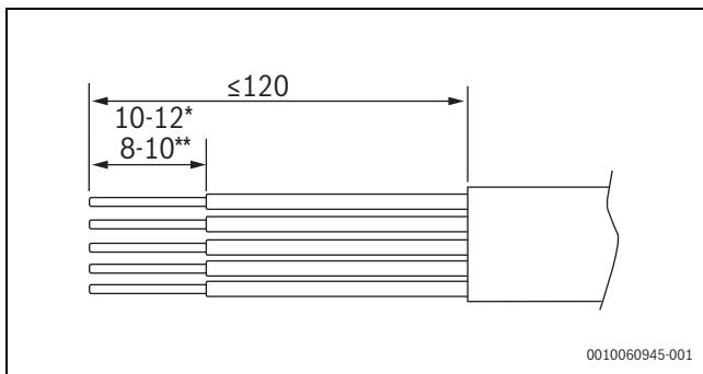
Afb. 34 De draden strippen voor de voedingsaansluiting (mm)
