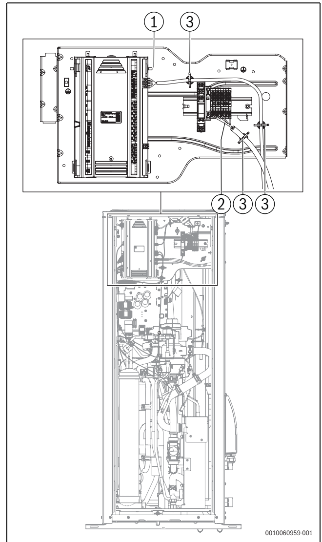
Afb. 37 Aansluitklemmen op de aansluitlocatie van de installatie (O-T)
