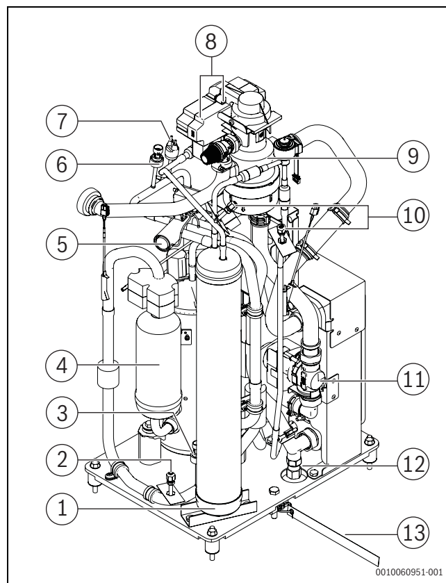
Afb. 2 Overzicht koelmiddelcircuit
