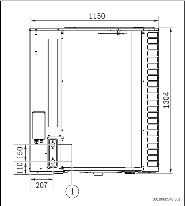
Afb. 4 Afmetingen warmtepomp en hydraulische koppelingen, achter-aanzicht
