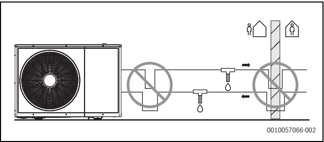
Afb. 22 Installatie antivriesventiel
