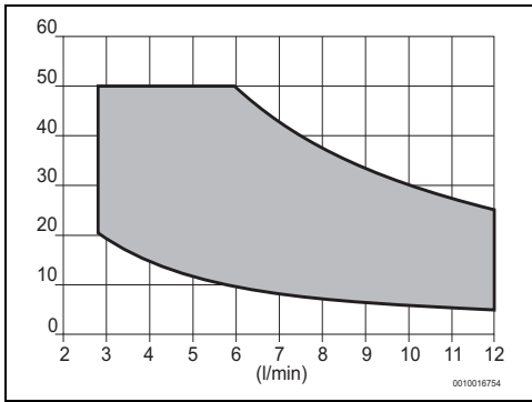
Fig. 29 Modèle 12 litres
