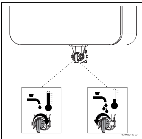
Fig. 9 Contrôle du débit
