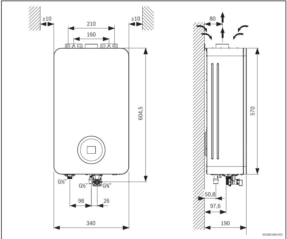
Bild 1 Abmessungen (Maße in mm)
