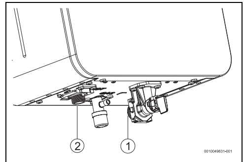
Bild 20 Wasseranschluss
