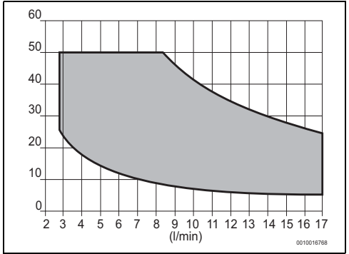
Bild 31 Modell 17 Liter
