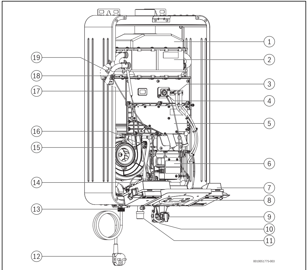
Bild 3 Gerätedesign
