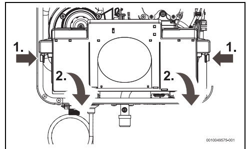
Bild 24 Kippen der Bedieneinheit
