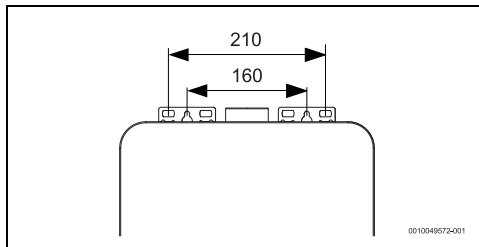
Bild 19 Befestigungspunkte
