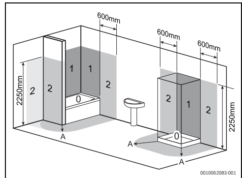
Bild 8 Empfohlene Mindestabstände (mm)
