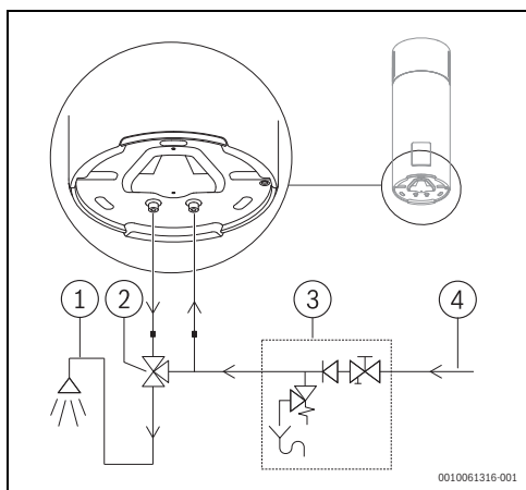
Afb. 20 Watertoevoeraansluitingen
