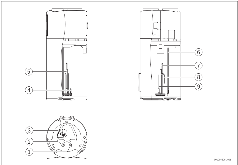
Bild 5 Produktübersicht
