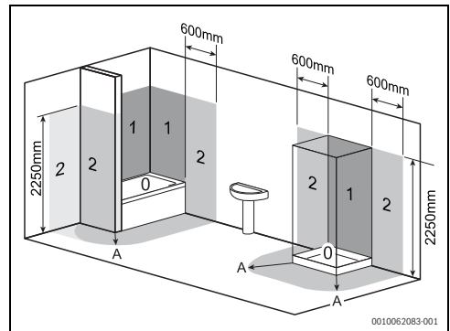
Fig. 8 Dégagements minimaux recommandés (mm)
