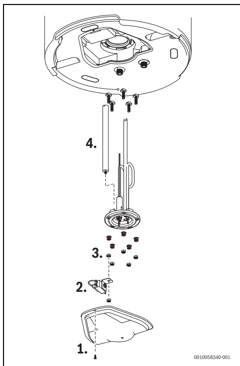
Afb. 31 Verwijderen van de magnesiumanode
