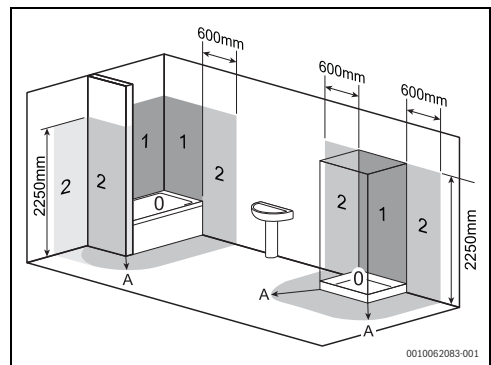
Afb. 8 Aanbevolen minimale vrije ruimten (mm)
