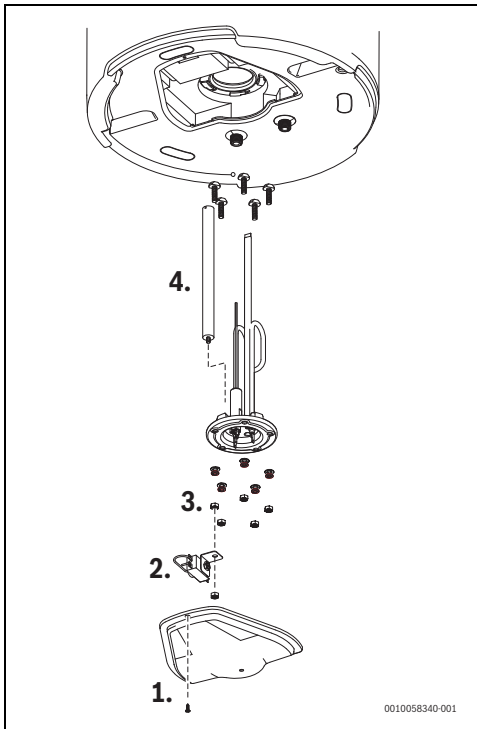
Fig. 31 Retrait de l'anode en magnésium
