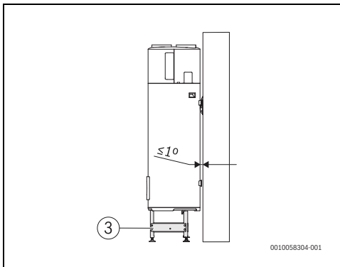
Bild 13 Installieren Sie das Gerät vertikal
