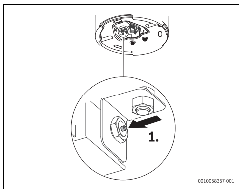
Afb. 32 Resetten van de maximaalthermostaat
