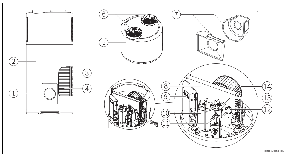
Afb. 4 Productoverzicht
