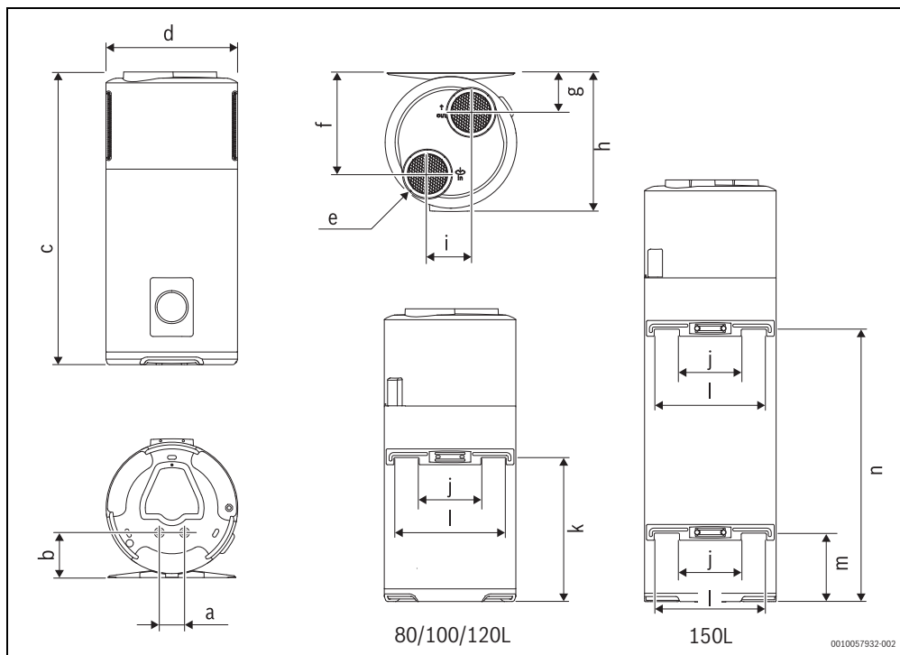
Afb. 3 Toestelafmetingen
