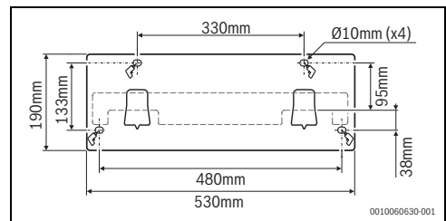
Afb. 11 Bevestigingsstrip
