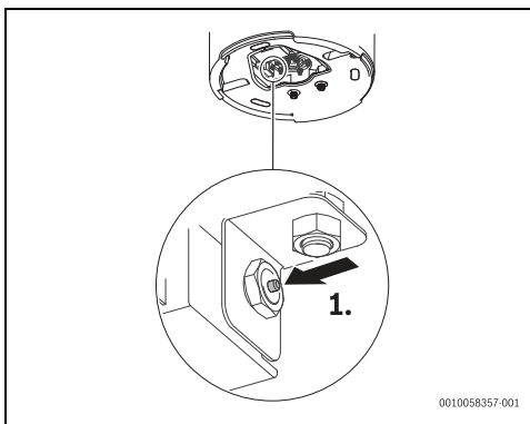
Bild 32 Sicherheitsthermostat zurücksetzen
