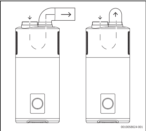
Afb. 16 Speciaal luchtkanaal
