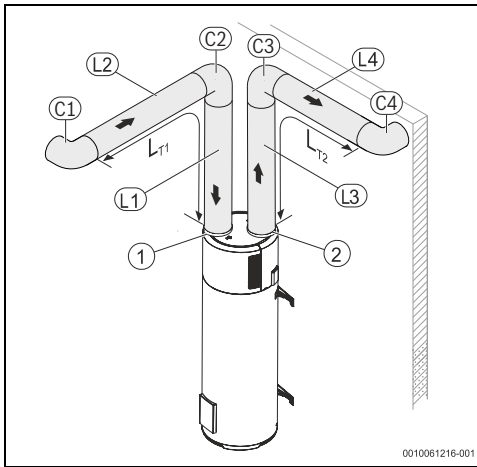
Bild 18 Installationsbeispiel
