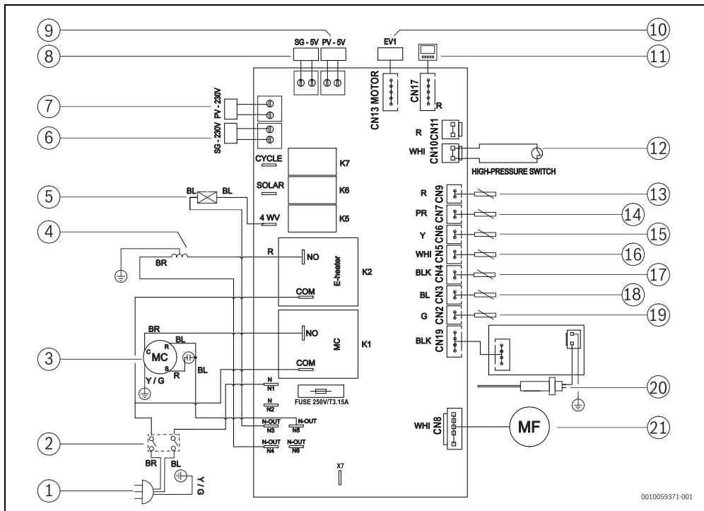
Fig. 33 Schéma électrique
