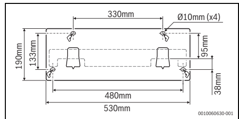
Bild 11 Aufhängeschiene
