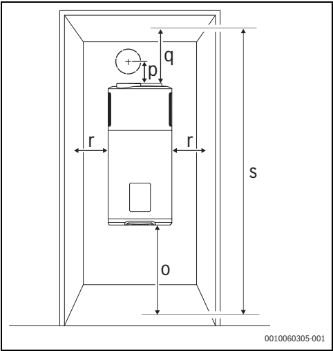
Afb. 9 Minimale afstanden zonder sokkel
