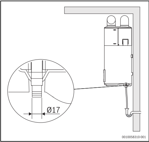
Afb. 21 Aansluiting van de condensatafvoer
