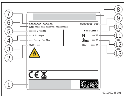
Afb. 2 Beschrijving van de typeplaat
