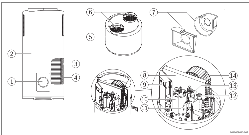
Bild 4 Produktübersicht
