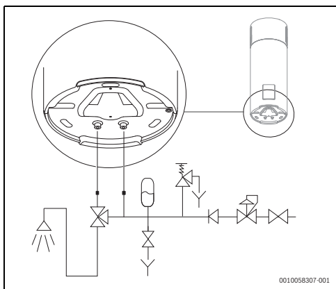
Afb. 20 Watertoevoeraansluitingen
