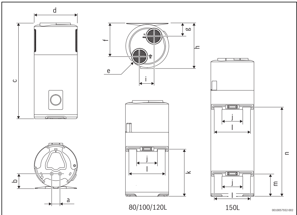
Bild 3 Geräteabmessungen
