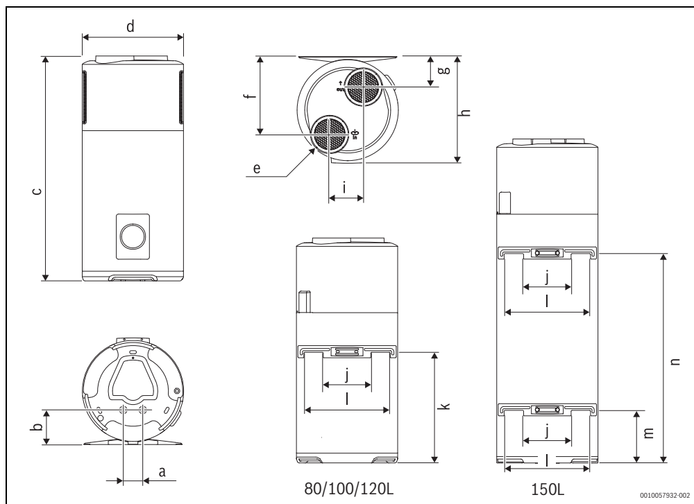
Afb. 3 Afmetingen toestel
