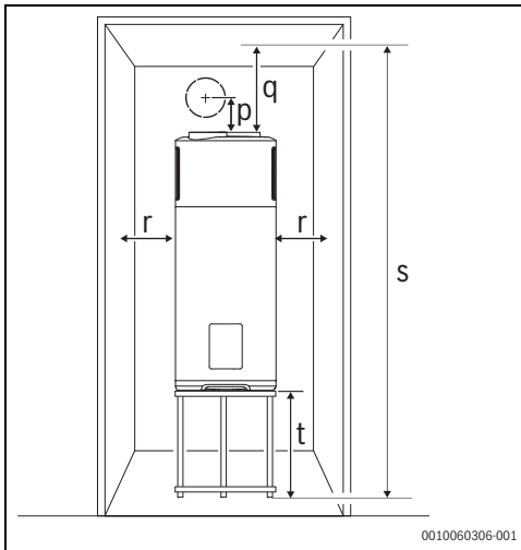
Bild 10 Mindestabstände mit Gestell
