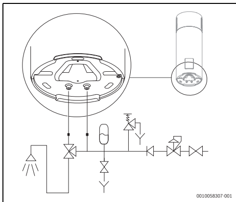
Bild 20 Anschlüsse Wasserzufuhr
