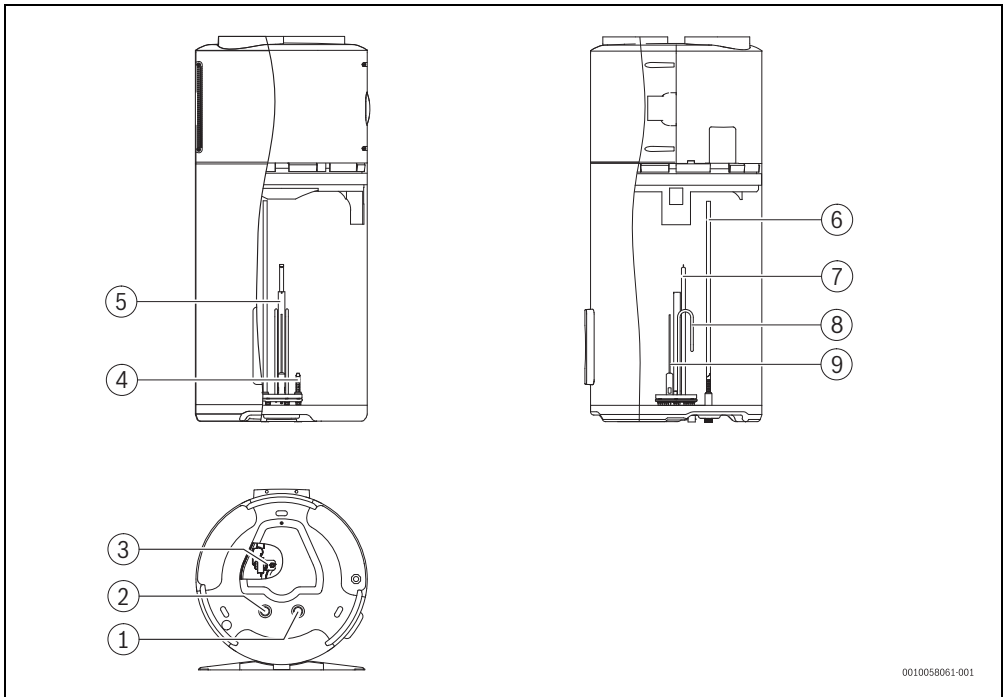
Afb. 5 Productoverzicht
