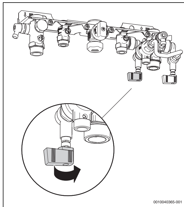
Bild 6 Füllleinrichtung öffnen
