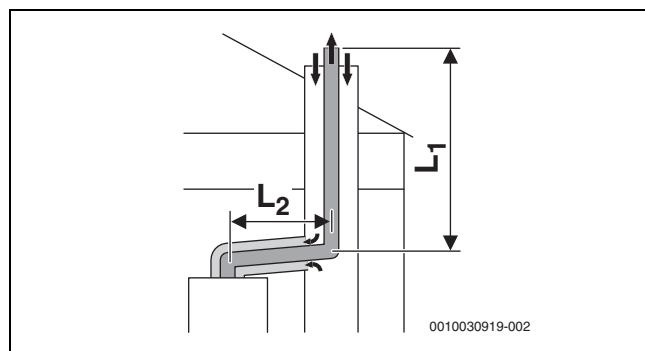
Fig. 17 Évacuation des fumées rigide selon C 93x dans le conduit et circuit d'air et de fumées concentrique dans le local d'installation
