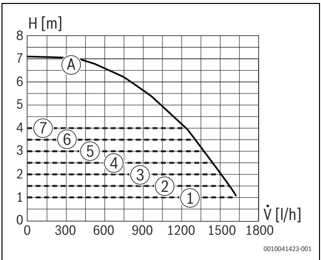
Fig. 70 Diagrammes de pompe et courbes caractéristiques de pompe
