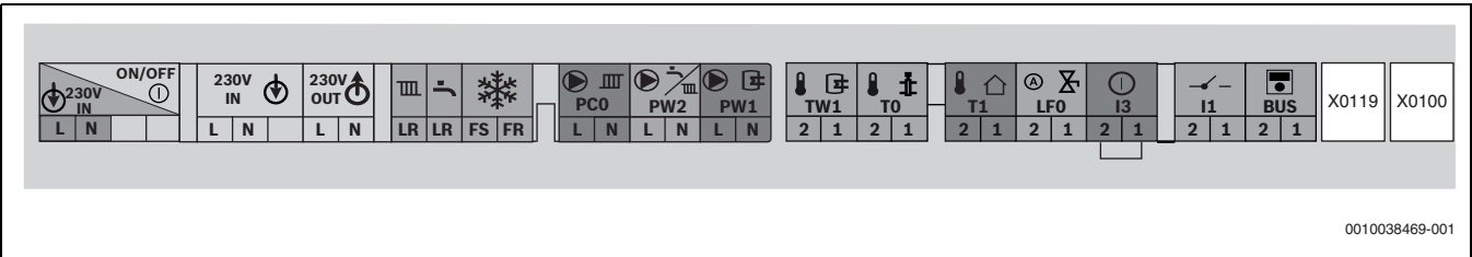
Fig. 38 Bornier pour accessoires externes
