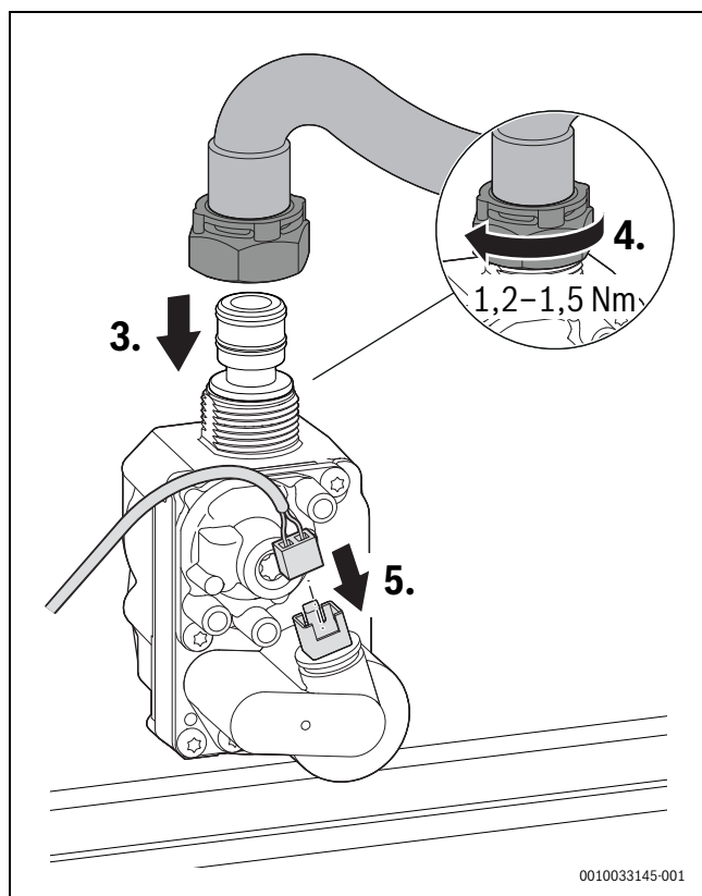
Fig. 59 Raccordement du tuyau du gaz et du connecteur – Respect du couple de serrage
