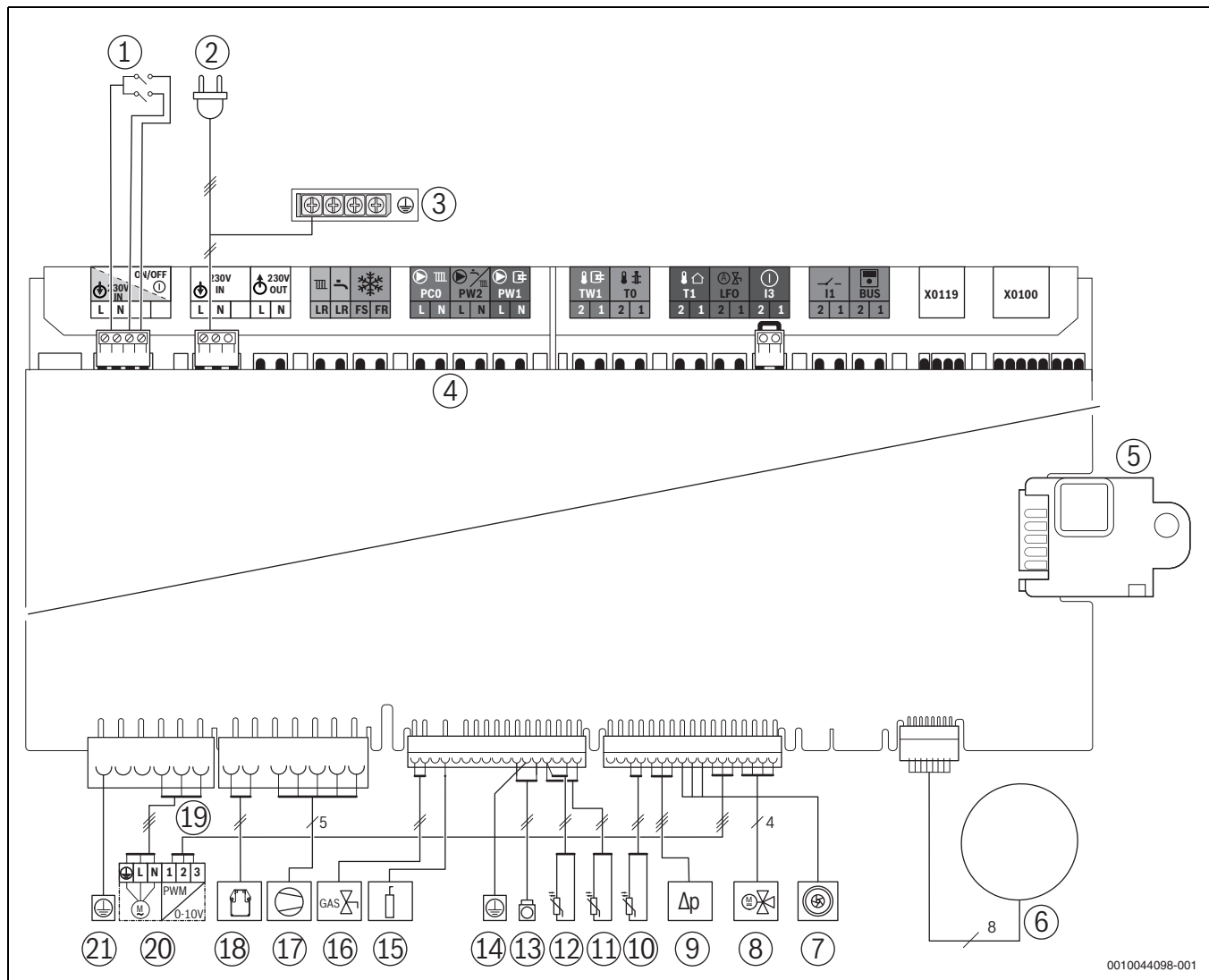
Fig. 71 Câblage électrique
