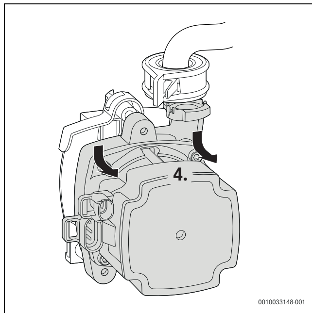
Fig. 50 Retirer la pompe de chaudière par l'avant
