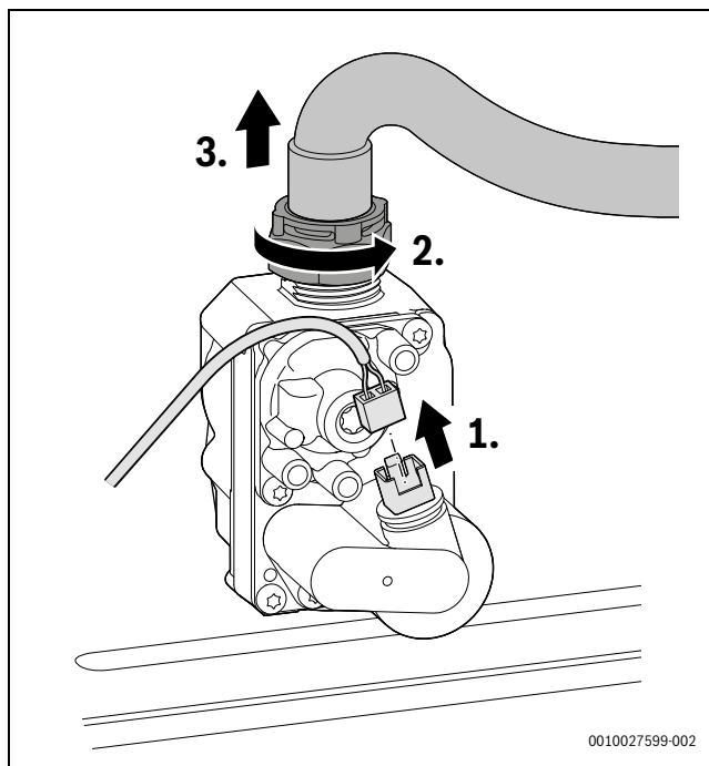
Fig. 52 Retrait du connecteur du bloc gaz et de l'écrou avec le tuyau du gaz
