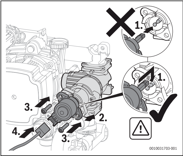
Fig. 69 Remontez le moteur au niveau de la vanne sélective (variante avec vis)
