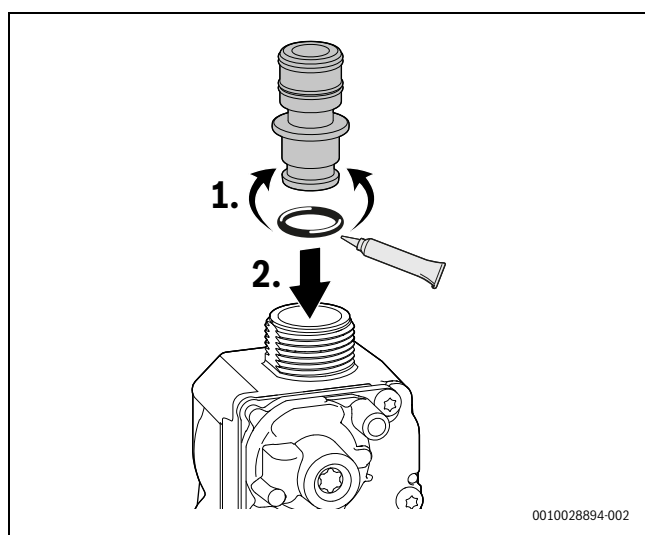
Fig. 58 Insertion l'orifice de réglage de gaz
