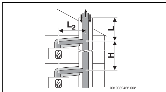
Fig. 24 Raccordement de plusieurs foyers selon C (14)3x avec évacuation des fumées rigide collective et circuit d'air et de fumées concentrique dans le local d'installation
