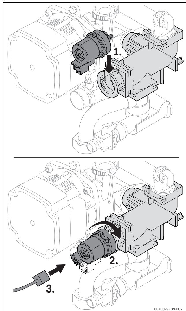
Fig. 67 Remonter le moteur au niveau de la vanne sélective (variante sans vis)
