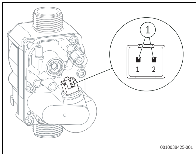
Fig. 47 Points de mesure du bloc gaz
