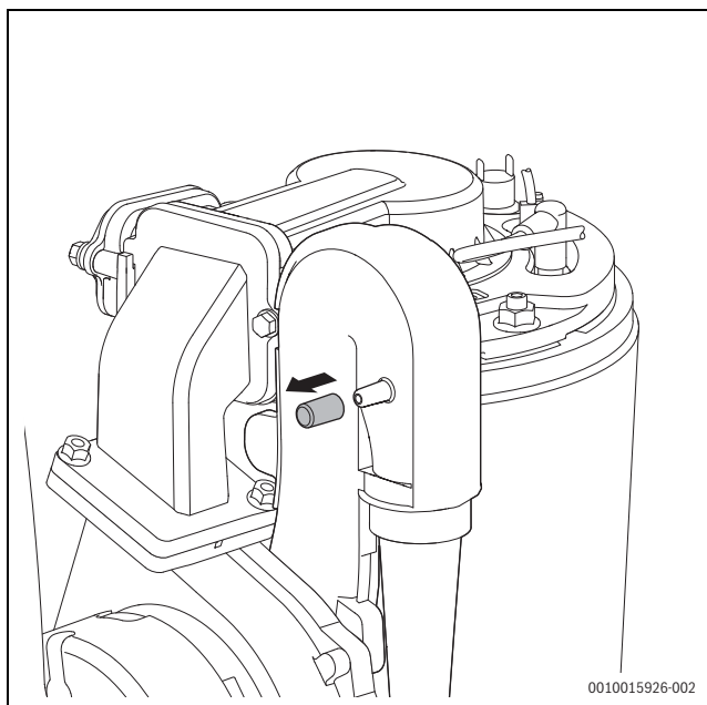
Fig. 46 Tubulure de mesure sur le dispositif de mélange
