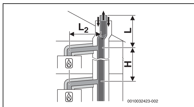
Fig. 25 Raccordement de plusieurs foyers selon C (14)3x avec évacuation des fumées flexible collective et circuit d'air et de fumées concentrique dans le local d'installation
