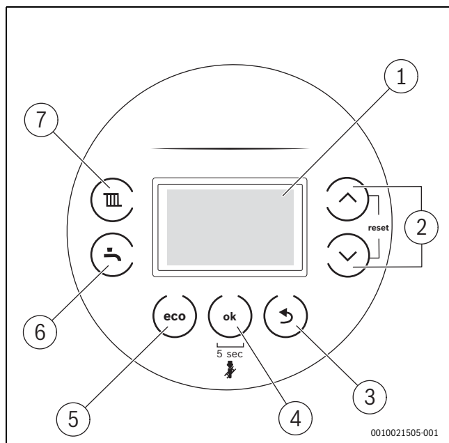
Fig. 40 Tableau de commande
