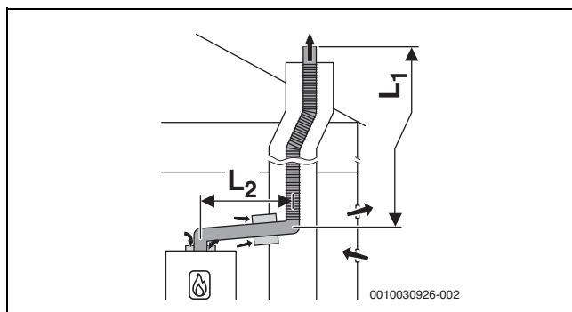
Fig. 20 Evacuation des fumées flexible dans le conduit selon B 53p avec alimentation d'air dépendant de l'air ambiant sur l'appareil et pièce de raccordement concentrique entre le local d'installation et le conduit
