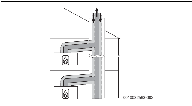
Fig. 21 Raccordement de plusieurs foyers selon C_{(10)3x} avec circuit d'air et de fumées concentrique dans le local d'installation
