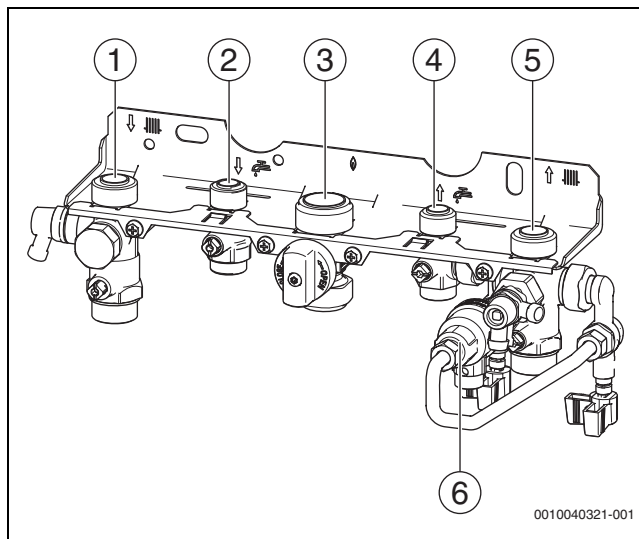
Fig. 34 Raccordements côté gaz et eau
