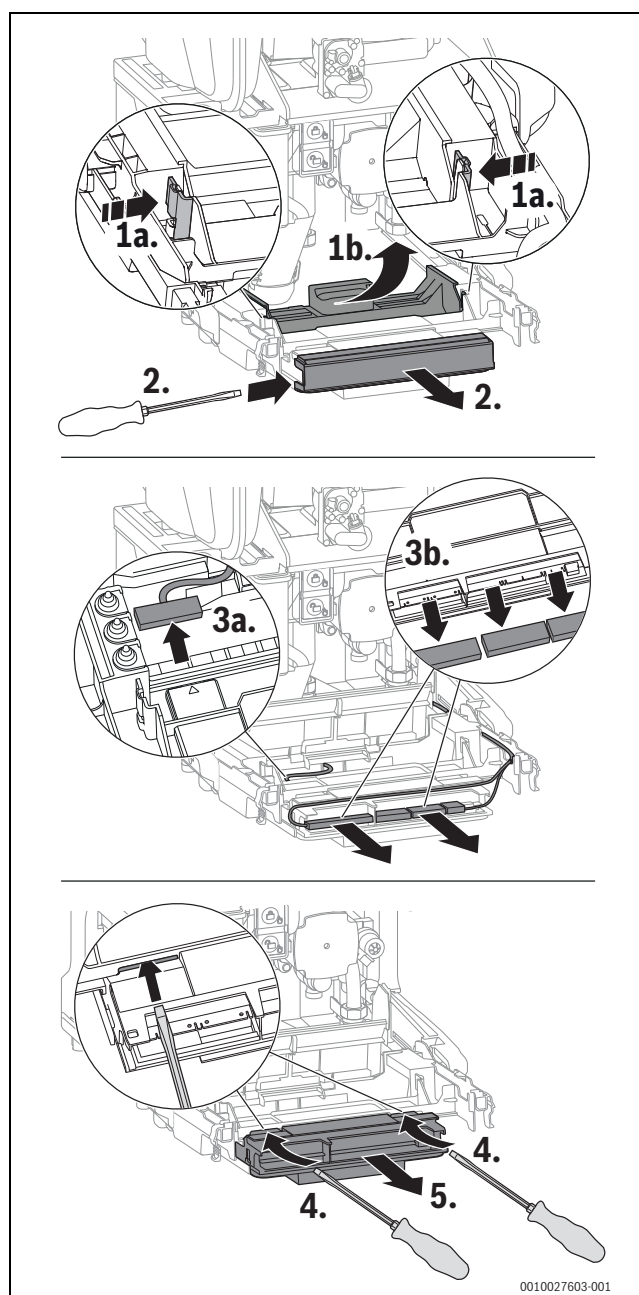
Fig. 60 Retirer l'appareil de commande
