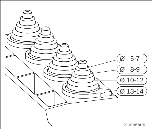
Fig. 37 Adaptation du serre-câbles au diamètre du câble
