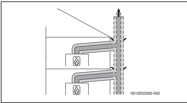
Fig. 22 Raccordement de plusieurs foyers selon C_{(12)3x} avec circuit d'air et de fumées concentrique dans le local d'installation
