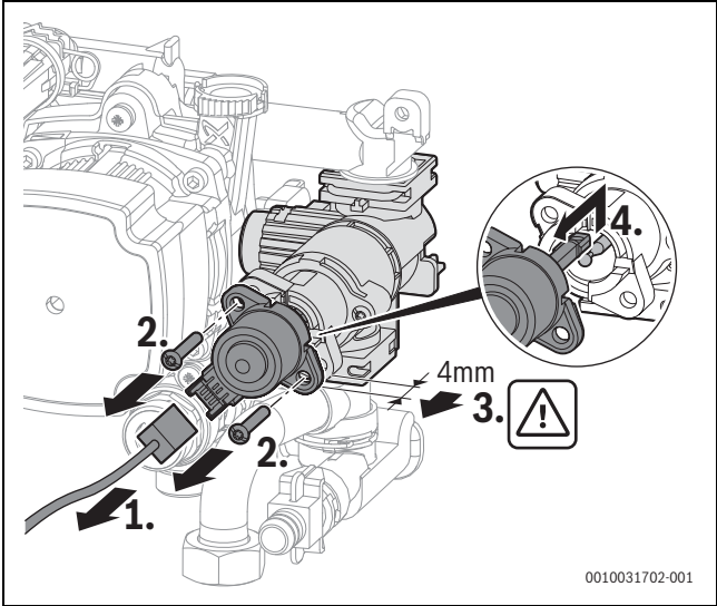
Fig. 68 Démontez le moteur au niveau de la vanne sélective (variante avec vis)
