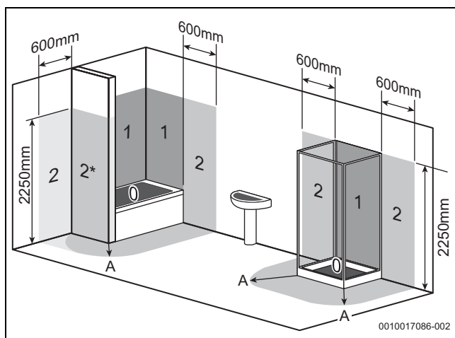
Fig. 27 Volumes de protection (exemple)
