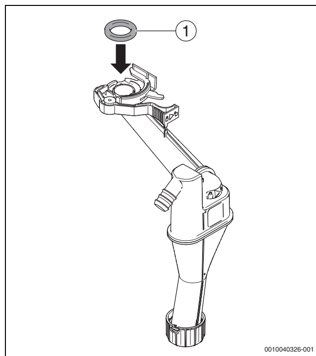
Fig. 63 Mise en place du nouveau joint sur le siphon de condensats
