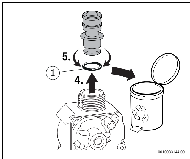
Fig. 53 Retrait de l'orifice
