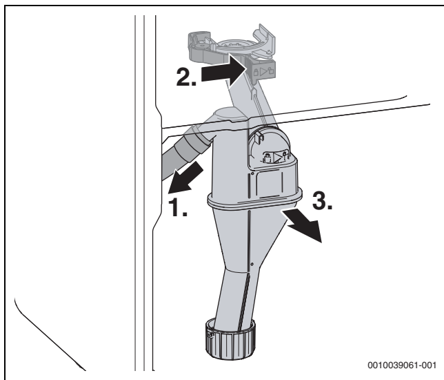
Fig. 61 Démontez le siphon des condensats
