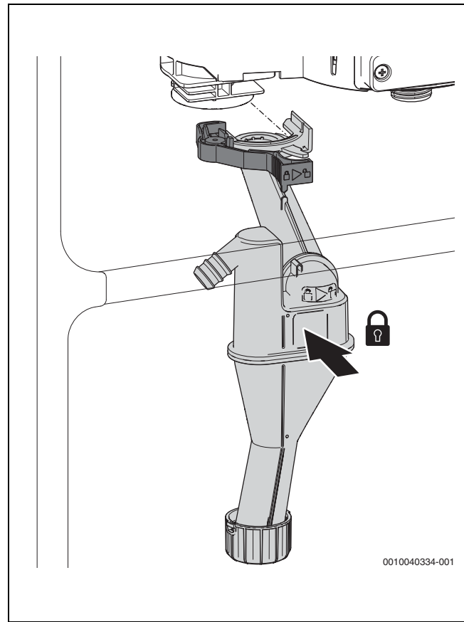
Fig. 65 Insertion du siphon de condensats
