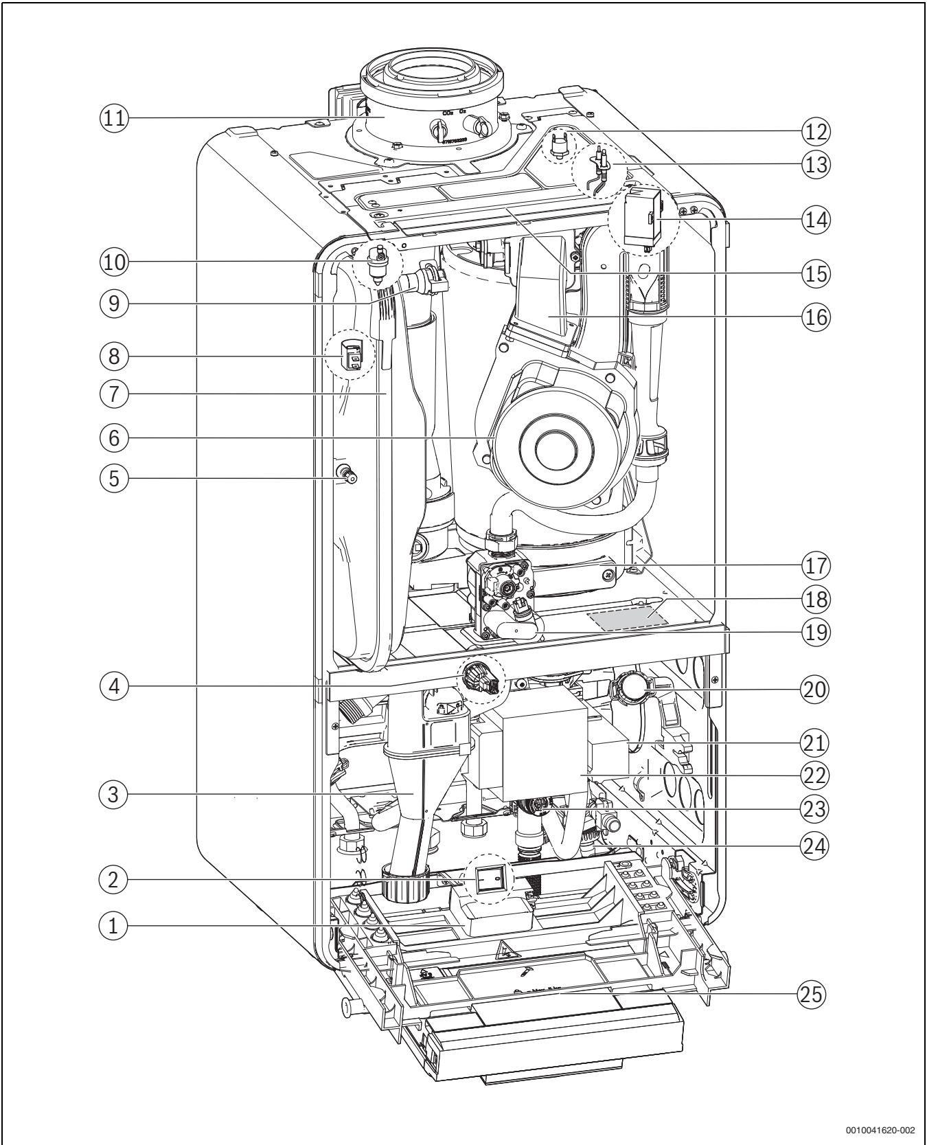
Fig. 7 Aperçu du produit
