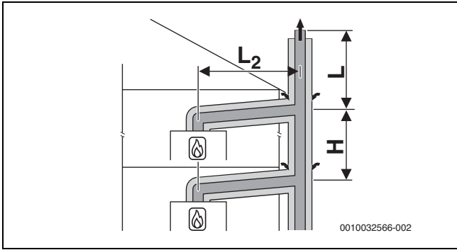
Fig. 23 Raccordement de plusieurs foyers selon C_{(13)3x} avec circuit d'air et de fumées concentrique sur le mur extérieur et dans le local d'installation
