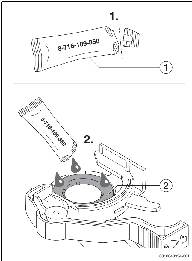
Fig. 64 Graisser le joint
