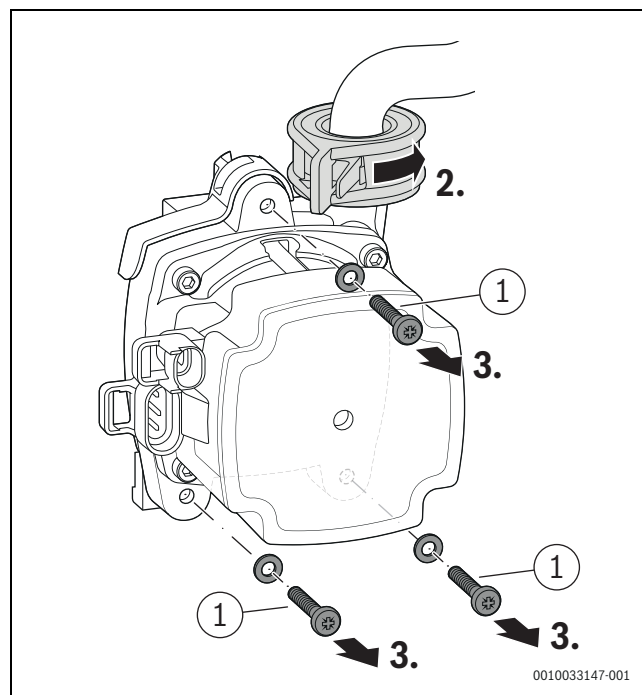
Fig. 49 Déverrouiller la pompe de chaudière et retirer les vis
