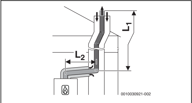
Fig. 18 Évacuation des fumées flexible selon C93x dans le conduit et circuit d'air et de fumées concentrique dans le local d'installation
