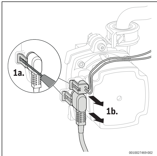
Fig. 48 Débrancher le connecteur de la pompe de chaudière
