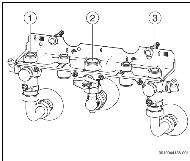
Fig. 35 Raccordements côté gaz et eau
