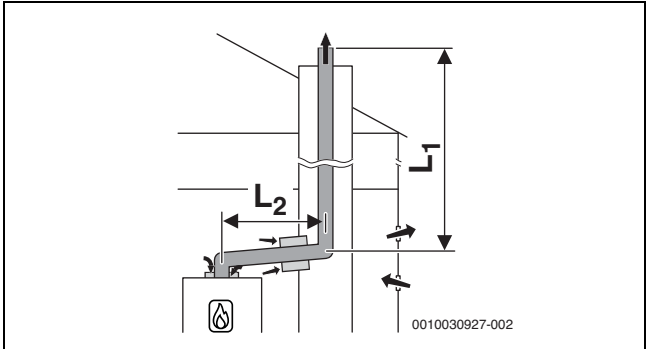
Fig. 19 Évacuation des fumées rigide dans le conduit selon B53p avec alimentation d'air dépendant de l'air ambiant sur l'appareil et pièce de raccordement concentrique entre le local d'installation et le conduit
