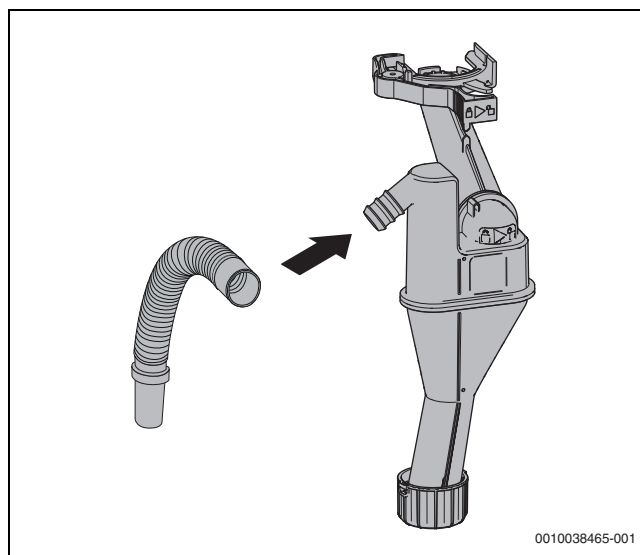
Fig. 31 Placer l'évacuation des condensats sur le raccord
