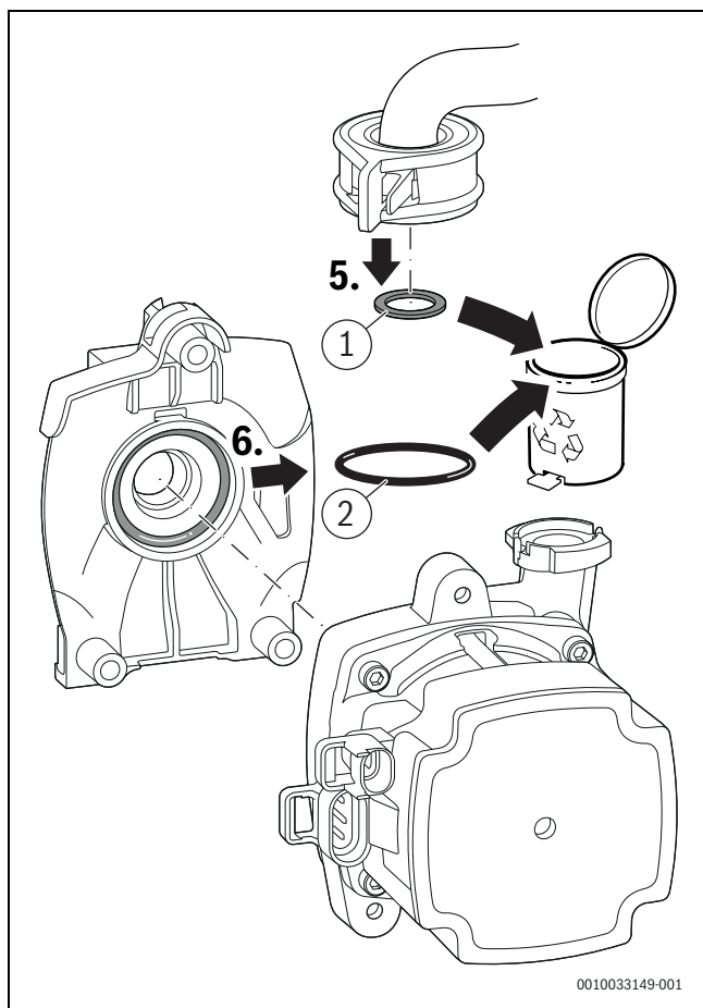
Fig. 51 Éliminer les joints
