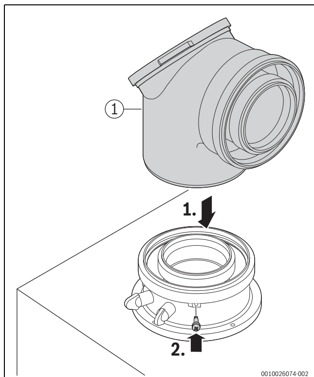
Fig. 33 Insérer les accessoires de fumisterie et fixer avec une vis.
