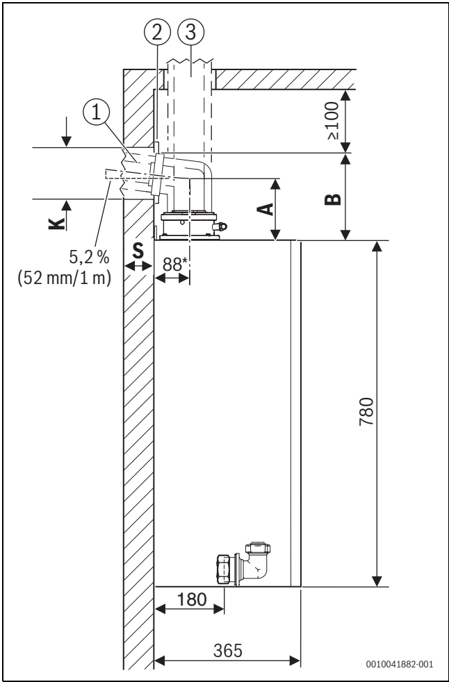
Fig. 4 Vue latérale (mm)
