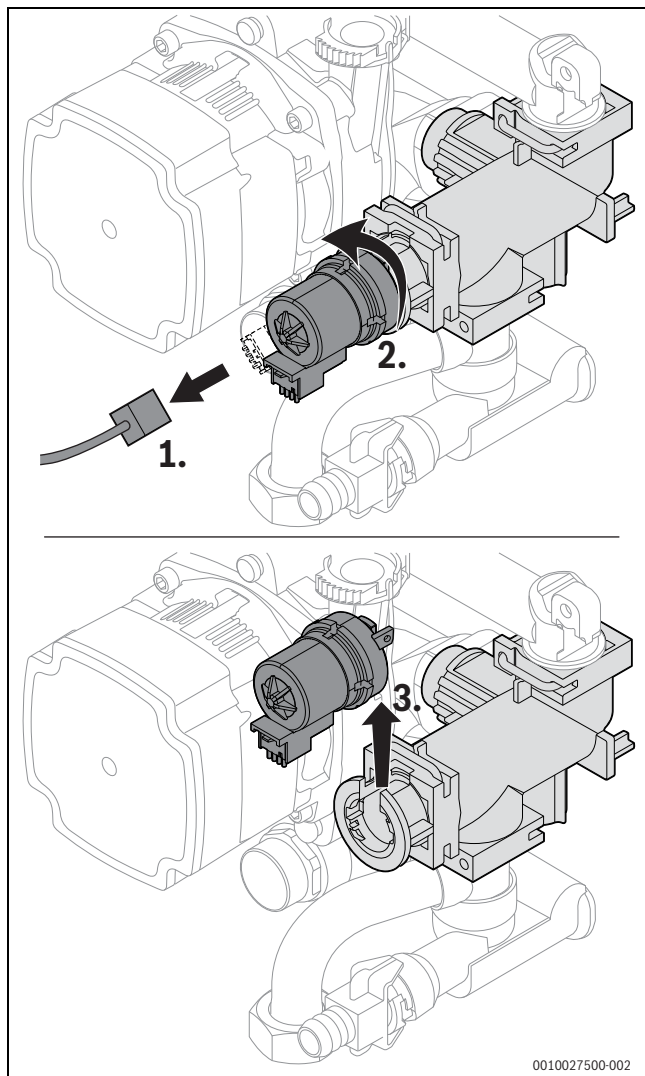
Fig. 66 Démontez le moteur au niveau de la vanne sélective (variante sans vis)
